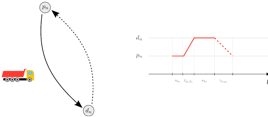
FIGURE 5.2 – Représentations d'une rotation de type \Omega_1 entre un véhicule de la catégorie f et une demande n . Sur le dessin de gauche, nous représentons une illustration du graphe. Sur le dessin de droite, nous représentons le graphique temporel de cette rotation.
