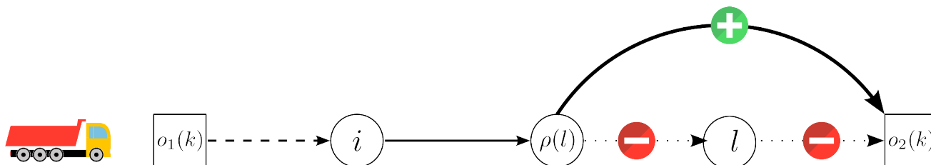
FIGURE 8.7 – Suppression d'une pause-déjeuner (C).
