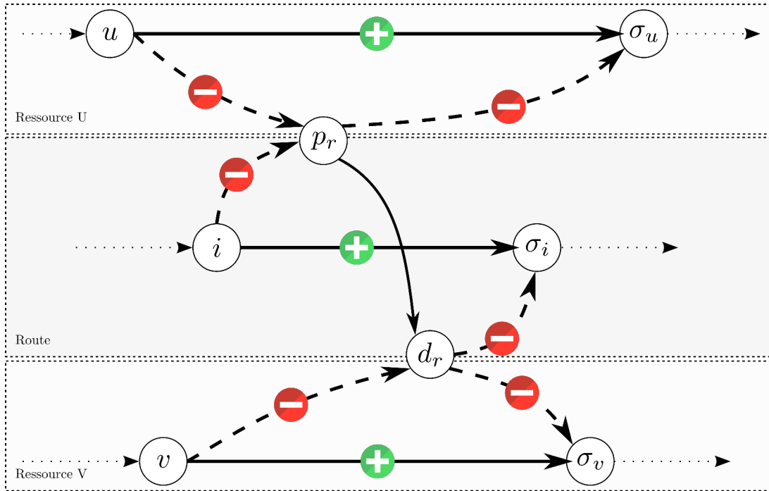
FIGURE 7.1 – Retrait d’une requête r . Les arcs retirés sont symbolisés par le symbole - et les arcs ajoutés par le symbole + .
