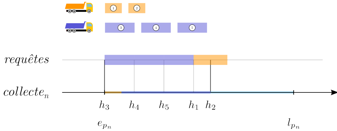
FIGURE 6.4 – Solution retenue pour la création des requêtes.
