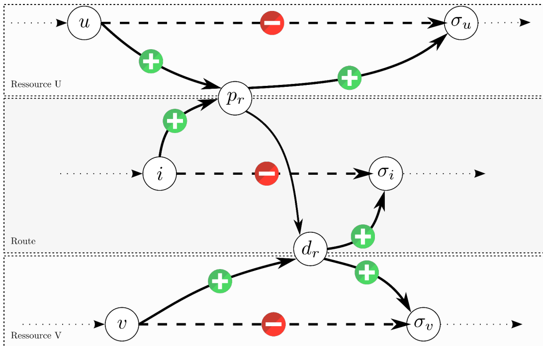
FIGURE 7.2 – Ajout d’une requête r . Les arcs retirés sont symbolisés par le symbole - et les arcs ajoutés par le symbole + .
