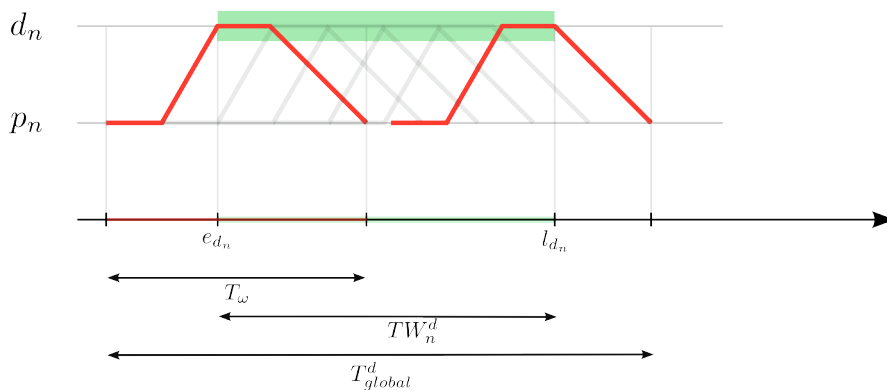
FIGURE 5.5 – Représentation du nombre d’aller-retour maximum dans le cadre d’une livraison. Dans la fenêtre de temps TW_n^d , 6 véhicules différents peuvent se succéder. Également, le premier véhicule peut effectuer la première rotation et la dernière. Son nombre maximal de rotations est de 2.
