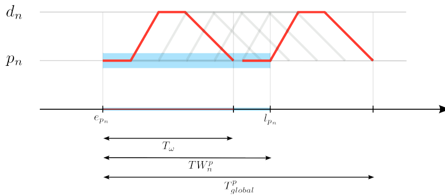
FIGURE 5.4 – Représentation du nombre d’aller-retour maximum dans le cadre d’une collecte. Dans la fenêtre de temps TW_n^p , 6 véhicules différents peuvent se succéder. Également, le premier véhicule peut effectuer la première rotation et la dernière. Son nombre maximal de rotations est de 2.
