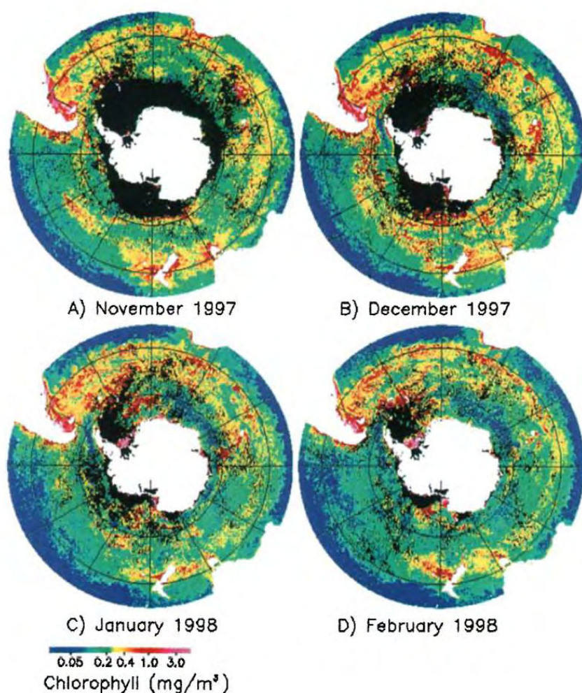
FIGURE 2.7 – Images SeaWiFS de concentration mensuelle en chlorophylle a ( \text{mg}/\text{m}^3 ) sur la période Novembre 1997 - Février 1998. Figure extraite de Moore and Abbott (2000) .
