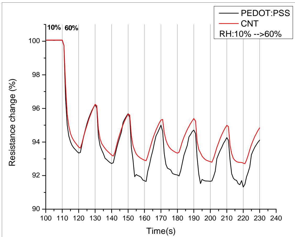
Figure IV-56.- Réponse à une variation du taux d'humidité relative de 10% à 60%.
