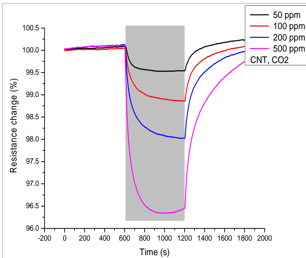
Figure IV-58.- Réponse de l'encre CNTs / PEDOT : PSS à différentes concentrations de CO 2 .
