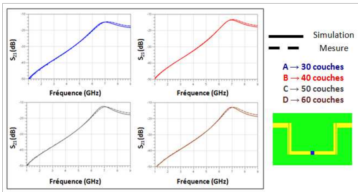
Figure III-28.- Comparaison entre la simulation et la mesure des résonateurs avec un gap rempli par un motif d'encre de CNT/polymère avec un nombre variable de couches imprimées.
