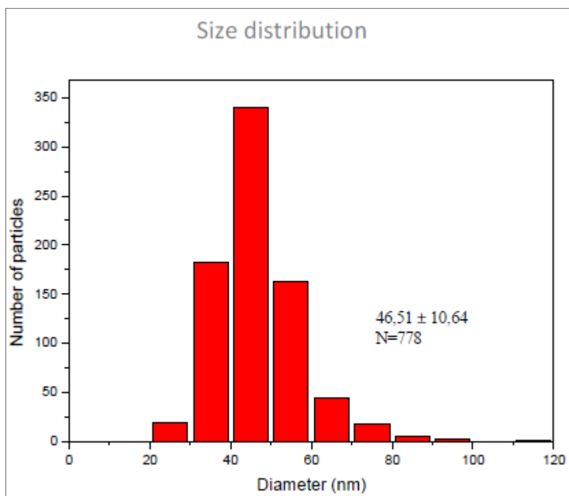
Figure II-27.- Distribution de taille des nanoparticules d'argent.
