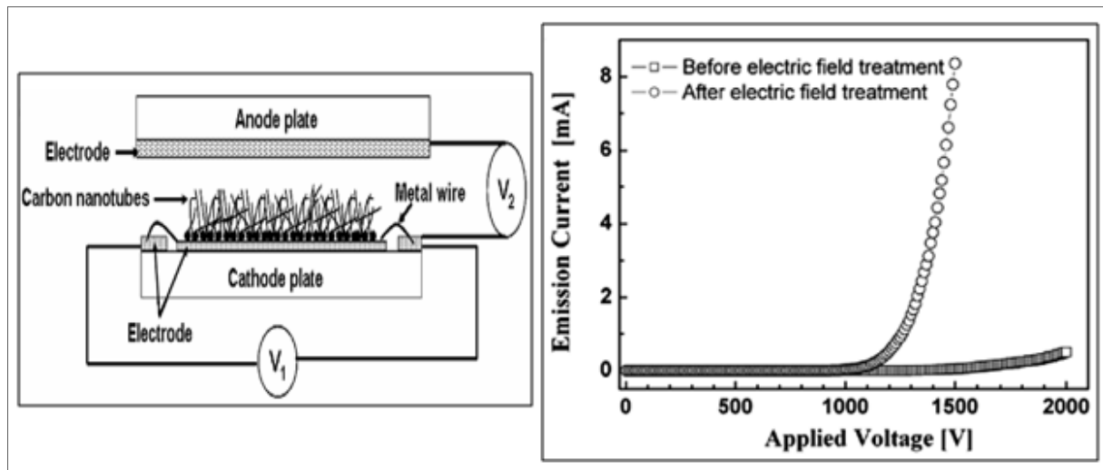
Figure I-7.- Schéma du mécanisme utilisée par Y. D. Lee et al. [I.136] pour appliquer le champ électrique aux MWCNTs (gauche). Mesures de courant et tension des MWCNTs avant et après le traitement électrique (droite).
