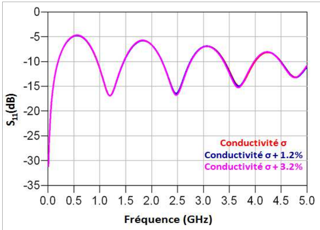
Figure IV-61.- Paramètres S_{11} des simulations de la ligne avec stub sur papier. Comparaison entre les réponses pour différentes valeurs de conductivité du motif contenant des CNTs/polymère.
