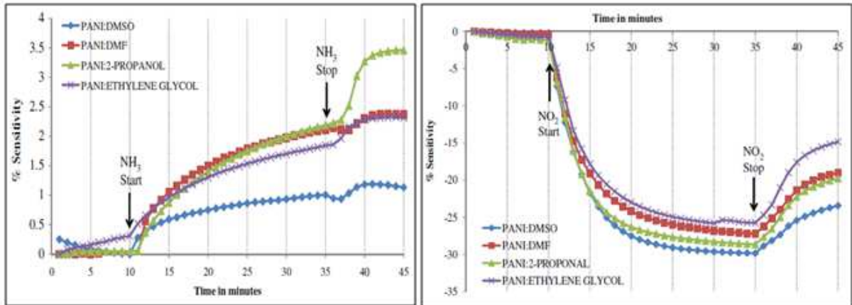
Figure IV-9.- Réponse du film de MWCNTs - PANI à 100 ppm d'ammoniac - \text{NH}_3 (gauche) et à 100 ppm de dioxyde d'azote - \text{NO}_2 (droite) avec un temps de gravure à plasma d'oxygène de 60s [IV.14].
