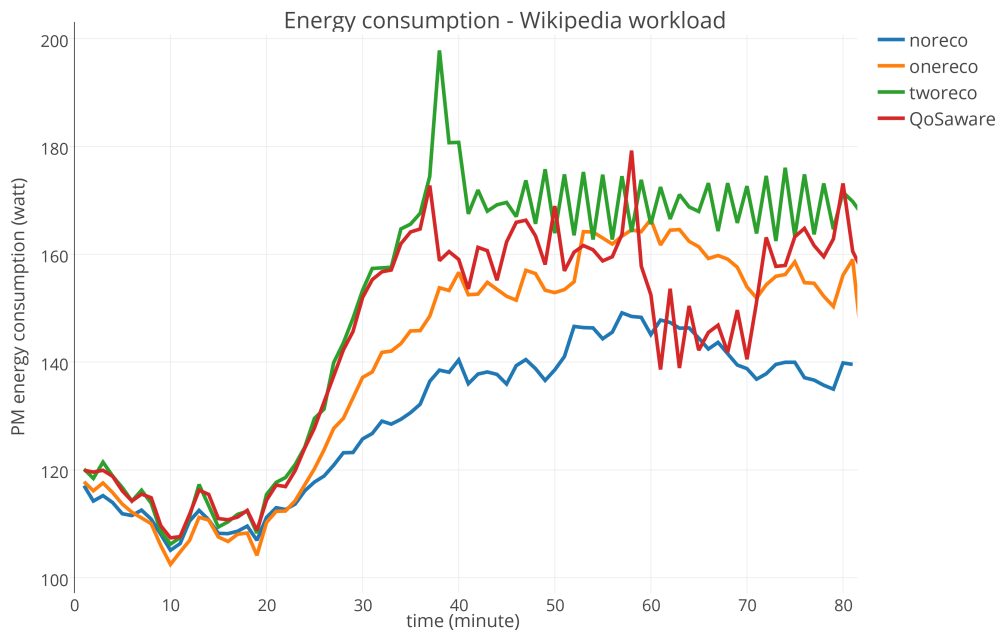
FIGURE 8.9 – Consommation énergétique - Wikipedia .
