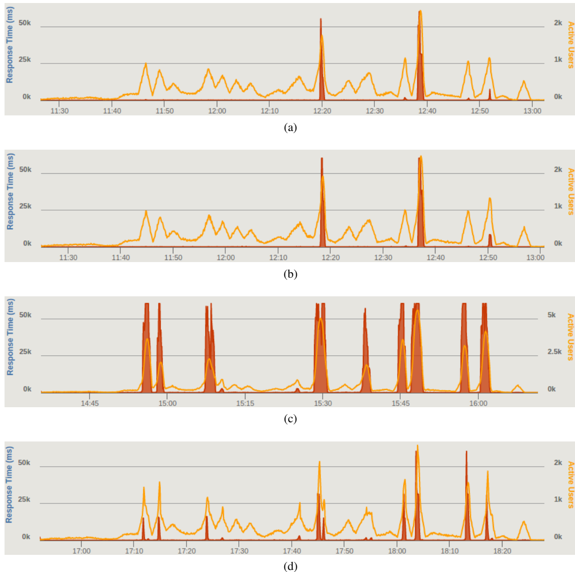
FIGURE 8.12 – Temps de réponse (requêtes OK) - FIFA.
