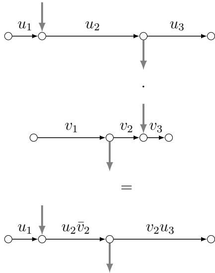
FIGURE 3.16 – Deux cas de produit non-nul d’une tuile positive (u_1, u_2, u_3) et d’une tuile négative (v_1, v_2, v_3)^{-1} : le produit peut être positif ou négatif.
