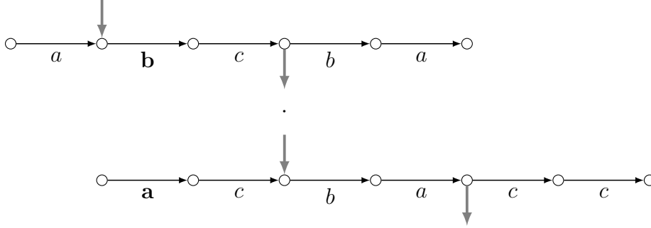
FIGURE 3.11 – En revanche, le produit des tuiles (\{1, \mathbf{b}, \mathbf{bc}, \mathbf{bcb}, \mathbf{bcba}, \bar{a}\}, ac) et (\{b, ba, bac, bacc, \bar{c}, \bar{c}\bar{a}\}, ba) vaut 0. Les arêtes en gras, étiquetées différemment, ne peuvent être unifiées, et le produit ne peut donc pas être une tuile linéaire.
