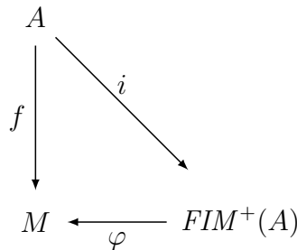
FIGURE 3.20 – Pour un alphabet A , i représentant l'injection canonique, f une application, le monoïde FIM^+(A) assure que le morphisme \varphi existe.
