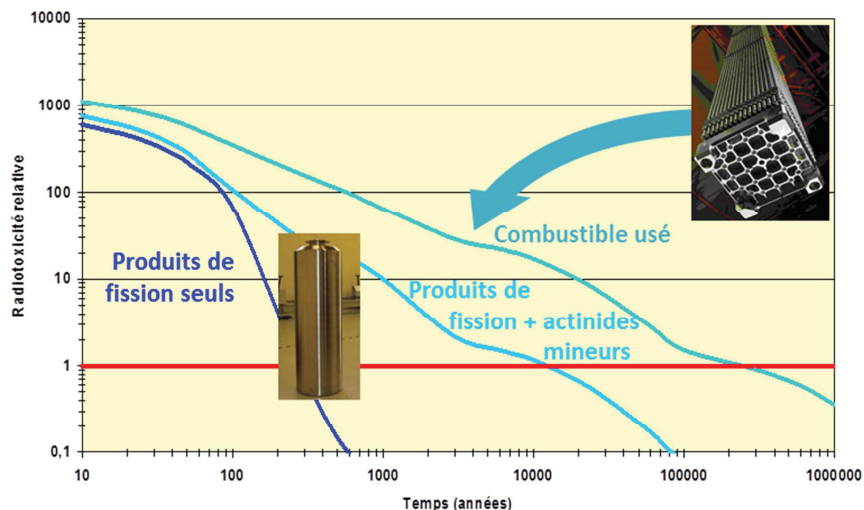
Figure 2 : Evolution de la radiotoxicité comparativement à celle des mines (ligne rouge) en fonction de la nature du déchet ultime (Combustible utilisé = UOx non retraité ; Produits de fission + actinides mineurs = Déchets vitrifiés après retraitement de l'uranium et du plutonium ; Produits de fission seuls = Déchets vitrifiés ne contenant pas d'actinides) 3
