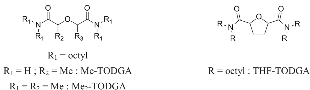
Figure 103 : Structure des nouveaux extractants étudiés par le groupe de Modolo 55,128,134
