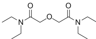
Figure 22 : Structure du TEDGA (tétraéthyl diglycolamide)
