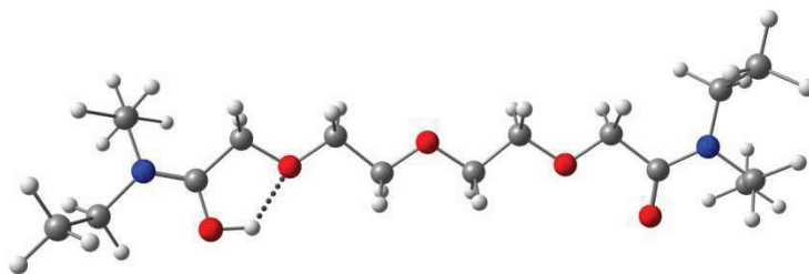
Figure 99 : Conformation la plus stable obtenue par DFT pour le TETOUDA- H^+ k
