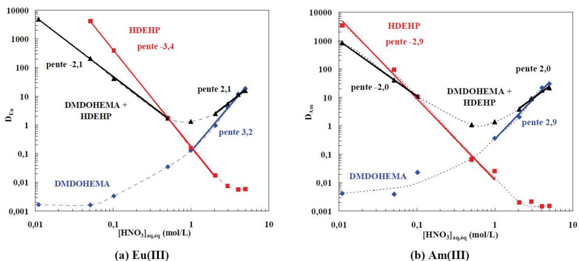
Figure 36 : Coefficients de distribution de l'euprémium et de l'américium en fonction de l'acidité en phase aqueuse à l'équilibre.
