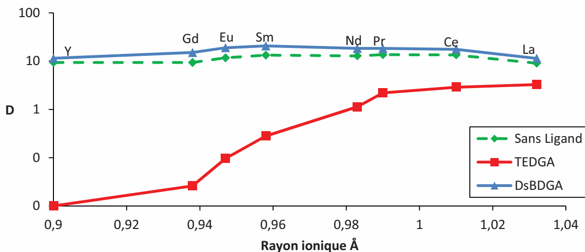
Figure 69 : Coefficients de distribution des lanthanides et de l'yttrium en fonction de leur rayon ionique Solvant : DMDOHEMA 0,6M, HDEHP 0,45M dans le TPH Phase aqueuse : HNO_3 5M ; La, Ce, Pr, Nd, Sm, Eu, Gd, Y, Mo, Zr, Fe et Pd 400mg/L ; Ligand 70mM
