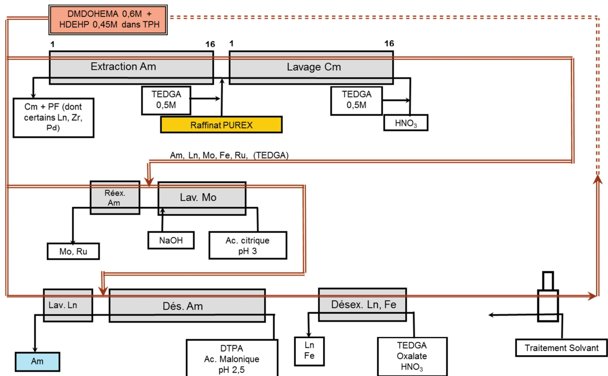
Figure 34 : Schéma du procédé EXAm testé à partir d'un raffinat PUREX 8
