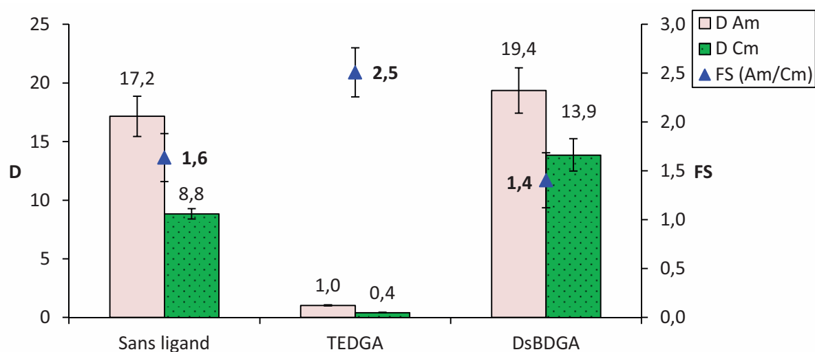
Figure 68 : Résultats d'extraction avec les DGA secondaires synthétisés Solvant : DMDOHEMA 0,6M, HDEHP 0,45M dans le TPH Phase aqueuse : HNO 3 5M ; La, Ce, Pr, Nd, Sm, Eu, Gd, Y, Mo, Zr, Fe et Pd 400mg/L ; Ligand 70mM ; tracée avec 241 Am, 244 Cm et 152 Eu
