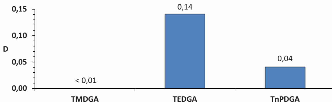
Figure 61 : Partage des ligands déterminé par HPLC Phase organique : HDEHP 0,45M, DMDOHEMA 0,6M dans du TPH Phase aqueuse : 6M HNO 3 , 30mM de ligand, 0,1mM de chaque cations (La, Nd, Sm, Eu, Y)
