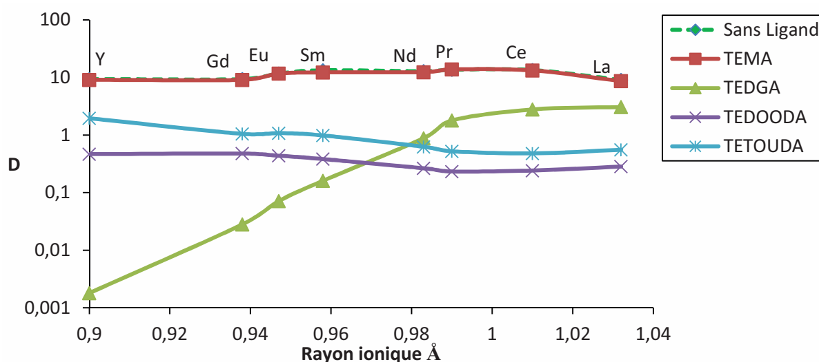
Figure 89 : Coefficients de distribution des lanthanides et de l'yttrium en fonction de leur rayon ionique Solvant : DMDOHEMA 0,6M, HDEHP 0,45M dans le TPH Phase aqueuse : \text{HNO}_3 5M ; La, Ce, Pr, Nd, Sm, Eu, Gd, Y, Mo, Zr, Fe et Pd 400mg/L ; Ligand 70mM
