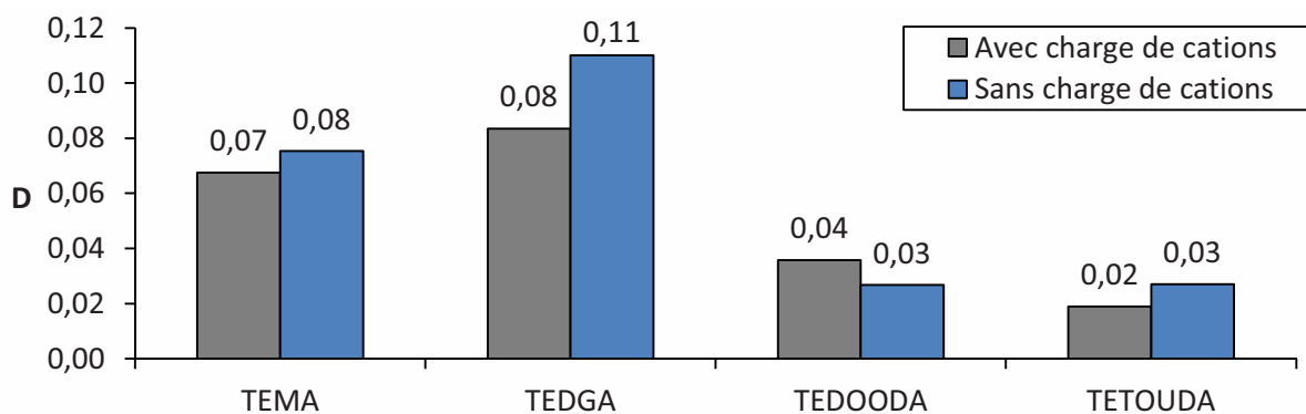
Figure 92 : Partage des ligands déterminé par HPLC Solvant : DMDOHEMA 0,6M, HDEHP 0,45M dans le TPH Phase aqueuse : HNO_3 5M ; Nd 1mM ; Ligand 70mM (bleu) Phase aqueuse : HNO_3 5M ; La, Ce, Pr, Nd, Sm, Eu, Gd, Y, Mo, Zr, Fe et Pd 400mg/L ; Ligand 70mM (gris)
