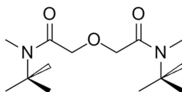
DMDtBDGA (N,N'-diméthyl-N,N'-di-ter-butyl-diglycolamide)
