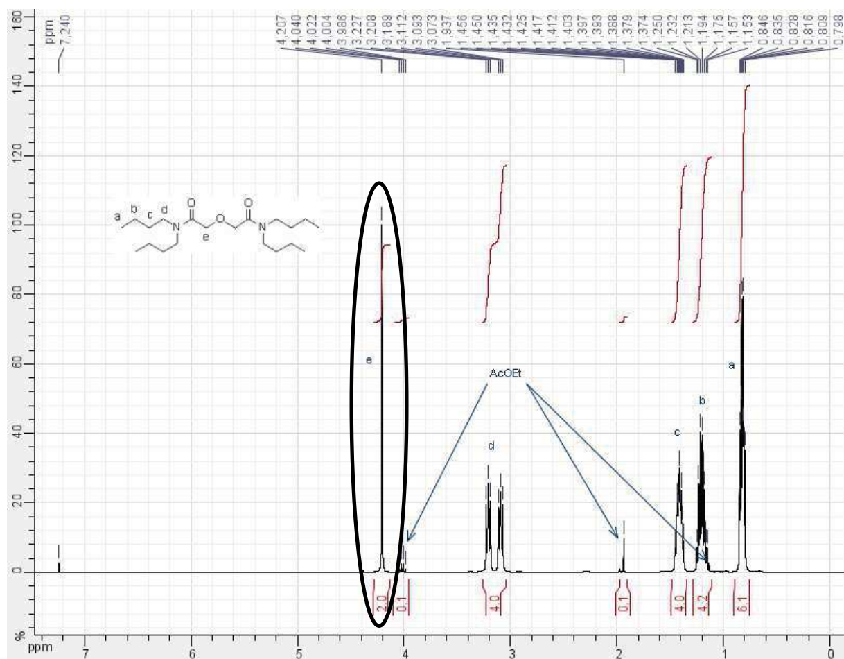
Figure 56 : Spectre RMN du TnBDGA dans le CDCl_3
