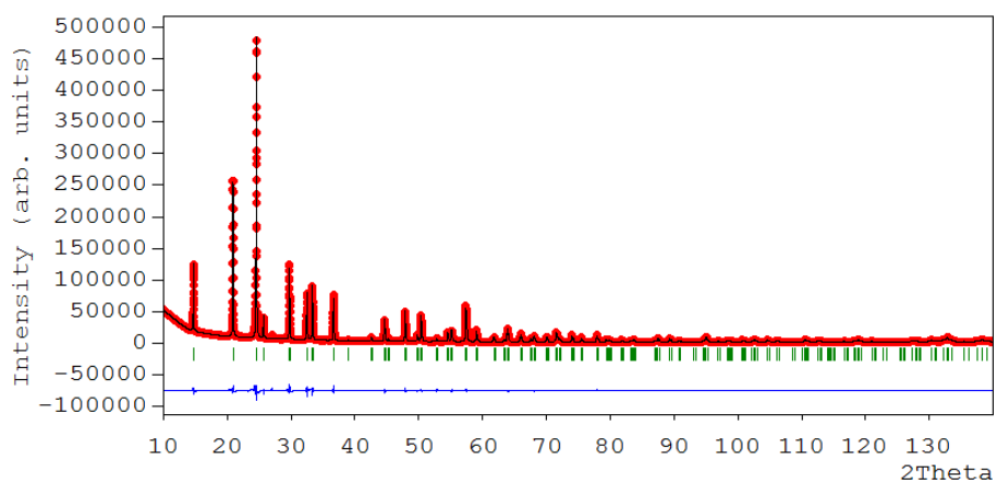
Figure III.12 : Affinement en mode Le Bail de la structure de la poudre obtenue par voie sol-gel, logiciel Fullprof. La courbe bleue montre l’écart entre le diagramme calculé et le diagramme expérimental. R_{wp} = 9,60 \% .
