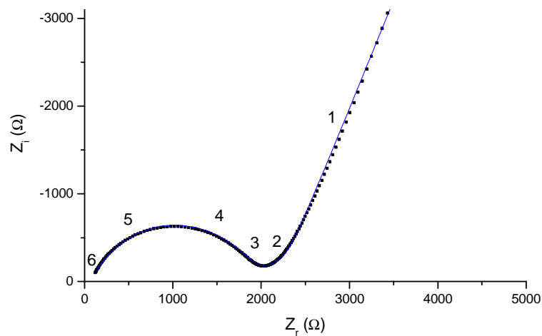
Figure II.6 : Diagramme d'impédance d'une pastille de LATP obtenue par synthèse solide-solide (densité relative 76 %). Le logarithme des fréquences de mesure a été reporté sur les diagrammes. Le modèle équivalent correspond à la courbe bleue. La pastille caractérisée mesure 12,4 mm de diamètre et 1,9 mm d'épaisseur.
