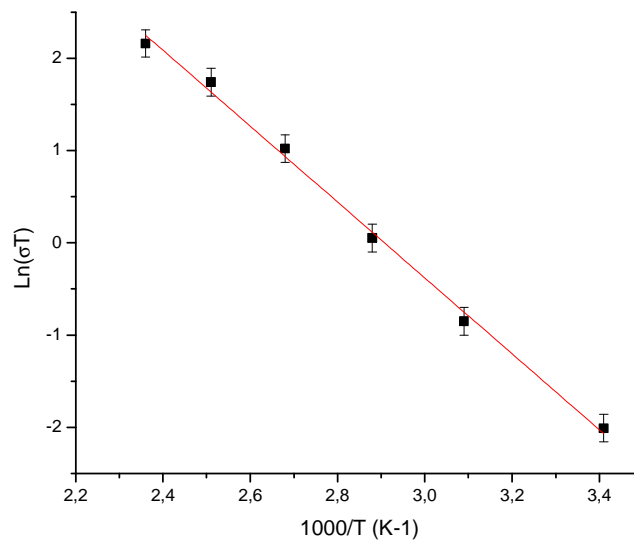
Figure III.21 : Variation de la conductivité ionique en fonction de la température obtenue sur une pastille de LATP, frittée par SPS à 900 \text{ °C} sous air pendant 1 min.
