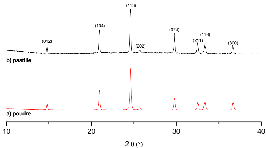
Figure II.20 : Diagrammes de diffraction des rayons X obtenus a) sur la poudre de LATP obtenue par le procédé Pechini calcinée à 900 \text{ }^\circ\text{C} pendant 4 h. b) sur la pastille polie obtenue après frittage à 950 \text{ }^\circ\text{C} pendant 6 h.
