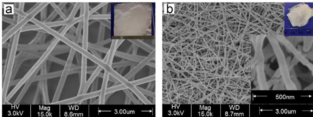
Figure I.18 : Fibres de \text{LaBO}_3 (a) Avant calcination (b) Après calcination à 750\text{ }^\circ\text{C} pendant 6h. Reproduit de 164 .
