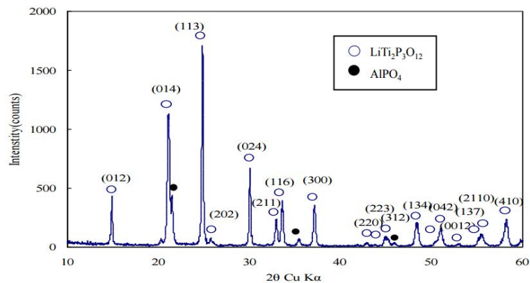
Figure I.8 : Diagramme de diffraction des rayons X de la vitrocéramique Ohara Corporation. Reproduite de 116
