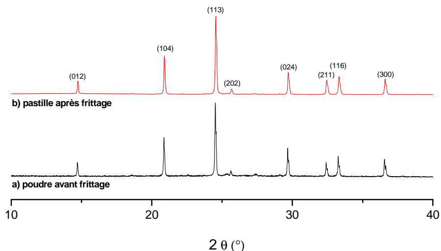
Figure II.29 : Diagrammes de diffraction des rayons X. a) Poudre avant frittage. b) Pastille après frittage ( 950 \text{ }^\circ\text{C} , 6 h).
