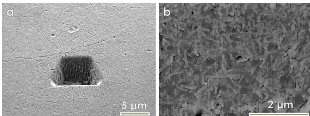
Figure III.45 : Vues en coupe d'une membrane contenant 66 % volumiques de PVDF-HFP, réalisées par sonde ionique focalisée. a) vue d'ensemble de l'échantillon, face S. b) vue en coupe de la membrane.
