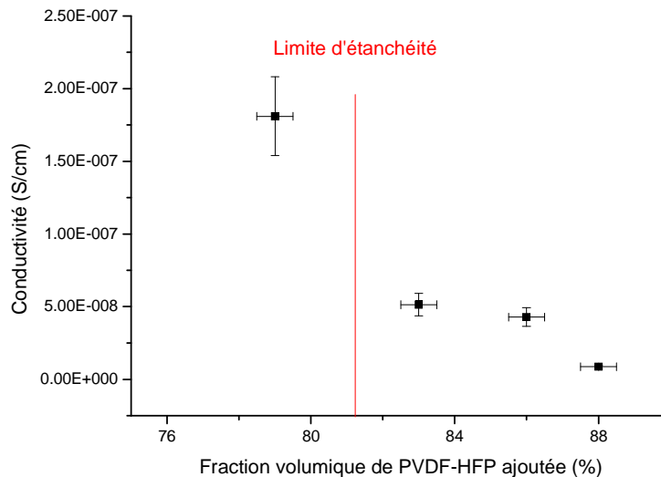
Figure III.57 : Evolution de la conductivité et de l'étanchéité des membranes en fonction de la fraction volumique de PVDF-HFP ajoutée.
