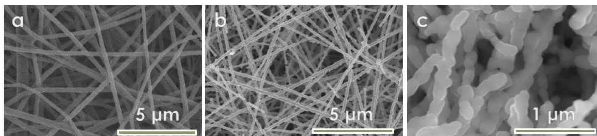
Figure III.34 : Images obtenues par microscopie électronique à balayage à effet de champ. a) fibres après électrospinning, grossissement x10000. b) fibres calcinées à 850 °C pendant 2 h, avec une rampe de 5 °C.min -1 , grossissement x10000. c) fibres calcinées dans les mêmes conditions, grossissement x50000.
