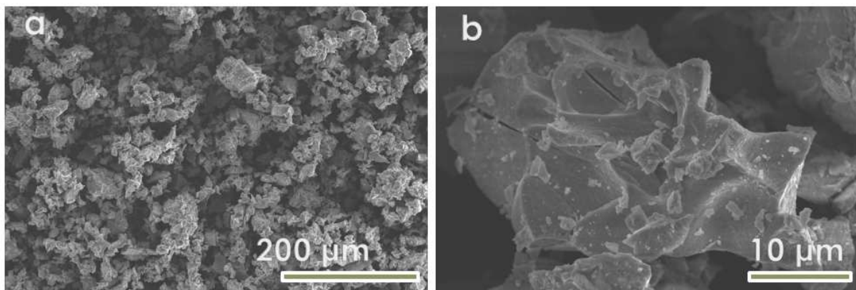
Figure A3.2: Morphologie des particules de LLTO, microscope à balayage. a) grandissement x200. b) grandissement x3000.
