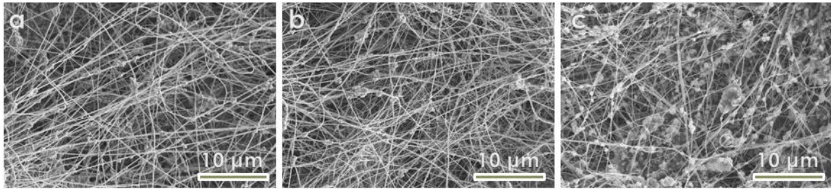
Figure II.45 : Effet de la fraction volumique de LATP sur la microstructure des membranes. a) 40 %. b) 60 %. c) 80 %.
