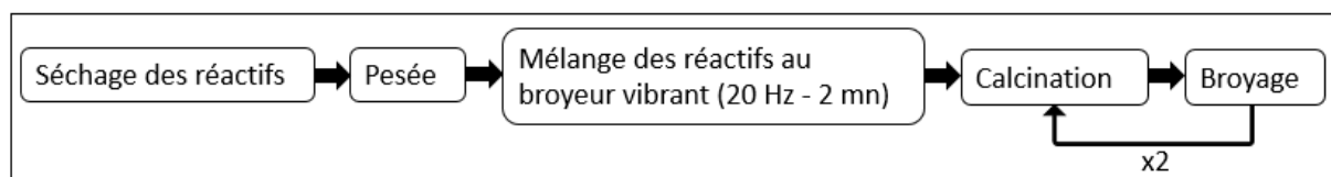
Figure II.1 : Mode opératoire de la synthèse solide-solide.
