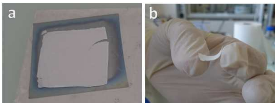
Figure III.33 : a) morphologie du dépôt après calcination à 850 °C pendant 2 h avec une rampe de 5 °C.min -1 . Le volume injecté est de 1 mL. b) flexibilité d'un réseau de nanofibres de 50 μm d'épaisseur.
