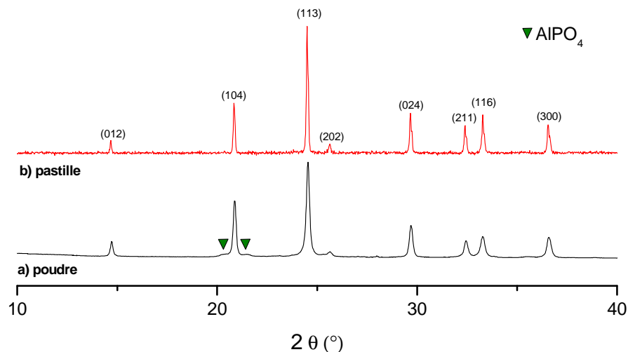
Figure II.13 : Diagrammes de diffraction des rayons X obtenus a) sur la poudre de LATP obtenue par coprécipitation et calcinée à 750 \text{ }^\circ\text{C} pendant 2 h 30. b) sur la pastille polie obtenue après frittage ( 950 \text{ }^\circ\text{C} pendant 6 h).
