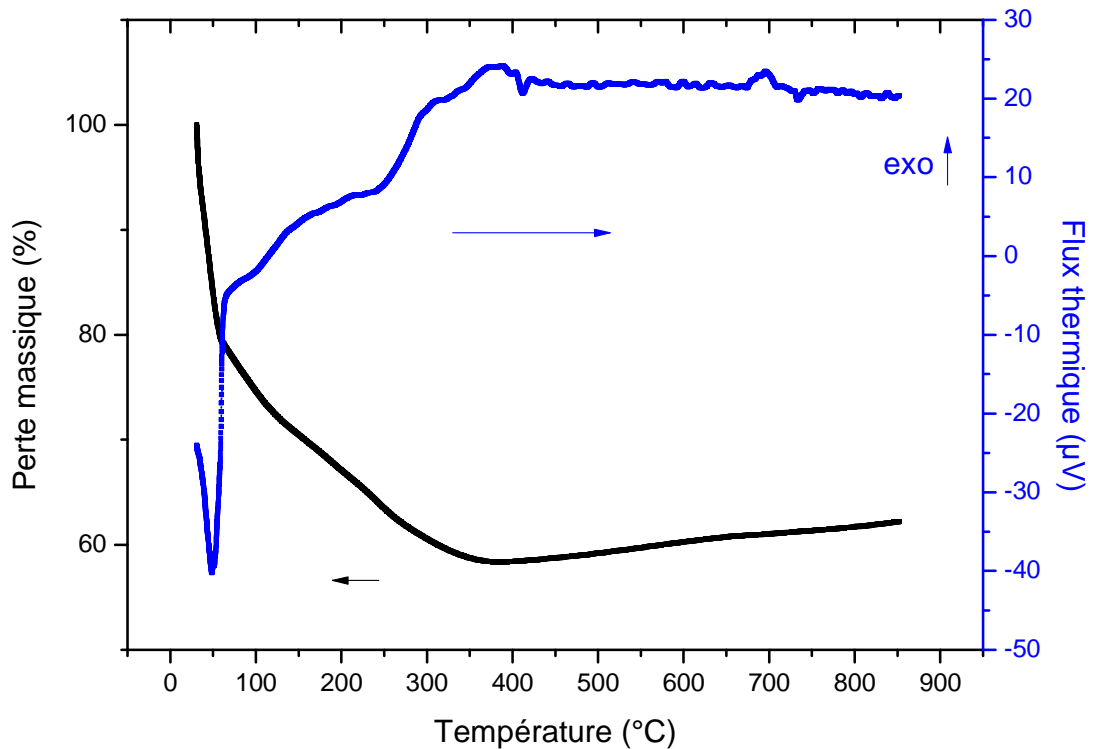
Figure II.8 : Analyse thermique du précurseur coprécipité. En bleu, l'analyse thermique différentielle. En noir, la thermogravimétrie.
