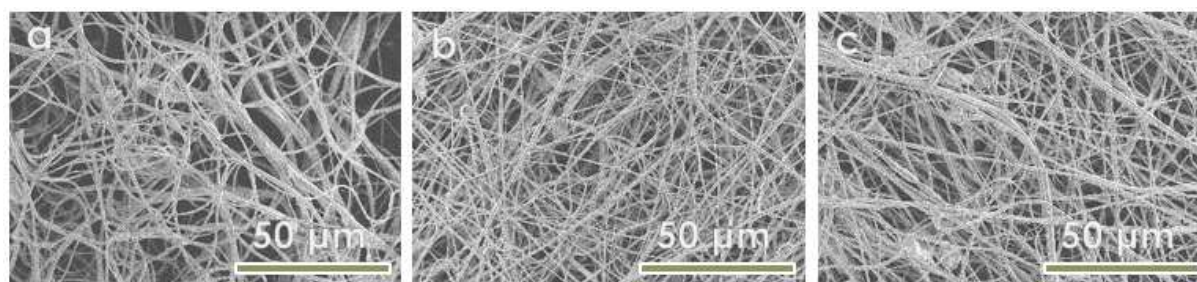
Figure A3.4 : Effet des paramètres procédé sur l'homogénéité du dépôt, microscope à balayage. a) 10 cm, 24 kV, 100\text{ }\mu\text{L}\cdot\text{min}^{-1} . b) 10 cm, 12 kV, 20\text{ }\mu\text{L}\cdot\text{min}^{-1} . c) 10 cm, 14 kV, 30\text{ }\mu\text{L}\cdot\text{min}^{-1} .
