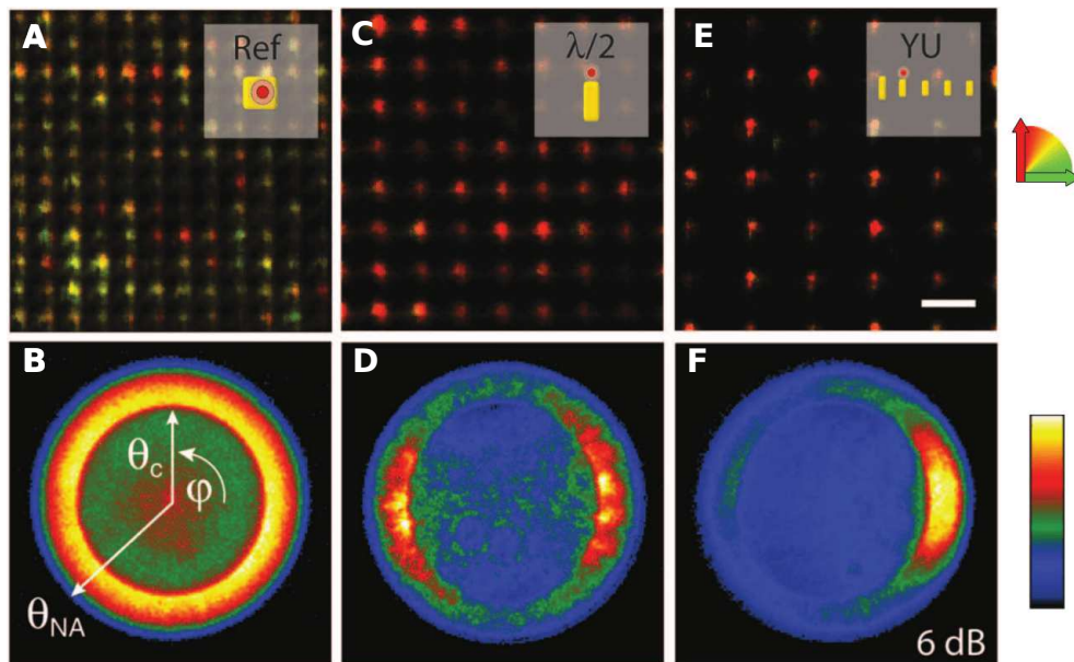
FIGURE 3.10 – Colonne de gauche : Boîtes quantiques déposées sur des carrés d'or Colonne du centre : Boîtes quantiques couplées à une antenne \lambda/2 en or. Colonne de droite : Boîtes quantiques couplées à une antenne Yagi-Uda en or. La polarisation du rayonnement est représentée selon l'échelle à droite de la figure : les flèches verticale et horizontale indiquent l'orientation de la polarisation. D'après [180]
