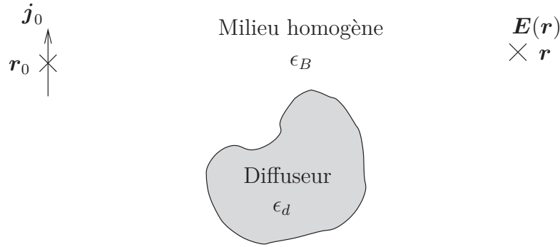
FIGURE C.1 – Représentation de la source en \mathbf{r}_0 , du diffuseur dans un fond homogène, et d'un point arbitraire où le champ \mathbf{E}(\mathbf{r}) est calculé.
