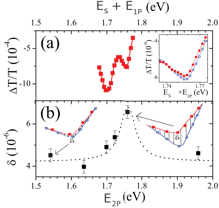
FIGURE 2.26 – (a) Signal non-linéaire en fonction de la somme des énergies E_s + E_{1p} . L’encart représente un zoom sur la partie biexcitonique du signal, où est ajouté le signal du biexciton en présence des deux pompes (cercles bleus). (b) Déformation \delta du spectre de transmission différentielle du biexciton en présence de la seconde pompe en fonction de son énergie E_{2p} . Les deux schémas sont des illustrations de la signification de \delta . La ligne pointillée est un guide Lorentzien pour les yeux.
