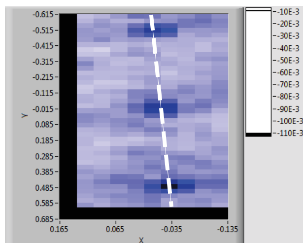
FIGURE 3.33 – Carte de réflectivité de trois antennes alignées verticalement. La ligne pointillée blanche est un guide pour l'œil et passe par le centre des antennes. Une dérive mécanique de 100 nm par heure est observée.
