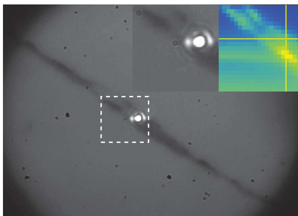
FIGURE 3.31 – Corrélation entre l'imagerie en lampe blanche (à gauche) et la carte de PL (à droite) d'une ligne de gélatine contenant des nanotube de carbone déposés sur un substrat de verre. L'échelle spatiale est respectée entre la carte de PL et l'imagerie. L'échelle d'intensité de la carte de PL est arbitraire. Le point blanc sur l'image en lampe blanche est le spot laser, dont la position équivalente est repérée sur la carte de PL par la croix jaune.
