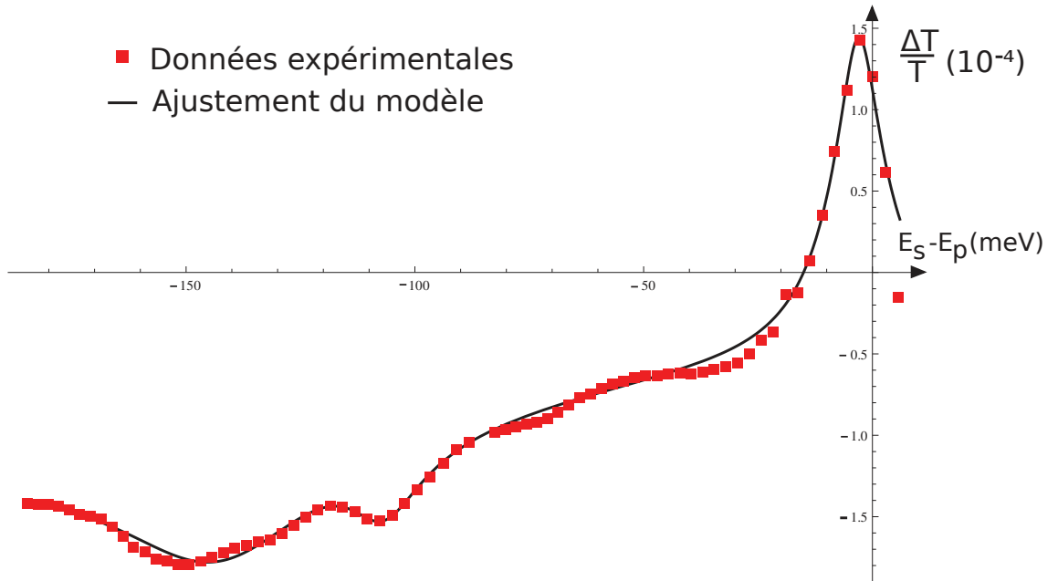
FIGURE 2.36 – Signal non-linéaire expérimental (carrés rouges) en fonction du désaccord entre l'énergie de sonde et l'énergie de pompe, ajusté par le modèle (trait plein).
