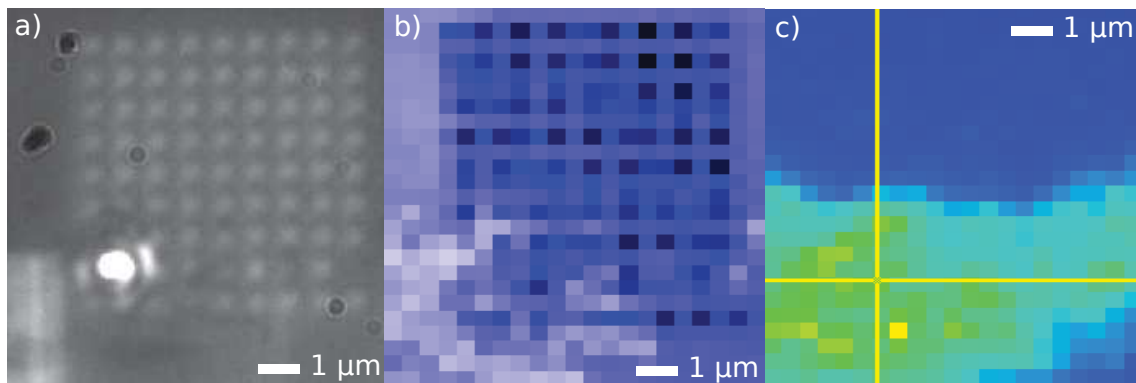
FIGURE 3.32 – Corrélation entre l'imagerie en lampe blanche a), la carte de réflectivité b) et la carte de PL c) d'un réseau d'antenne sur lequel sont dispersés des nanotubes de carbones en gélatine. Le point blanc sur l'image en lampe blanche est le spot laser, dont la position équivalente est repérée sur la carte de PL par la croix jaune.
