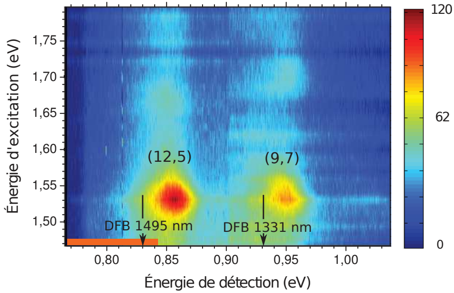
FIGURE 2.9 – Carte 2D de photoluminescence d'excitation à une température de 10 K de la distribution de nanotubes. Les deux flèches indiquent les énergies de pompage. Le trait épais horizontal sur l'axe des abscisses indique la partie haute énergie du domaine sondable, qui recouvre l'énergie du DFB 1495 nm. Le photoblanchiment de l'exciton est observé en pompant la classe (12,5) tandis que les grands désaccords sont étudiés en pompant la classe (9,7).
