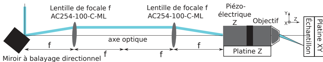
FIGURE 3.29 – Schéma du dispositif de déplacement du point de focalisation sur l'échantillon.
