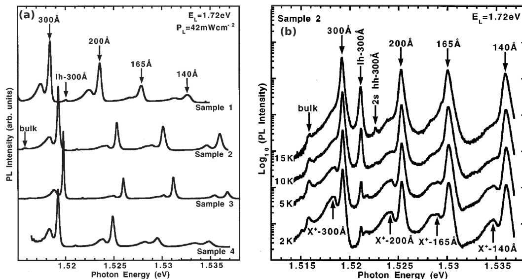
FIGURE 1.30 – (a) Photoluminescence de quatre échantillons de quatre puits quantiques GaAs/Al 0.66 Ga 0.33 As. (b) Etude en température du signal de photoluminescence de l'échantillon numéro 2. D'après [106].
