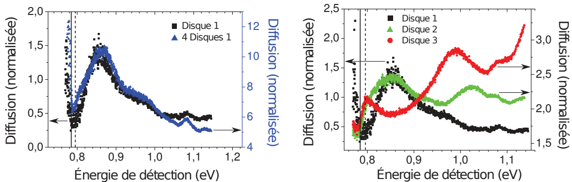
FIGURE 3.27 – (a) Spectre de diffusion en champ sombre d'un disque et de quatre disques de 300 nm de rayon. (b) Spectre de diffusion en champ sombre d'antennes disques de trois diamètres différents.
