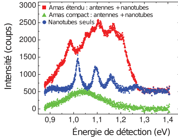
FIGURE 3.46 – Comparaison des spectres de nanotubes de type C associées à des antennes commerciales avec le spectre des nanotubes sans antennes. Les spectres sont décalés en intensité pour plus de clarté.
