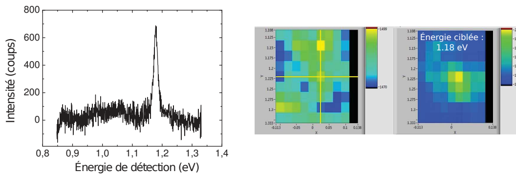
FIGURE 3.39 – Cartes et spectre de photoluminescence d'un échantillon de type B sur lequel on observe l'émission d'un nanotube unique.
