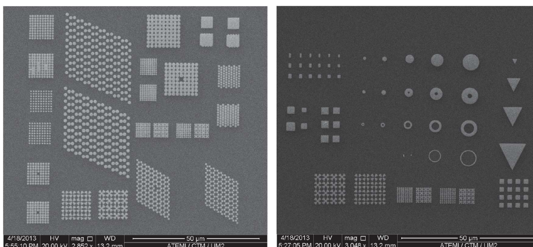
FIGURE 3.18 – Réseau d’antennes métalliques.
