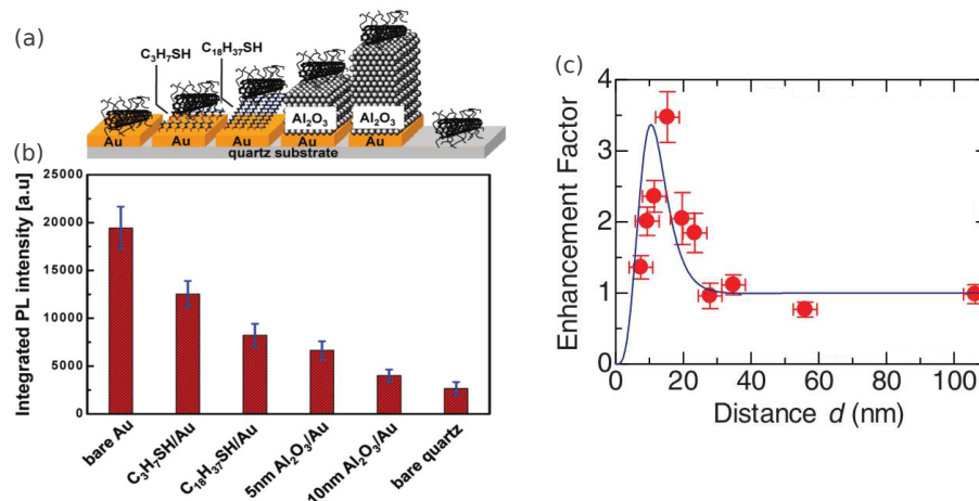
FIGURE 3.16 – Illustration des différentes configurations conduisant à des espacements de plus en plus importants entre le nanotube et le plan d’or rugueux (a), et intensité intégrée de la luminescence des tubes dans chacune de ces configurations (b), d’après [207]. Dépendance expérimentale (rond) et théorique (trait plein) de l’exaltation de la luminescence du nanotube en fonction de la distance entre le nanotube et la surface rugueuse, d’après [206].
