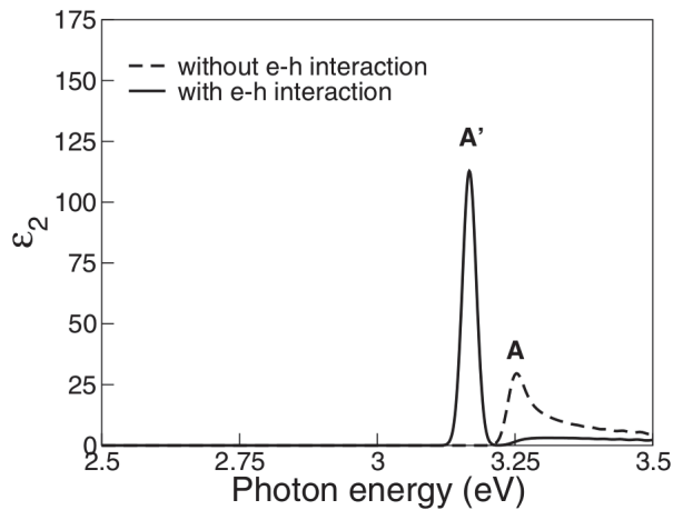
FIGURE 1.14 – Spectre d'absorption théorique d'un nanotube. Le pic A' est d'origine excitonique, tandis que le pic A provient des paires e-h libres. D'après [40].
