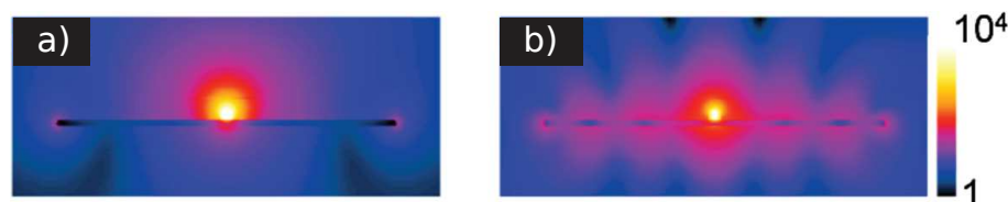
FIGURE 3.14 – Simulation de l'amplitude du champ électrique dans un plan passant par l'axe d'un disque d'argent de rayon 600 nm, excité par un dipôle aux longueurs d'onde \lambda_0 : 1763 nm (a) et 760 nm (b). D'après [198]
