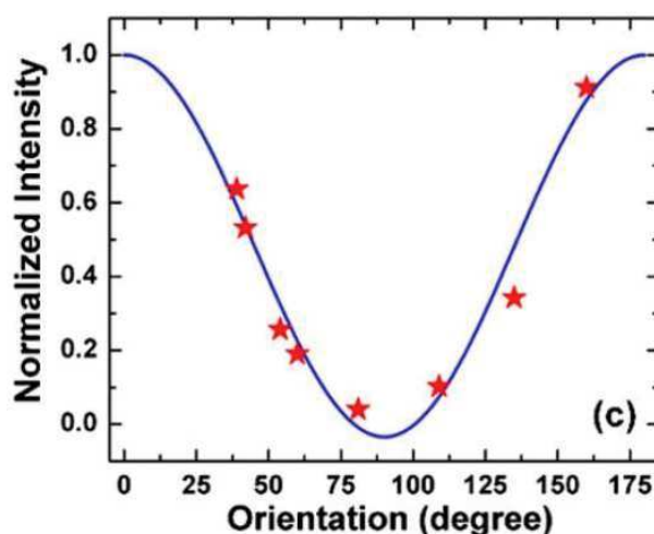
FIGURE 3.17 – Intensité de photoluminescence (étoiles rouges) en fonction de l’orientation du nanotube par rapport à la direction de propagation de l’onde de surface excitateur. La ligne bleu est un ajustement par une fonction \cos^2(\theta_{NT}) où \theta_{NT} est l’angle en abscisse de cette figure. D’après [164]
