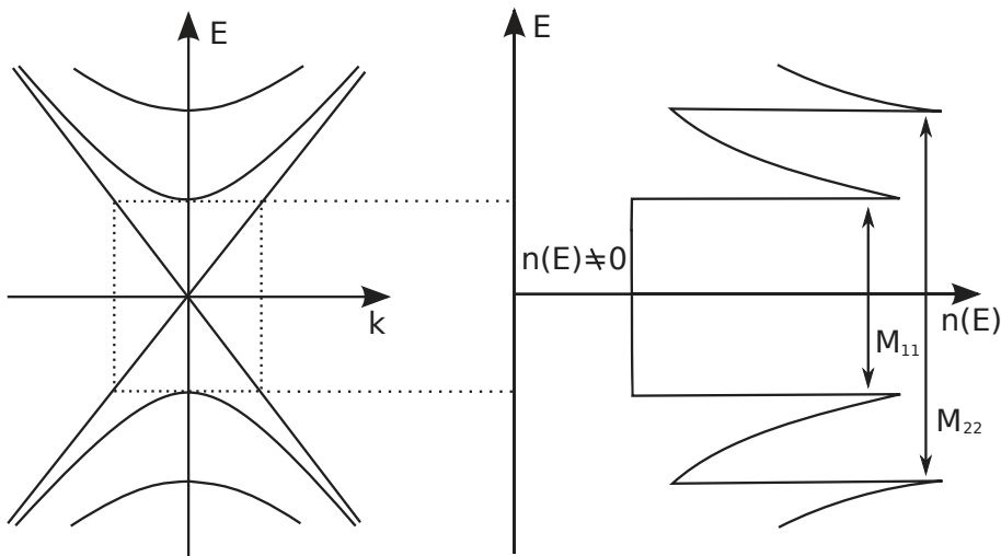
FIGURE 1.8 – Représentation de la densité d'états électroniques n(E) d'un nanotube métallique
