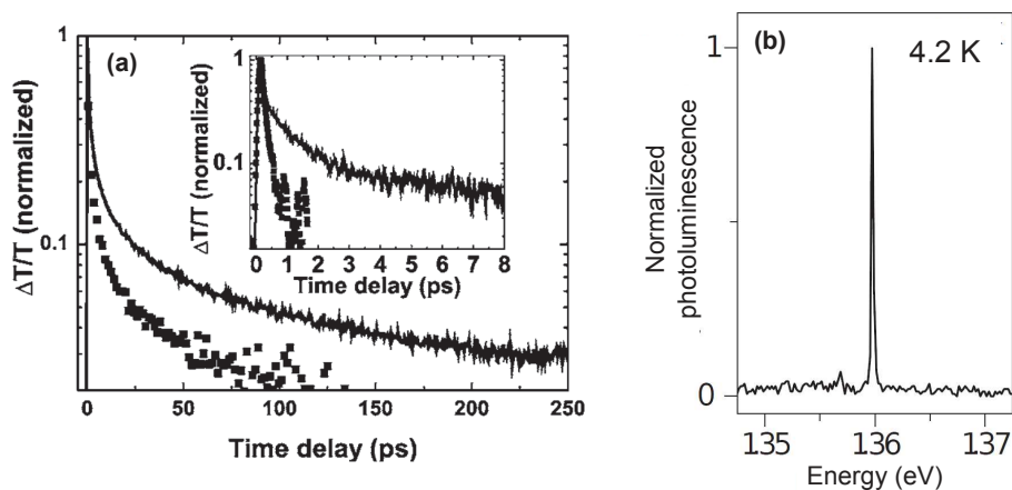
FIGURE 1.23 – (a) Signal pompe-sonde résolu en temps de nanotubes agrégés (carrés pleins) et de nanotubes isolés en micelles (trait plein). D'après [81] (b) Photoluminescence de nanotube suspendu dans l'air. D'après [82].
