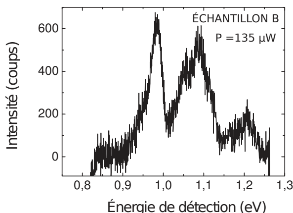
FIGURE 3.38 – Spectres de photoluminescence d'un échantillon de type B dense en nanotubes, excité à une énergie de 1.96 eV (633 nm).
