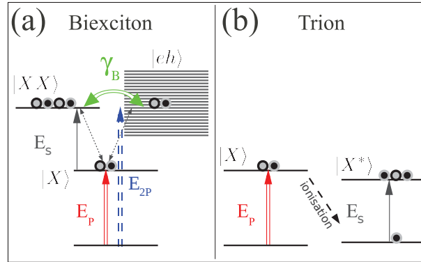
FIGURE 2.21 – (a) Processus de formation du biexciton |XX\rangle et de ses interactions avec le continuum |eh\rangle des paires e-h libres. \gamma_B est le taux d'annihilation du biexciton caractérisant le couplage de type Coulombien entre le biexciton et le continuum des paires e-h libres. (b) Processus de formation du trion |X^*\rangle .
