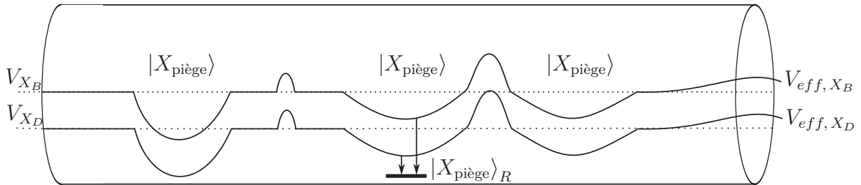
FIGURE 1.22 – Représentation du potentiel effectif V_{eff} formant pour les états électroniques des pièges |X_{piège}\rangle . Est représenté un état |X_{piège}\rangle_R optiquement actifs, induit par un défaut, vers lequel les excitons peuvent se désexciter.
