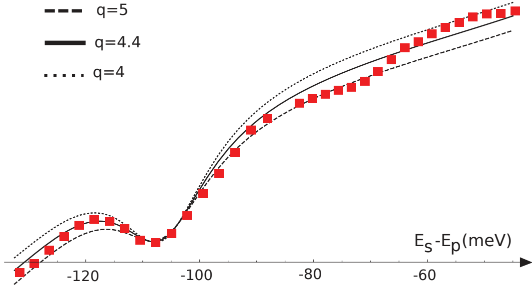
FIGURE 2.39 – Zoom sur la raie du biexciton du modèle complet, ajustant les données brutes pour différentes valeurs de q dans le régime \hbar\Gamma_{X,XX} \approx \hbar\eta .
