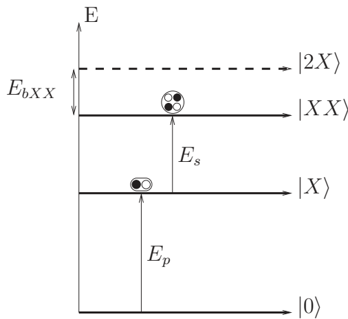
FIGURE 2.6 – Représentation des états à un exciton |X\rangle , deux excitons |2X\rangle et celui du biexciton |XX\rangle .
