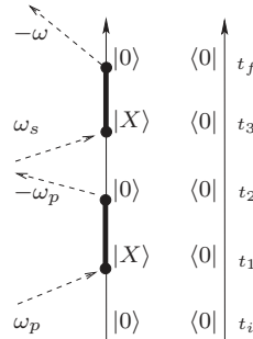
FIGURE 2.28 – Diagramme participant à la susceptibilité du troisième ordre.
