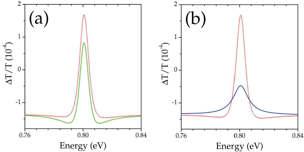
FIGURE 2.3 – Contributions \Delta\Gamma (a) et \Delta f (b) dans le signal non linéaire excitonique. D'après [133]
