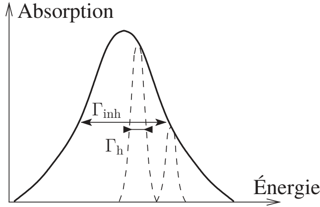
FIGURE 2.1 – Absorption linéaire d'un ensemble de systèmes à deux niveaux présentant un élargissement inhomogène \Gamma_{inh} . Des Lorentziennes de largeur \Gamma_h ont été ajoutées pour illustrer la réponse homogène de deux systèmes à deux niveaux particuliers.
