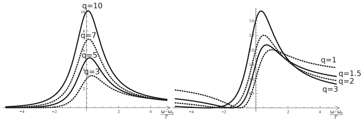
FIGURE 2.33 – Comportement de la fonction F(\omega) pour différentes valeur du facteur de Fano q .
