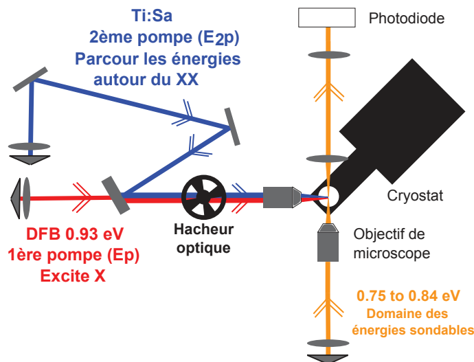
FIGURE 2.22 – Schéma de la configuration à deux pompes.
