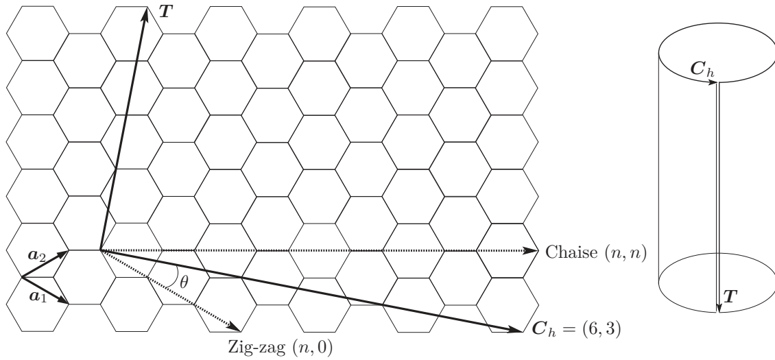
FIGURE 1.1 – Construction géométrique du nanotube (6,3) par enroulement d'une feuille de graphène le long du vecteur chiral \mathbf{C}_h et autour du vecteur de translation \mathbf{T}
