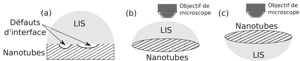
FIGURE 3.36 – Différentes configurations testées avec la LIS.
