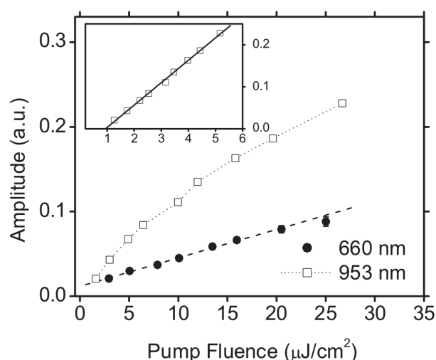
FIGURE 1.28 – Évolution de l'amplitude maximale du signal pompe-sonde de la chiralité de nanotube (8,3) en fonction de la puissance du laser de pompe. L'encart présente une partie des données (carrés ouverts) de la figure principale, tracées en fonction de la racine carrée de la puissance de pompe. D'après [99]
