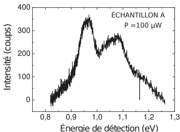
FIGURE 3.34 – Spectres de photoluminescence d'un échantillon de type A dense en nanotubes, excité à une énergie de 1.96 eV (633 nm).
