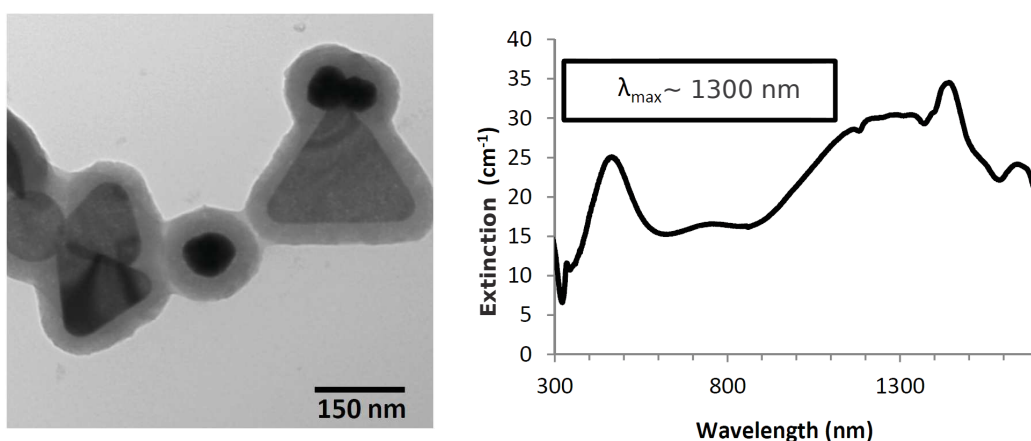
FIGURE 3.19 – Imagerie des antennes commerciales et caractérisation de leur absorption. D’après nanoComposix.
