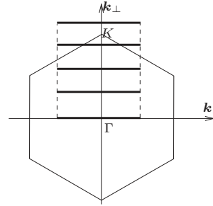
FIGURE 1.5 – Première zone de Brillouin d'un nanotube semi-conducteur superposé à celle du graphène. Chaque segment épais correspond à une valeur de \mu .
