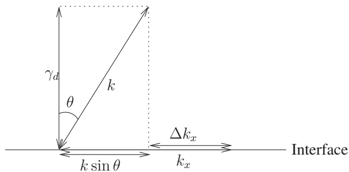
FIGURE 3.8 – Schéma de l'émission d'un photon par diffusion d'une onde de surface sur un défaut topologique.
