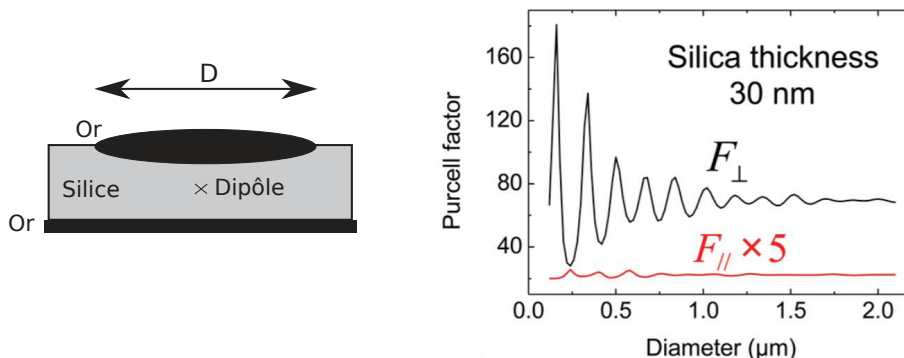
FIGURE 3.13 – Illustration d'une antenne patch . Évolution théorique du facteur de Purcell d'un dipôle couplé à une antenne patch , en fonction du diamètre D , d'après [197]
