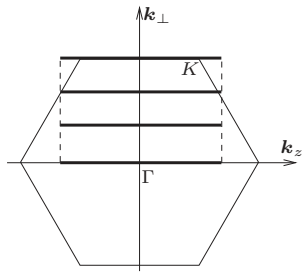
FIGURE 1.4 – Première zone de Brillouin d'un nanotube métallique superposé à celle du graphène. Chaque segment épais correspond à une valeur de \mu .
