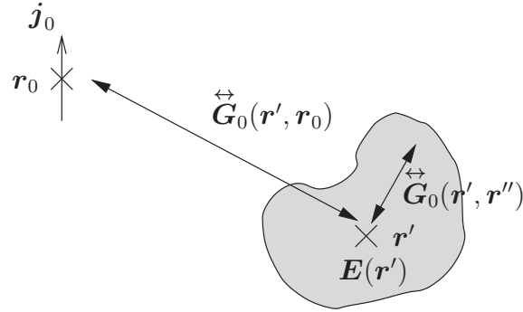
FIGURE C.3 – Représentation de la contribution au champ \mathbf{E}(\mathbf{r}') de la source en \mathbf{r}_0 et d'un point \mathbf{r}'' du diffuseur. La contribution totale du diffuseur est obtenue par intégration sur le volume du diffuseur de la contribution ponctuelle \overleftrightarrow{\mathbf{G}}_0(\mathbf{r}', \mathbf{r}'')\mathbf{j}_{\text{ind}}(\mathbf{r}'') .
