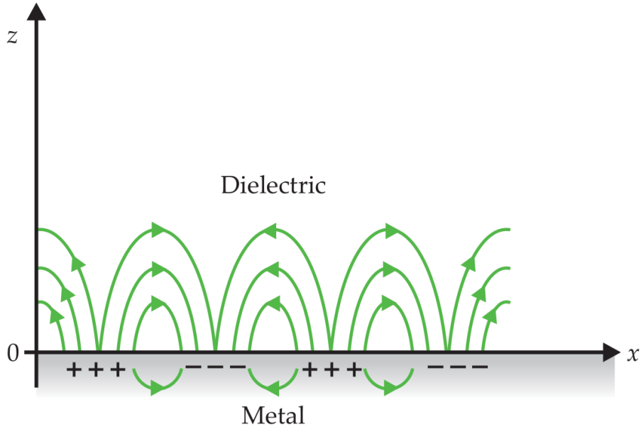
FIGURE 3.6 – Représentation du champ électrique d'une onde de surface. D'après [170]
