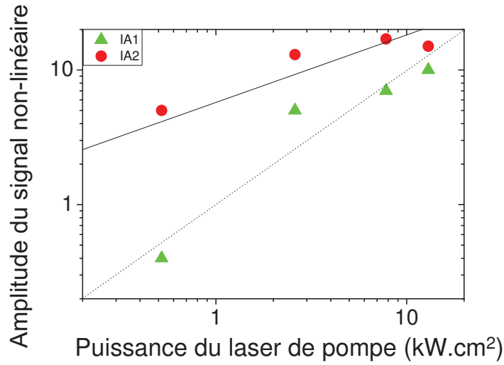
FIGURE 2.20 – Dépendance de l'amplitude maximale de transmission différentielle normalisée des effets d'absorptions induites IA_1 à E_s - E_p = -150 meV et IA_2 à E_s - E_p = -105 meV, en fonction de la puissance d'excitation par unité de surface.
