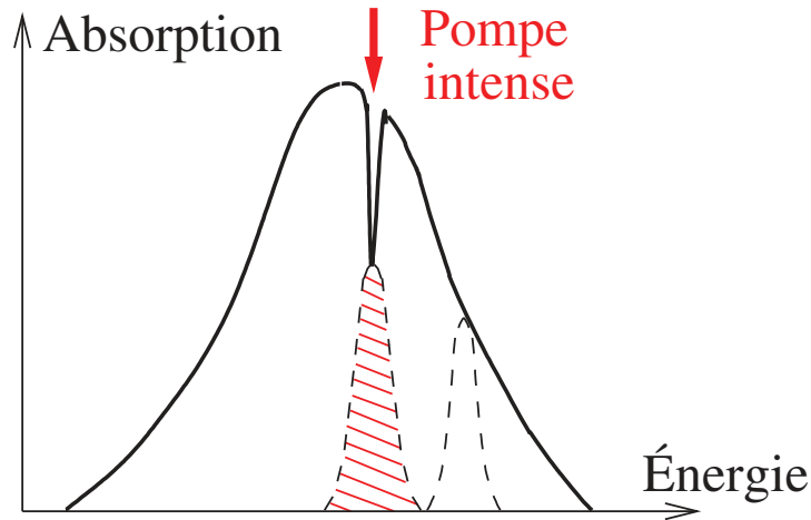
FIGURE 2.2 – Illustration de l'absorption d'un ensemble de systèmes à deux niveaux dont l'absorption d'un sous-ensemble (représentée par la lorentzienne hachurée de largeur arbitraire) est saturée par un laser de pompe intense. Dans le spectre d'absorption d'ensemble, on observe un trou centré sur l'énergie du laser de pompe.
