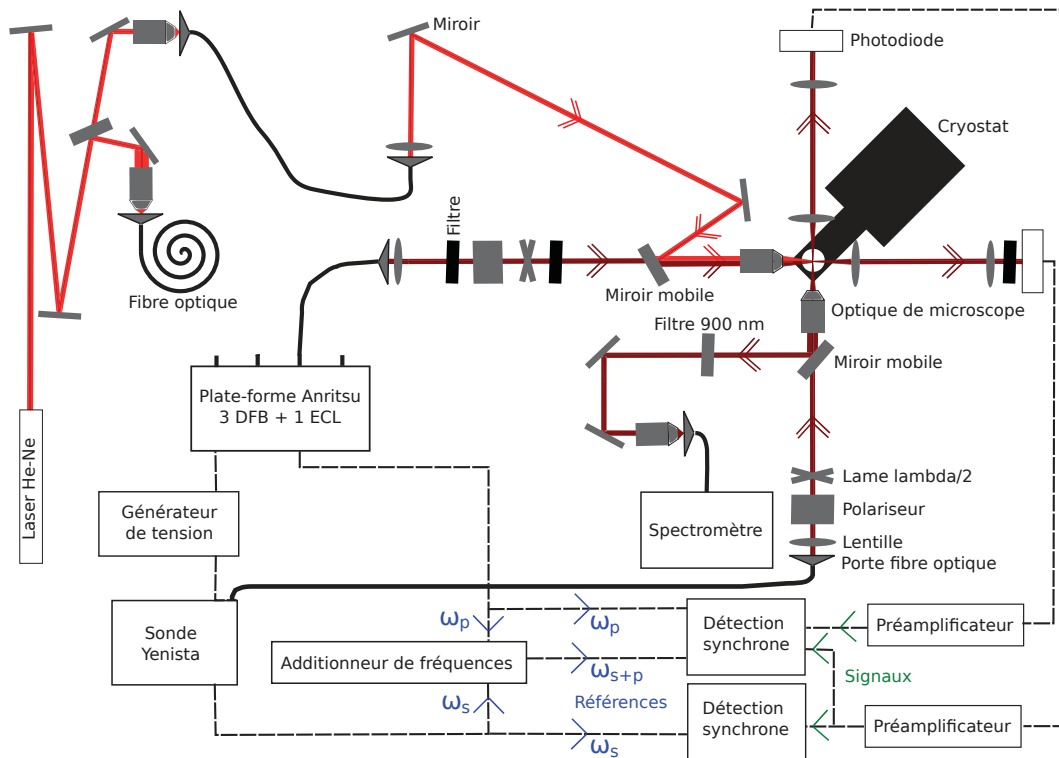
FIGURE 2.8 – Schéma du dispositif expérimental.
