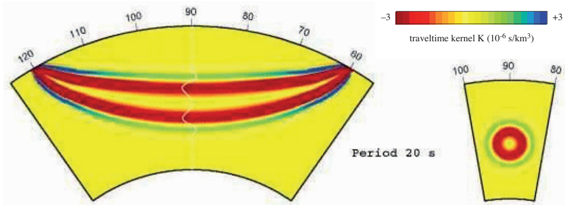
FIGURE 2.1 – Noyau de sensibilité des perturbation de temps d'arrivées d'ondes P \delta T à des variations de vitesses \delta v pour une distance épicentrale \Delta = 60^\circ sur une section de la Terre (gauche) et sur une coupe transversale (droite), d'après [Hung et al., 2000].
