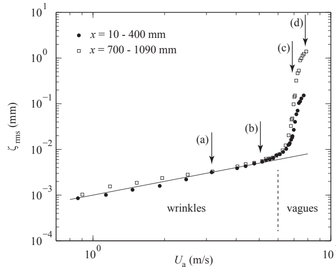
Figure B.3: Amplitude moyenne des déformations \zeta_{\text{rms}} en fonction de la vitesse du vent U_a . Les données sont moyennées sur la fenêtre de visualisation 390 \times 280 \text{ mm} centré à deux valeurs de fetch x = 205 \text{ mm} ( \bullet ) et x = 895 \text{ mm} ( \square ). Les lettres et les flèches verticales correspondent aux quatre champs de hauteur instantanés de la figure B.2. La ligne continue correspond à l'approximation linéaire \zeta_{\text{rms}} = \alpha U_a , avec \alpha = 10^{-6} \text{ s} .
