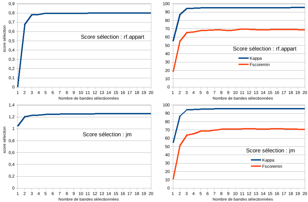
FIGURE 6.4 – Jeu de données Pavia : influence du nombre de bandes sélectionnées sur le score utilisé pour la sélection d’attributs (à gauche) et sur la qualité de la classification par un classifieur SVM gaussien en utilisant les jeux de bandes sélectionnés (à droite, avec en bleu le coefficient Kappa (en %) et en rouge le F-score (en %) le plus faible). Les 2 scores de sélection d’attributs considérés sont rf.appart (ligne du haut) et jm (ligne du bas)
