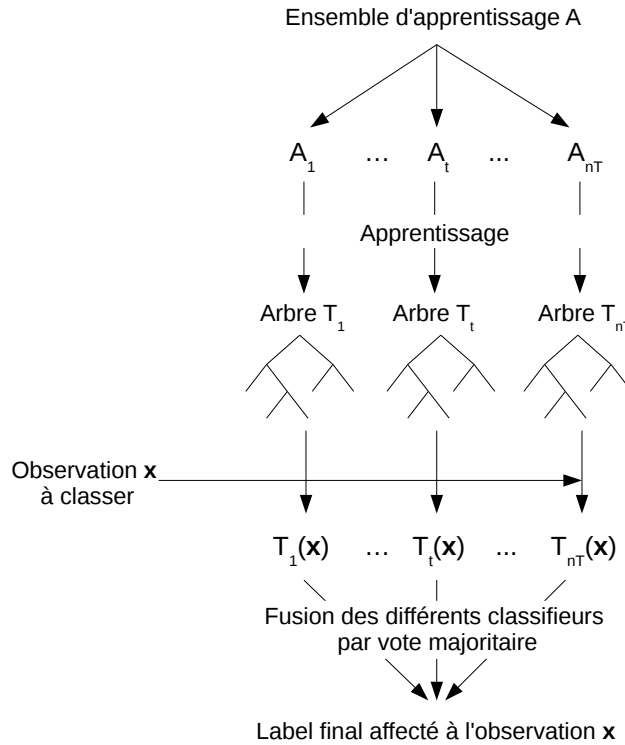
FIGURE 3.2 – Principe des forêts aléatoires (apprentissage et classification)
