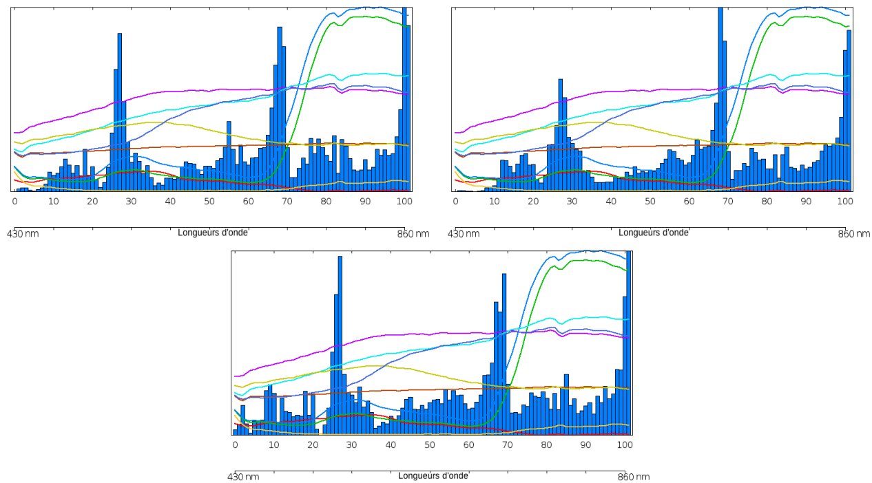
FIGURE 6.9 – Pavia : profils d'importance de bandes obtenus pour différents critères de sélection d'attributs : rf.appart (en haut à gauche), rf.conf (en haut à droite), rf.K (en bas)
