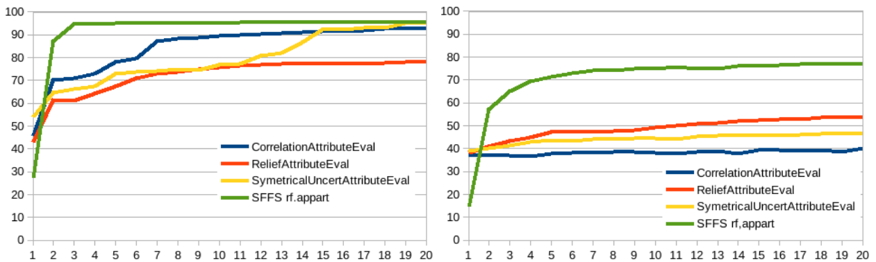
FIGURE 6.16 – Evolution (pour Pavie à gauche et Indian Pines à droite) du Kappa obtenu pour un classifieur SVM à noyau gaussien en fonction du nombre de bandes sélectionnées, pour des sélections de bandes effectuées à partir des 3 scores CorrelationAttributeEval , ReliefAttributeEval et SymmetricalUncertAttributeEval et par la méthode SFFS pour le score rf.appart
