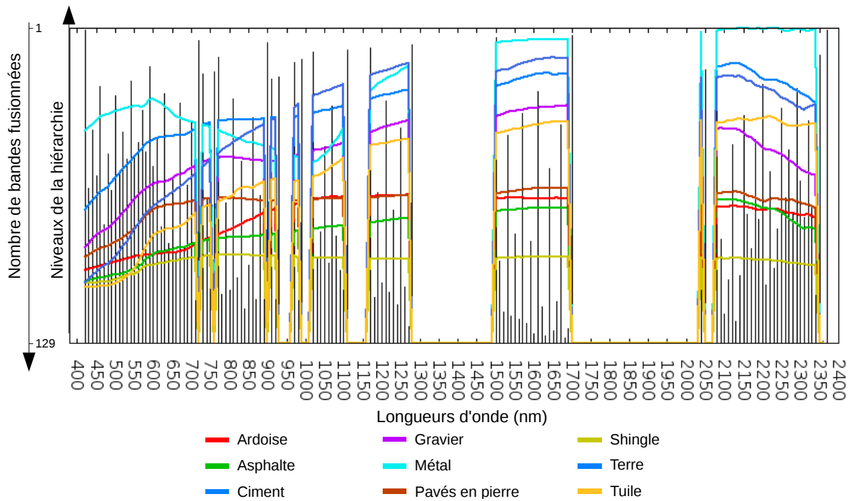
FIGURE 9.11 – Légende 1 : hiérarchie de bandes fusionnées obtenue pour le critère de fusion “erreur de reconstruction du spectre” L’abscisse correspond aux numéros/longueur d’onde des bandes. L’axe des ordonnées correspond aux niveaux dans la hiérarchie de bandes fusionnées (en bas : niveau le plus fin avec les bandes originales, en haut : une bande fusionnée unique). Les lignes noires verticales sont les limites entre bandes fusionnées : plus on monte dans la hiérarchie, plus le nombre de bandes fusionnées diminue. Les spectres médians des classes en présence sont affichés en couleur.
