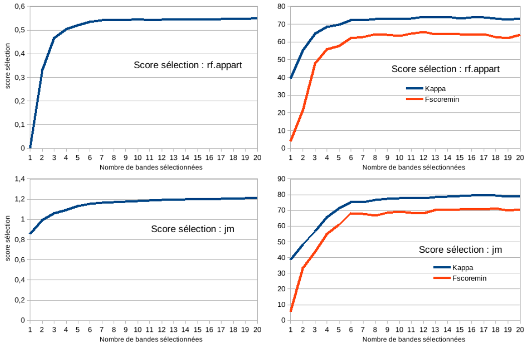
FIGURE 6.5 – Jeu de données Indian Pines : influence du nombre de bandes sélectionnées sur le score utilisé pour la sélection d’attributs (à gauche) et sur la qualité de la classification par un classifieur SVM gaussien en utilisant les jeux de bandes sélectionnées (à droite, avec en bleu le coefficient Kappa (en %) et en rouge le F-score (en %) le plus faible). Les 2 scores de sélection d’attributs considérés sont rf.appart (ligne du haut) et jm (ligne du bas)
