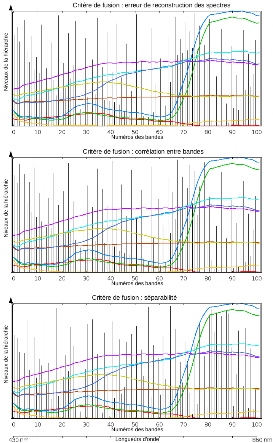
FIGURE 7.4 – Hiérarchies de bandes fusionnées obtenues pour différents critères sur le jeu de données Pavie : “erreur de reconstruction du spectre” (en haut), “corrélation entre bandes” (au milieu), “séparabilité” (en bas). L’abscisse correspond aux numéros/longueur d’onde des bandes. L’axe des ordonnées correspond aux niveaux dans la hiérarchie de bandes fusionnées (en bas : niveau le plus fin avec les bandes originales, en haut : une bande fusionnée unique). Les lignes noires verticales sont les limites entre bandes fusionnées : plus on monte dans la hiérarchie, plus le nombre de bandes fusionnées diminue. Les spectres médians des classes en présence sont affichés en couleur.
