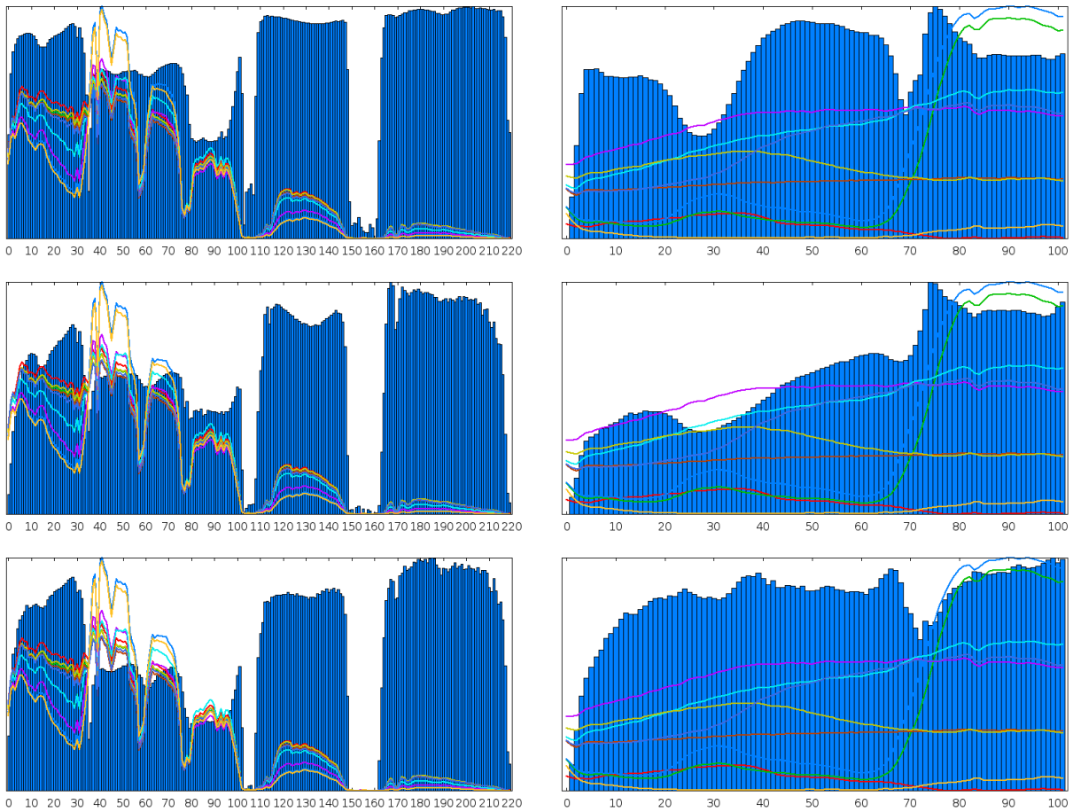
FIGURE 6.15 – Exemples pour Pavie (à gauche) et Indian Pines (à droite) d’importances de bandes données par différentes mesures de type filtre, avec de haut en bas, la corrélation entre les attributs et les classes, la mesure fournie par ReliefF et l’incertitude symétrique par rapport à une classe
