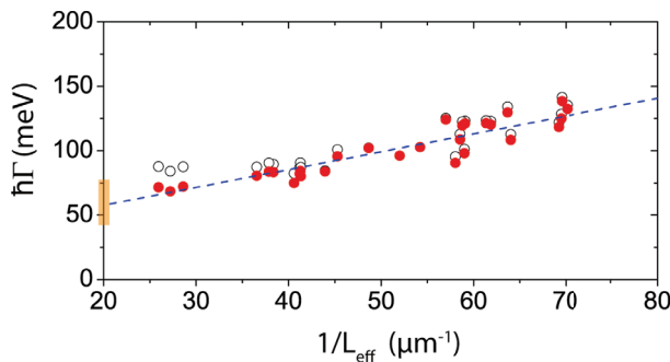
FIGURE 3.2 – Largeurs spectrales \Gamma de résonance plasmon de nanobâtonnets Au@SiO_2 en fonction de la longueur effective L_{eff} = \sqrt{LD} . Les points (○) sont les données brutes, les points (●) sont les données après soustraction du terme radiatif ( \Gamma - \Gamma_r ). La droite tiretée est un ajustement par une droite affine, on obtient g_s = 0,7 \pm 0,1 [55].
