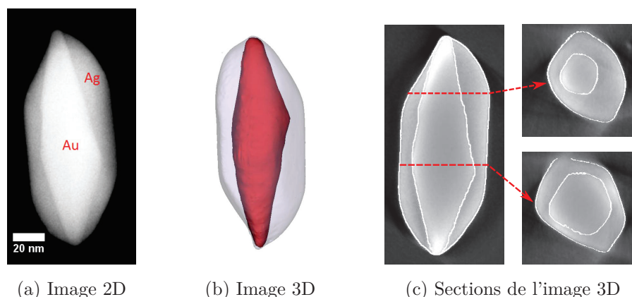
FIGURE 2.18 – Tomographie électronique d’une bipyramide d’or entourée d’argent. (a) Image 2D réalisée par MEET en mode HAADF. (b) Reconstruction 3D de la bipyramide. (c) Sections selon l’axe de la bipyramide et perpendiculaire à celui-ci.
