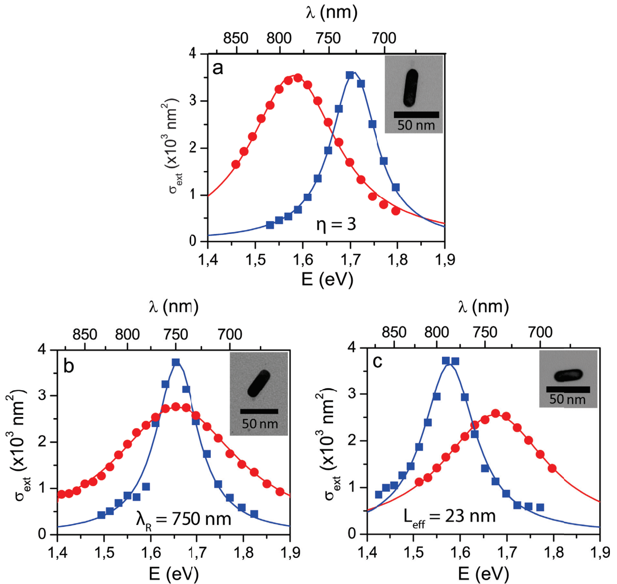
FIGURE 3.5 – a-c) Spectres absolus d’extinction longitudinaux de nanobâtonnets uniques (de longueur L et diamètre D , images MET en encart) sur des substrats de carbone ( \bullet ) et de silice ( \blacksquare ), éclairés avec une polarisation parallèle à l’axe long. La comparaison est effectuée sur des nanobâtonnets de même rapport d’aspect \eta = L/D = 3 (a), de même longueur d’onde \lambda_R de résonance (b) et de même longueur effective L_{\text{eff}} = \sqrt{LD} = 23 \text{ nm} (c). Les lignes continues (—, —) sont les ajustements lorentziens (équation (3.1)) des spectres.
