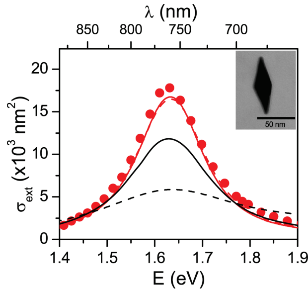
FIGURE 3.16 – Spectre d’extinction réalisé par SMS ( \bullet ) d’une bipyramide d’or ( L = 78 nm, D = 29 nm, image MET en encart) et spectres simulés correspondant dans une configuration horizontale ( \alpha = 0 et d = 2 nm, courbe —). Également représentés, les spectres calculés avec \alpha = 0 et d = 0 nm (courbe - - -), \alpha = \alpha_{max} et d = 2 nm (ligne —) et \alpha = \alpha_{max} et d = 0 nm (ligne - - -).
