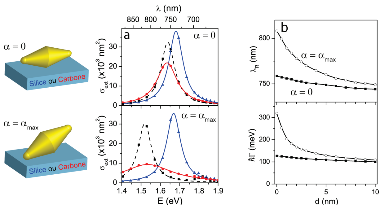
FIGURE 3.13 – a) Spectres d’extinction simulés d’une bipyramide d’or pour L = 78 nm, D = 29 nm et r = 4 nm en contact direct ( d = 0 ) avec le substrat d’épaisseur 20 nm, d’indice de réfraction n_s = 1,45 ( \blacktriangle ), n_s = 2,3 ( \blacksquare ) et n_s = 2,3 + 0,5i ( \bullet ), pour deux orientations : horizontale ( \alpha = 0 , en haut) et incliné au maximum ( \alpha = \alpha_{max} , en bas). Les lignes sont les ajustements lorentziens (équation (3.1)). c) Dépendance de la position de la résonance \lambda_R et de la largeur \Gamma avec la distance d sur la membrane en carbone, pour une orientation horizontale ( \blacksquare ) et incliné au maximum ( \circ ).
