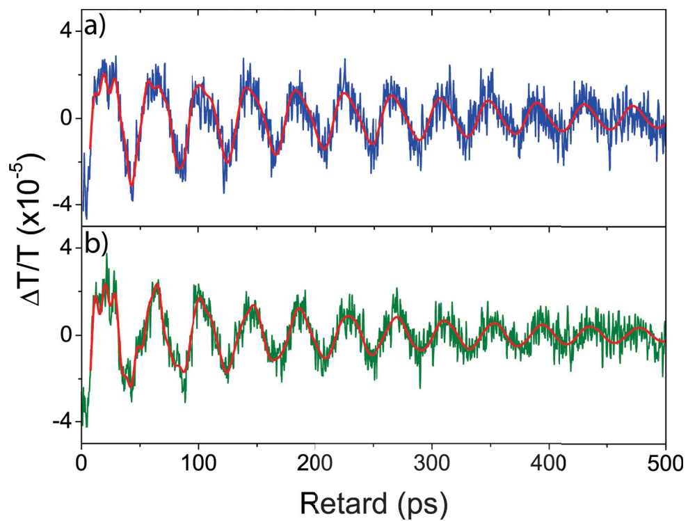
FIGURE 4.15 – a) Partie oscillante (—) du signal pompe-sonde de la figure 4.14 de BP1. b) idem pour BP2 (—). Les courbes (—) sont des ajustements par la somme de trois sinusoides amorties.
