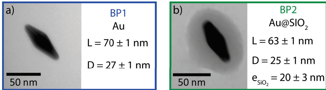
FIGURE 4.12 – a) Image MET de la bipyramide d'or BP1 (longueur L et diamètre D ) stabilisée par le PEG. (b) Image MET de la bipyramide d'or recouverte d'une couche de silice BP2 d'épaisseur e_{SiO_2} = 20 \pm 3 nm. Les tailles de la bipyramide d'or sont également indiquées.
