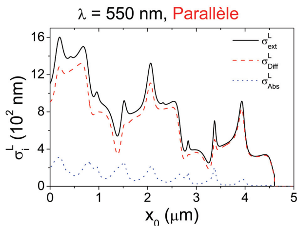
FIGURE 5.29 – Contributions de la diffusion \sigma_{diff}^L (---) et de l'absorption \sigma_{ext}^L (----) à l'extinction \sigma_{ext}^L (—) pour un cône en silicium à \lambda = 550 nm et en polarisation parallèle.
