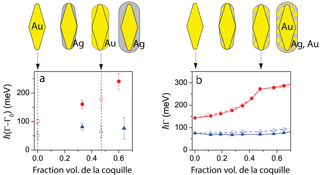
FIGURE 3.21 – a) Largeurs de la résonance plasmon pour différents nanobipyramides Au@Ag mesurées sur carbone ( \bullet , \circ ) et sur silice ( \blacktriangle , \triangle ). Les symboles vides \circ et \triangle correspondent à des nano-objets en or (bipyramide et nanobâtonnet, considéré ici comme une bipyramide d'or encapsulé par une coquille d'or). Les symboles pleins \bullet et \blacktriangle correspondent à des bipyramides entourées d'argent. La contribution intrinsèque de l'amortissement \Gamma_0 est soustraite pour s'affranchir de l'élargissement interbande survenant pour \lambda_R < 700 nm. b) Largeurs de la résonance plasmon simulées par FEM d'une bipyramide encapsulée ( L = 80 nm, D = 20 nm et r = 4 nm) sur carbone ( \bullet , \circ ) et silice ( \blacktriangle , \triangle ) en fonction de la fraction volumique de la coquille, pour des coquilles d'argent ( \bullet , \blacktriangle et courbes continues) et d'or ( \circ , \triangle et lignes tiretées).
