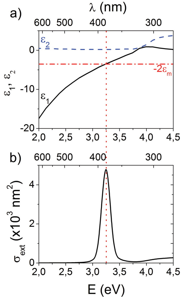
FIGURE 1.10 – a) Partie réelle ( \epsilon_1 , —) et imaginaire ( \epsilon_2 , ---) de la permittivité de l’argent. La droite (— · —) représente -2\epsilon_m avec \epsilon_m = (1,33)^2 . b) Spectre d’extinction d’une nanosphère d’argent de diamètre 20 nm dans l’eau ( n_m = 1,33 ) dans l’approximation quasi-statique (formule (1.21)). La position de la RPS ( \hbar\Omega_R \simeq 3,3 \text{ eV} , ·····) est corrélée avec l’intersection des courbes \epsilon_1 et -2\epsilon_m , soit la condition de résonance (équation (1.22)).
