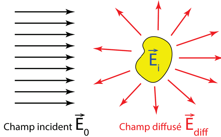
FIGURE 1.7 – Nanoparticule éclairée par une onde électromagnétique incidente (champ \vec{E}_0 ). L'interaction avec la nanoparticule produit un champ diffusé ( \vec{E}_{diff} ) et un champ interne ( \vec{E}_i ).
