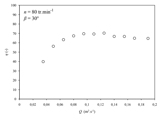
FIGURE A.7 – Rendements expérimentaux pour n = 80 \text{ tr.min}^{-1} et \beta = 30^\circ
