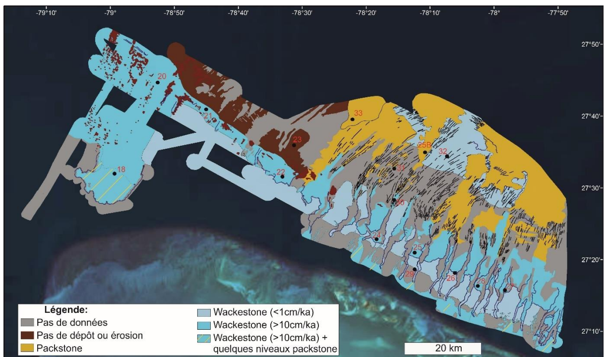
Figure 2-27: Synthèse des faciès sédimentaires en fonction des environnements morpho-sédimentaires définis par Tournadour (2015), pendant la période d'enneigement maximal du MIS 1 (0-4,4 ka cal BP).
