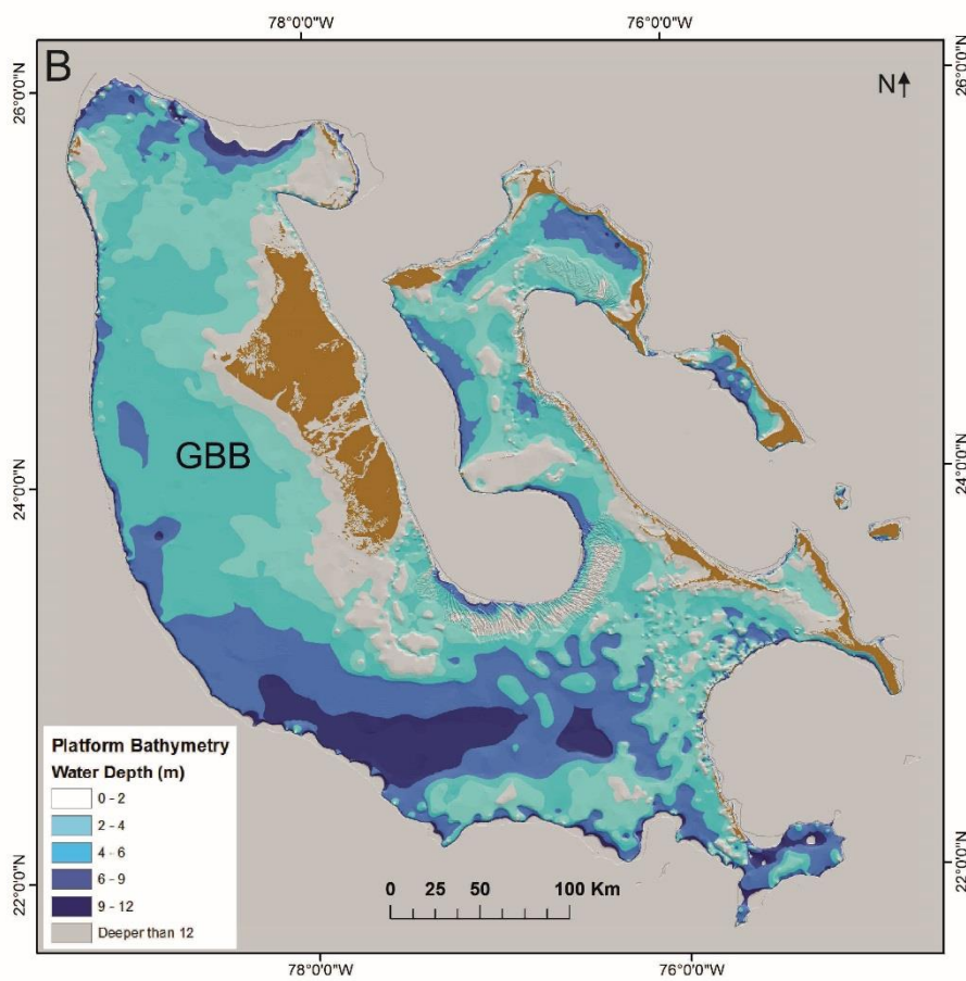
Figure 2-11: A) Carte Bathymétrique du LBB et du GBB du 14 décembre 2004 obtenues à partir des mesures du spectromètre imageur à moyenne résolution (MERIS) (Lee et al., 2010) ; B) Bathymétrie du GBB issue des sondages de bathymétrie et des mosaïques d'images satellites Landsat (Harris et al., 2014).
