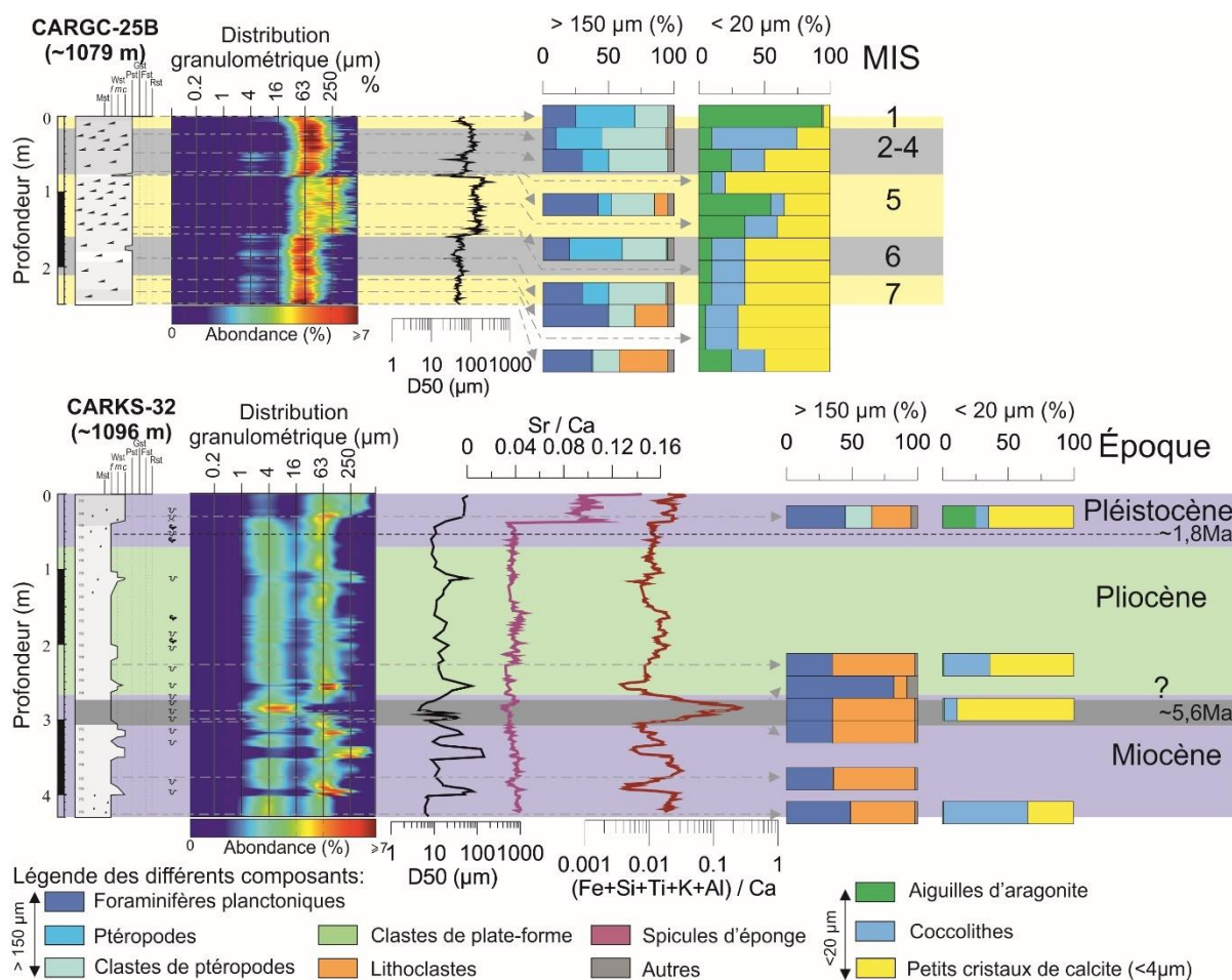
Figure 2-14: Synthèse des lithologies pour les carottes CARGC-25B et CARKS-32 montrant la distribution granulométrique, les courbes des rapports Sr/Ca et (Fe+Si+Ti+K+Al)/Ca , les pourcentages des composants principaux des fractions > 150 \mu m et < 20 \mu m ainsi que leur stratigraphie.
