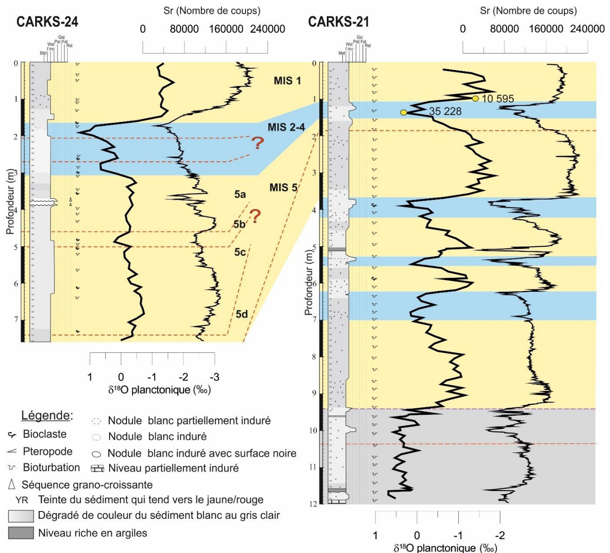
Figure 1-5: Correlations stratigraphiques entre les carottes CARKS-24 et CARKS-21 montrant la lithologie, la courbe du \delta^{18}\text{O} planctonique et le signal du strontium (nombre de coups). Les bandes jaunes indiquent les périodes interglaciaires, les bandes bleues les périodes glaciaires et les zones grisées indiquent les périodes où la stratigraphie n'est pas bien définie. Les âges indiqués sur la courbe du \delta^{18}\text{O} sont issus des datations ^{14}\text{C} et sont exprimés en années cal BP (erreurs indiquées dans le Tableau 1-1). La légende de la lithologie s'applique à tous les logs qui suivent.
