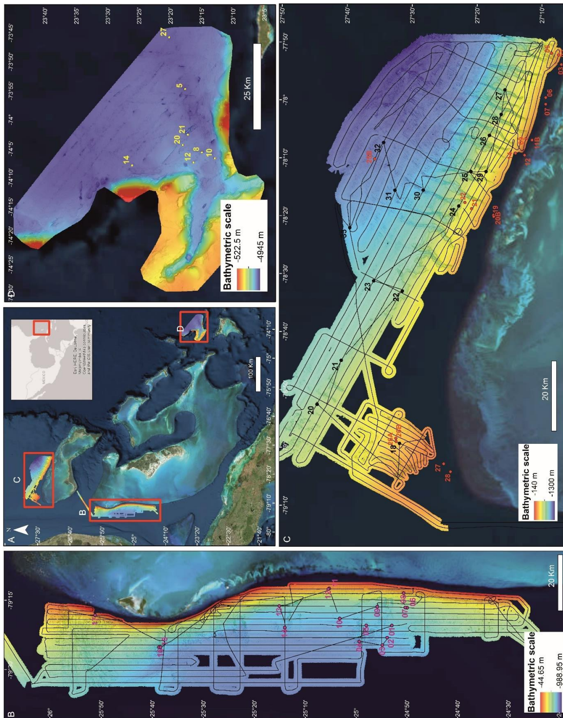
Figure 3-1: A) Carte de localisation des trois différentes zones d'étude sur les pentes des Bahamas. Les données bathymétriques, le profil de navigation pour les données CHIRP, et la position des carottes sédimentaires sont donnés par B) la zone du Leg 1 de CARAMBAR, C) zone de CARAMBAR (carottes indiquées en noir) et CARAMBAR 1.5 (carottes indiquées en rouge) et D) zone du canyon de San Salvador (BACAR 3).
