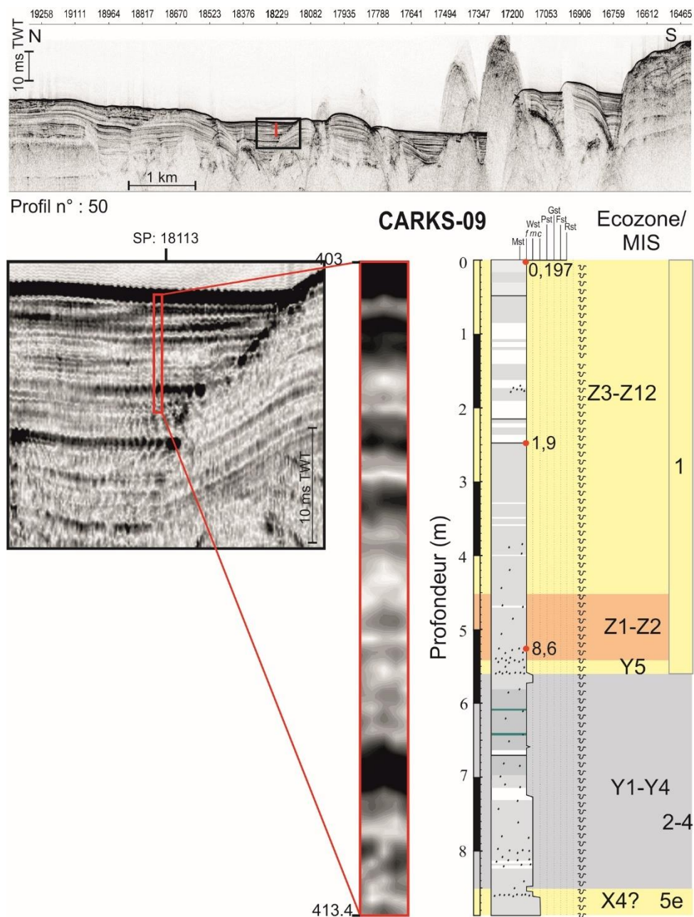
Figure 3-19: Section du profil sismique CHIRP n° 50 avec la position de la carotte CARKS-09 montrant le remplissage de la cicatrice du MTC et la corrélation des données sismiques THR avec la lithologie et la stratigraphie de la carotte.
