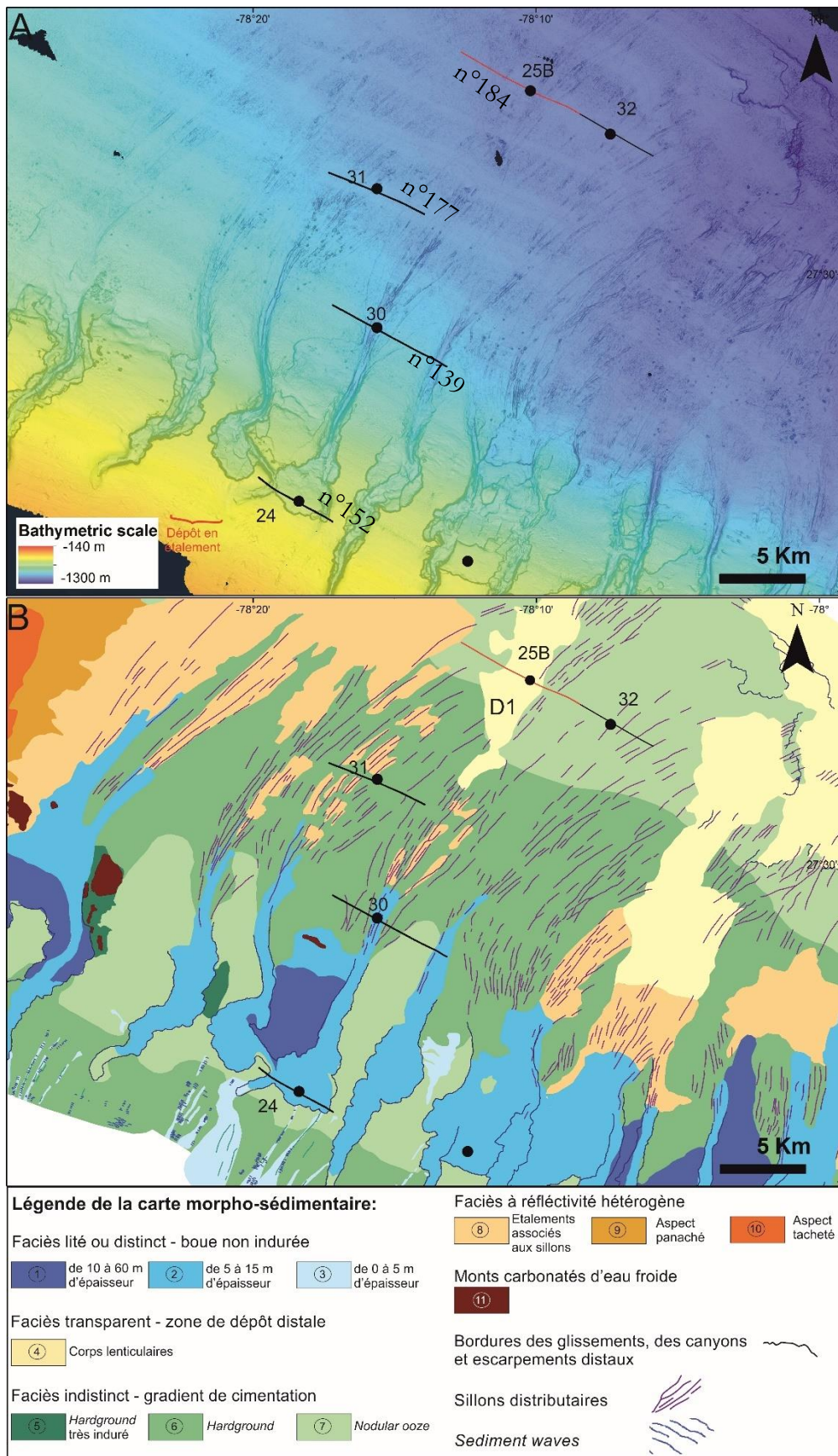
Figure 2-8: Zoom sur les carottes CARKS-24, CARKS-30, CARKS-31, CARKS-32 et CARGC-25B et localisation des profils CHIRP. A) fond bathymétrique ; B) carte morpho-sédimentaire (Tournadour, 2015). Les sediment waves sont issues de l'analyse des données bathymétriques.
