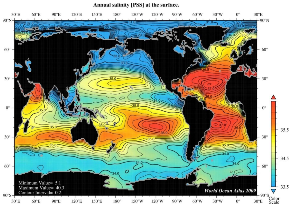
Figure 1-3: Salinité annuelle moyenne de surface à l'échelle mondiale (Antonov et al., 2010).
