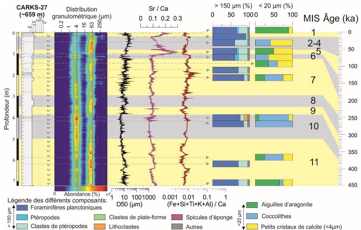
Figure 2-21: Synthèse des lithologies de la carotte CARKS-27 montrant la distribution granulométrique, les courbes des rapports Sr/Ca et (Fe+Si+Ti+K+Al)/Ca, les pourcentages des composants principaux des fractions > 150 \mu\text{m} et < 20 \mu\text{m} ainsi que leur stratigraphie.
