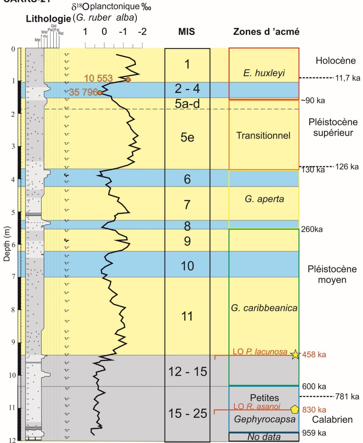
Figure 1-10: Exemple de la carotte CARKS-21 avec la lithologie, la courbe du \delta^{18}O planctonique et les âges ^{14}C en années cal. BP (erreurs dans le Tableau 1-1), les MIS ; les zones d'acmé, les âges des limites des zones d'acmé (Thierstein et al., 1977 ; Pujos, 1988 ; Sato et al., 1991 ; Raffi et al., 1993 ; Weaver, 1993) et les encadrés de couleur utilisés dans cette étude. Les bandes jaunes indiquent les périodes interglaciaires, les bandes bleues les périodes glaciaires et les bandes grisées indiquent les périodes où la stratigraphie n'est pas bien définie.
