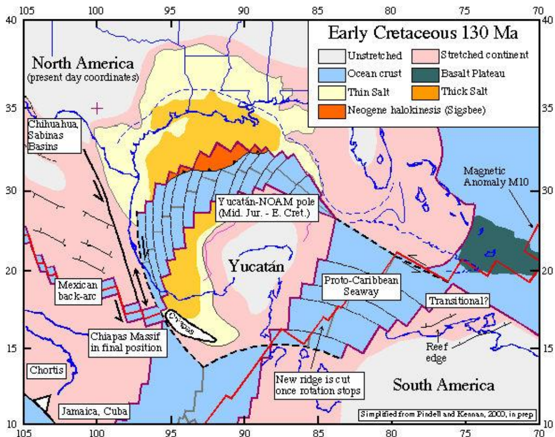
Figure 2-5: Reconstructions paléogéographiques au Crétacé inférieur (crédit de J. Pindell, L. Kennan, S. Barret).
