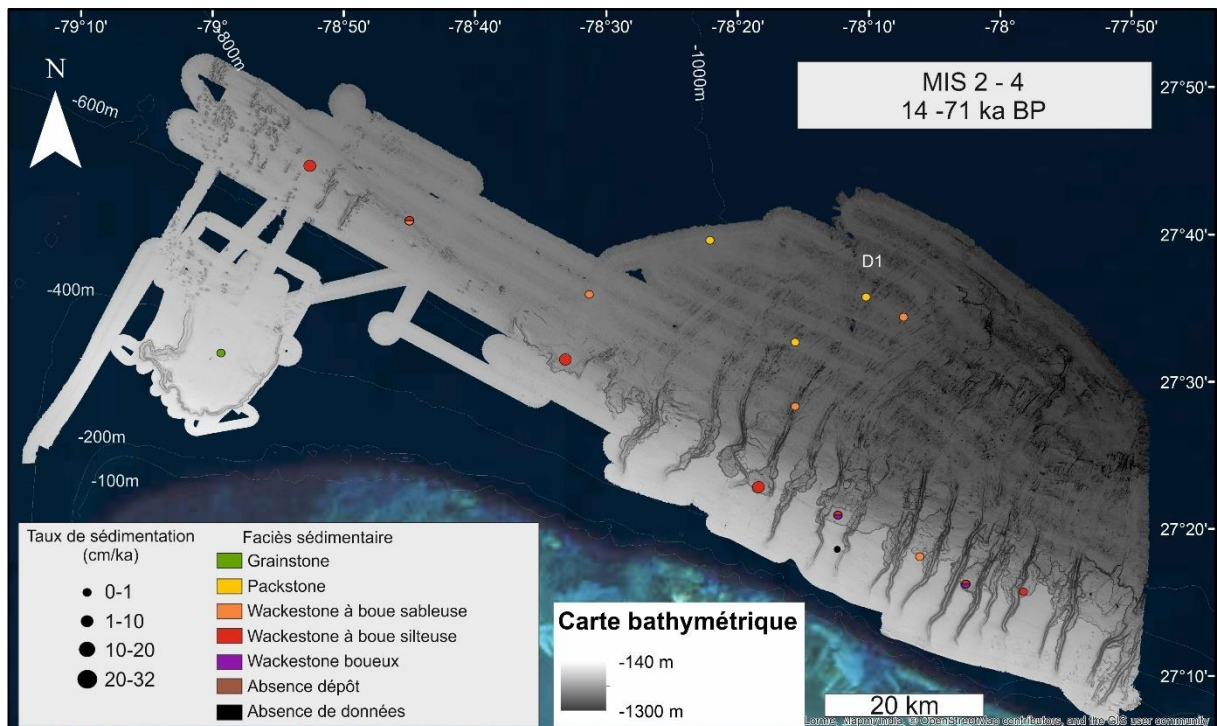
Figure 2-30: Synthèse des faciès sédimentaires et des taux de sédimentation par carotte pendant les MIS 2-4 (14-71 ka cal BP). La carte morpho-bathymétrique est issue du travail de thèse de Tournadour (2015).
