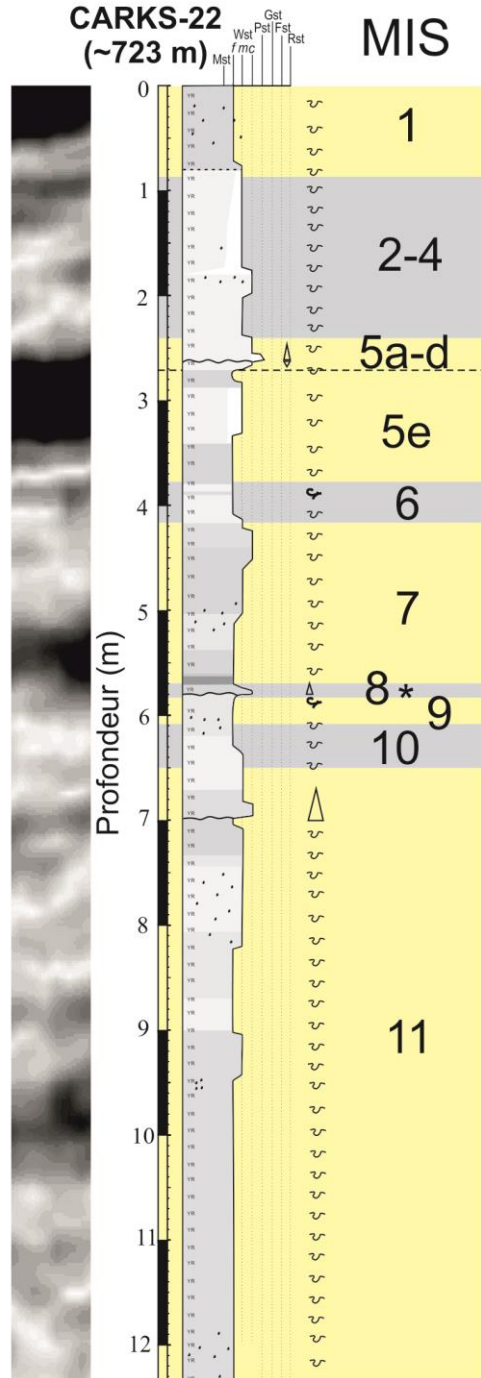
Figure 2-4: Section du profil sismique CHIRP n° 148 avec la position de la carotte CARKS-22 montrant le remplissage de la cicatrice du glissement 1 et la corrélation des données sismiques THR avec la lithologie et la stratigraphie de la carotte. Le profil sismique zoomé à l'échelle de la carotte provient du profil sismique réalisé lors du carottage, mais le trajet de ce dernier est non linéaire ce qui explique pourquoi il n'est pas présenté ici.
