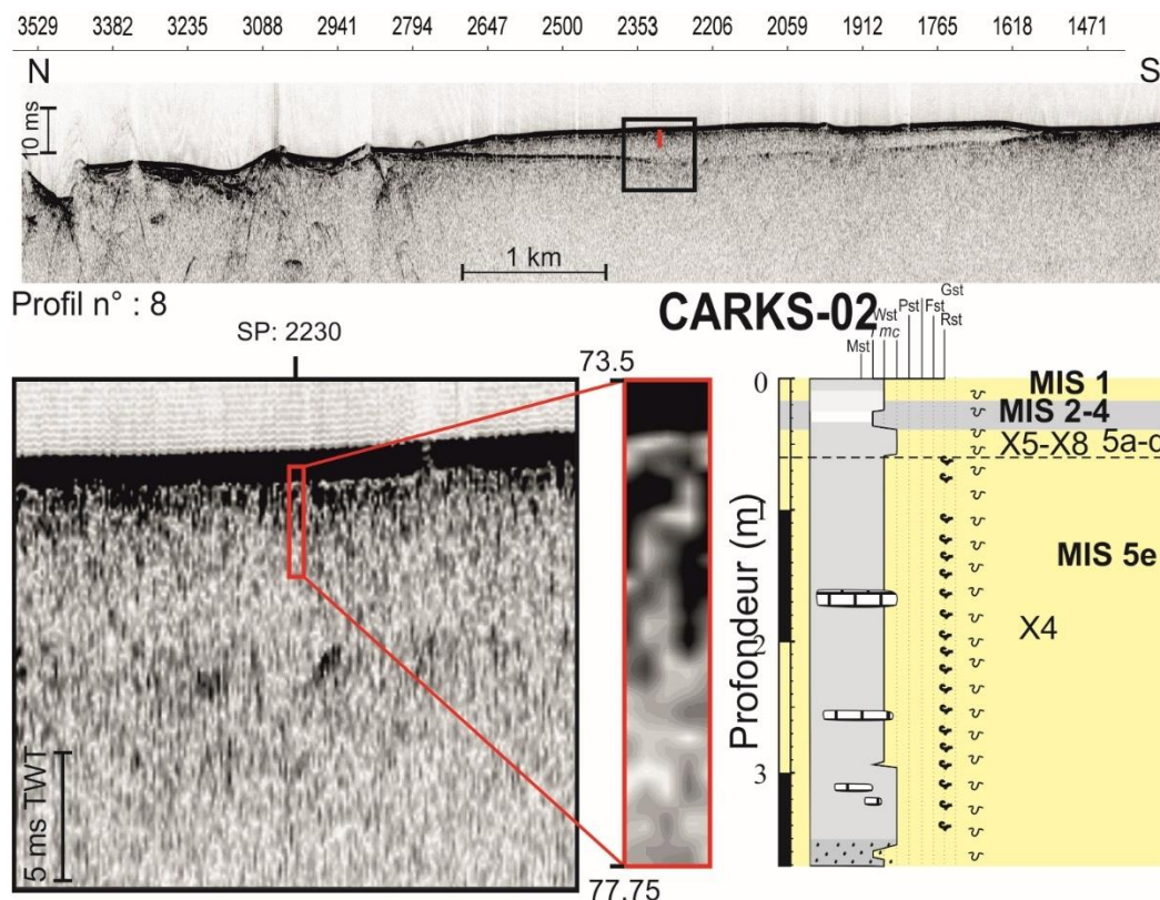
Figure 3-8: Section du profil sismique CHIRP n° 8 avec la position de la carotte CARKS-02 montrant le dépôt dans la zone médiane du lobe et la corrélation des données sismiques THR avec la lithologie et la stratigraphie de la carotte.
