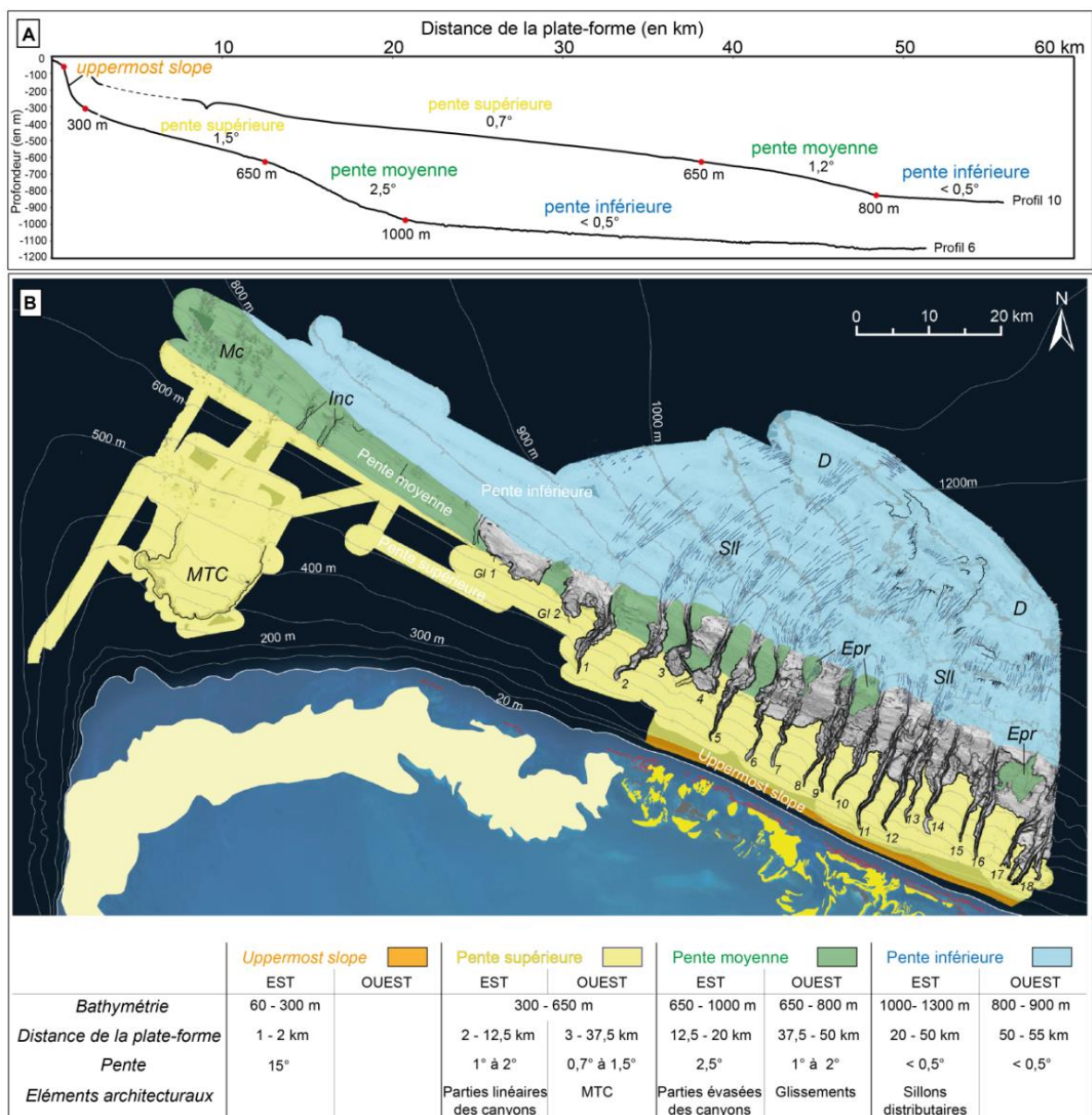
Figure 2-26: Profils de pente et localisation des différentes zones de la pente du LBB (Tournadour, 2015).
