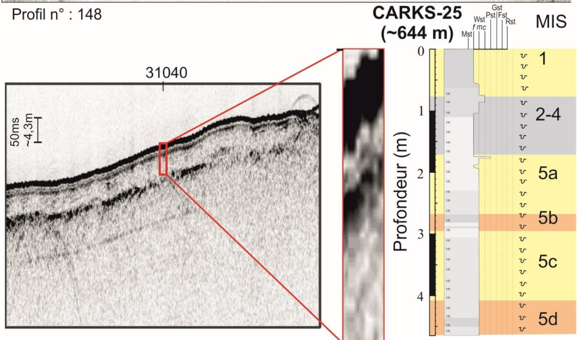
Figure 2-17: Section du profil sismique CHIRP n° 148 montrant la position de la carotte CARKS-25 dans le faciès lité de la terrasse entre les canyons 6 et 7 et corrélation avec la lithologie et la stratigraphie de la carotte.
