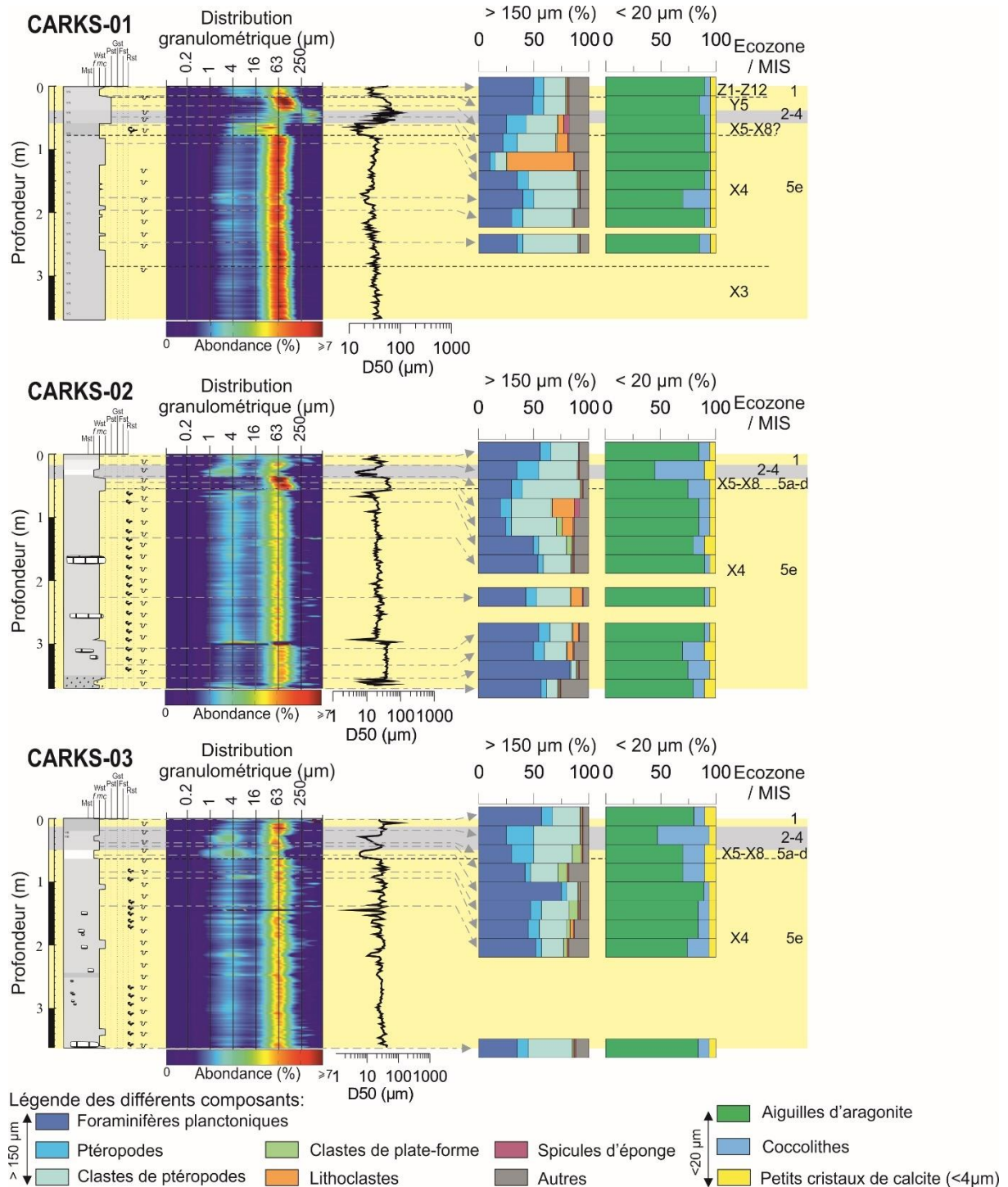
Figure 3-16: Synthèse de la lithologie des carottes CARKS-01, CARKS-02 et CARKS-03 montrant la distribution granulométrique, les courbes des rapports Sr/Ca et (\text{Fe}+\text{Si}+\text{Ti}+\text{K}+\text{Al})/\text{Ca} , les pourcentages des composants principaux des fractions > 150 \mu\text{m} et < 20 \mu\text{m} ainsi que la stratigraphie. Les analyses de constituants des carottes CARKS-01, CARKS-02 et CARKS-03 ont été réalisées par Joanna Lapuyade.
