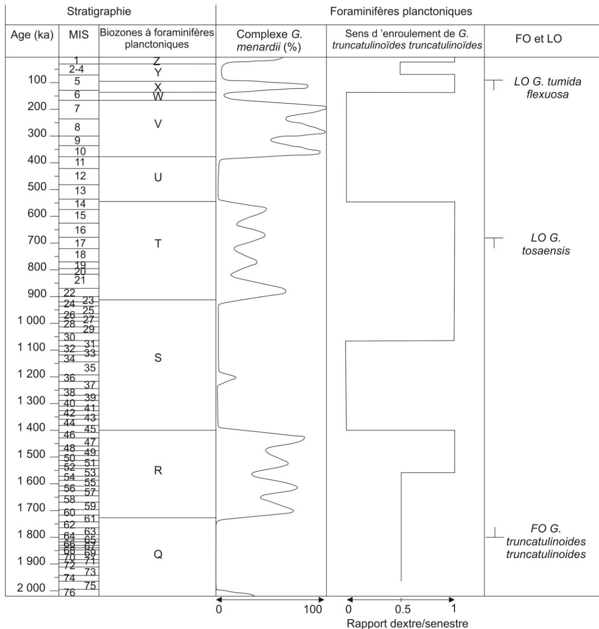
Figure 3-4: Corrélation entre une courbe généralisée des variations de fréquence du complexe G. menardii (Ericson et Wollin, 1968), avec une courbe généralisée montrant les sens d'enroulement de G. truncatulinoides truncatulinoides (Lamb et Beard, 1972), ainsi que les premières et dernières occurrences de trois espèces de foraminifères planctoniques. Les corrélations entre la courbe généralisée montrant les sens d'enroulement de G. truncatulinoides truncatulinoides et les autres courbes sont approximatives de par les indications non détaillées de la stratigraphie de Lamb et Beard, 1972. Les limites des stades isotopiques marins (MIS) sont calées sur les corrélations d'Emiliani (1966).
