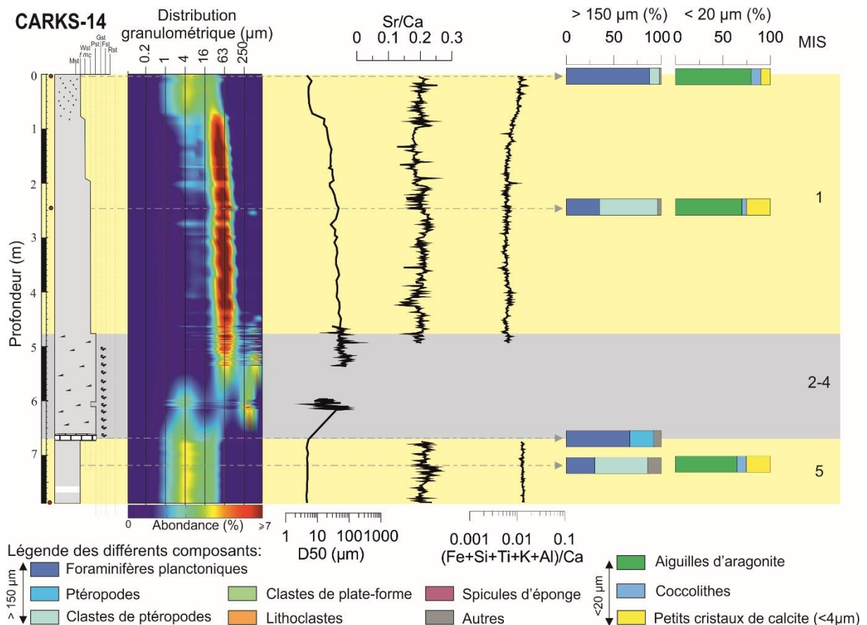
Figure 3-35: Synthèse de la lithologie de la carotte CARKS-14 montrant la distribution granulométrique, les courbes des rapports Sr/Ca et (\text{Fe}+\text{Si}+\text{Ti}+\text{K}+\text{Al})/\text{Ca} , les pourcentages des composants principaux des fractions > 150 \mu\text{m} et < 20 \mu\text{m} ainsi que la stratigraphie.
