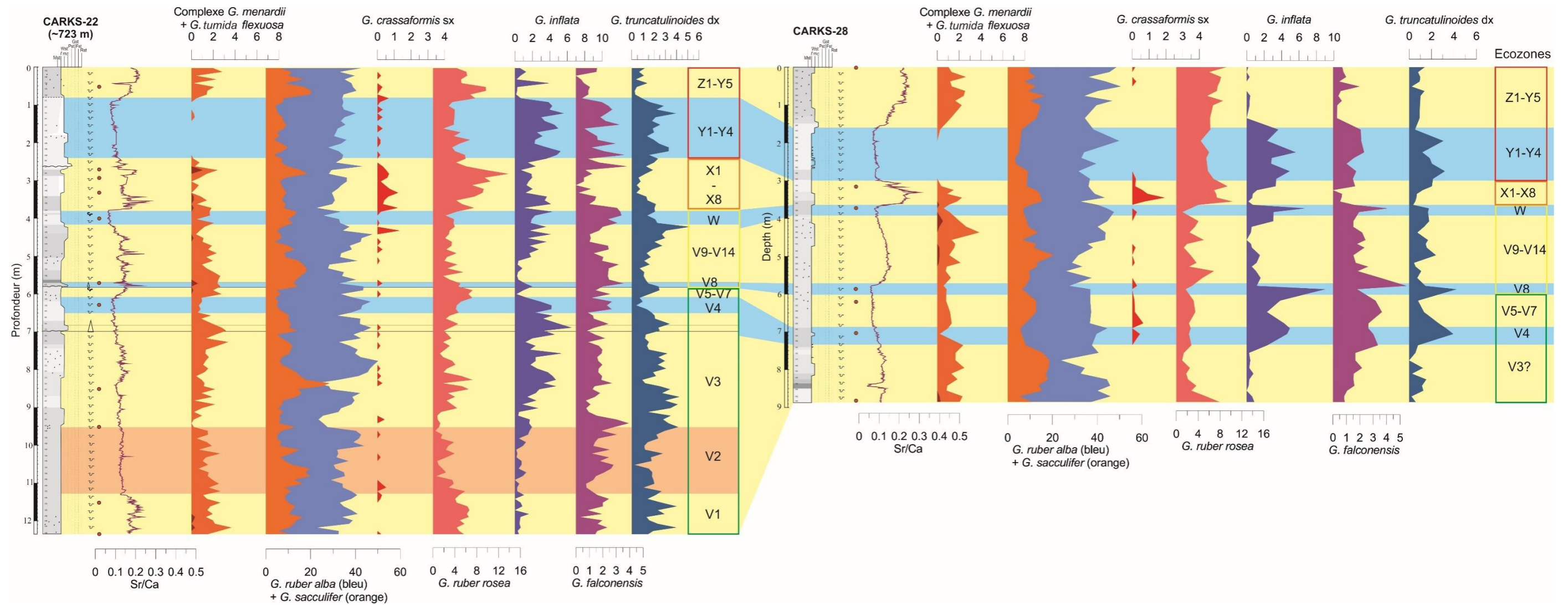
Figure 1-15: Corrélations des écozones entre les carottes du LBB CARKS-22 et CARKS-28. Les points rouges le long du log indiquent les niveaux observés pour la biostratigraphie des coccolithophores et les rectangles de couleur ainsi que l'étoile et le pentagone jaunes se réfèrent aux biozones des coccolithophores de la figure 1-8. Les bandes jaunes indiquent des écozones pendant les périodes interglaciaires et les bandes bleues indiquent des écozones pendant la dernière période glaciaire.
