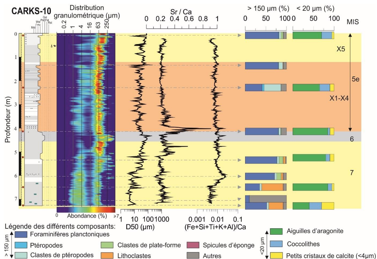
Figure 3-30: Synthèse de la lithologie de la carotte CARKS-10 montrant la distribution granulométrique, les courbes des rapports Sr/Ca et (Fe+Si+Ti+K+Al) / Ca, les pourcentages des composants principaux des fractions > 150 µm et < 20 µm ainsi que la stratigraphie.
