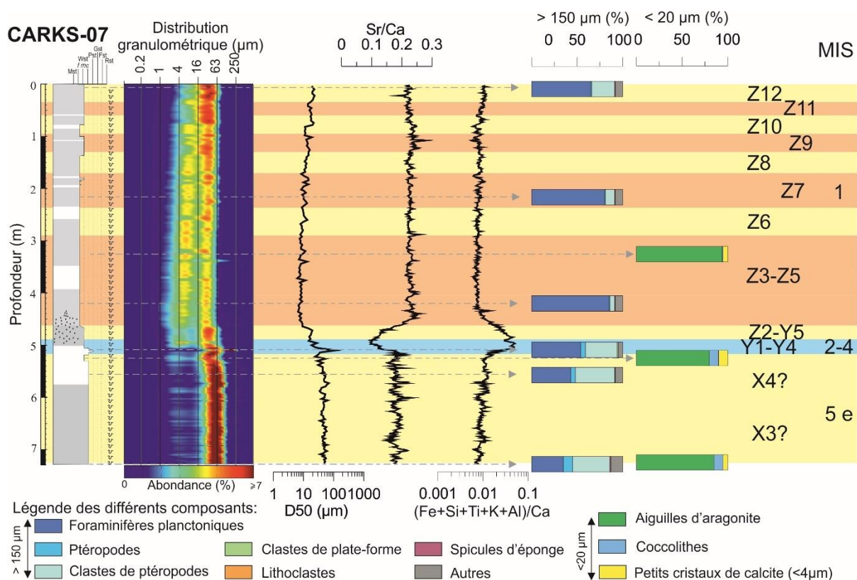
Figure 3-15: Synthèse de la lithologie de la carotte CARKS-07 montrant la distribution granulométrique, les courbes des rapports Sr/Ca et (Fe+Si+Ti+K+Al)/Ca , les pourcentages des composants principaux des fractions > 150 \mu m et < 20 \mu m ainsi que la stratigraphie.
