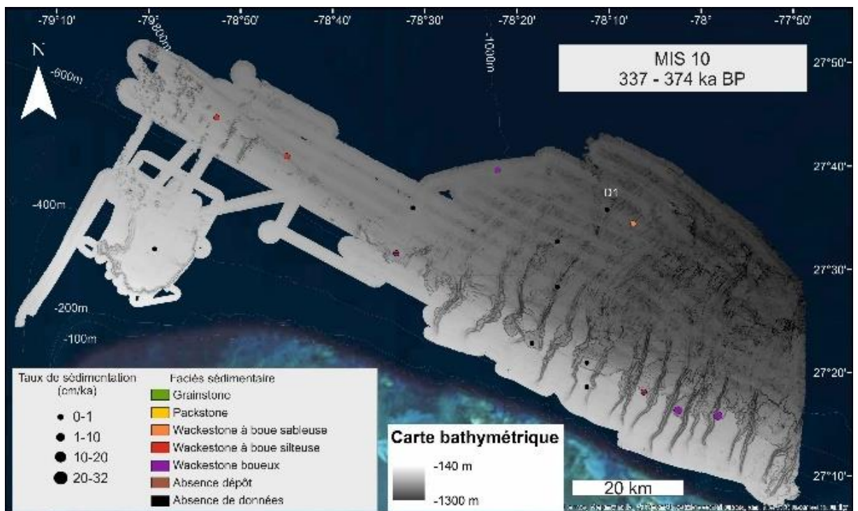
Figure 3-10: Synthèse des faciès sédimentaires et des taux de sédimentation par carotte pendant le MIS 10 (337-374 ka cal BP).
