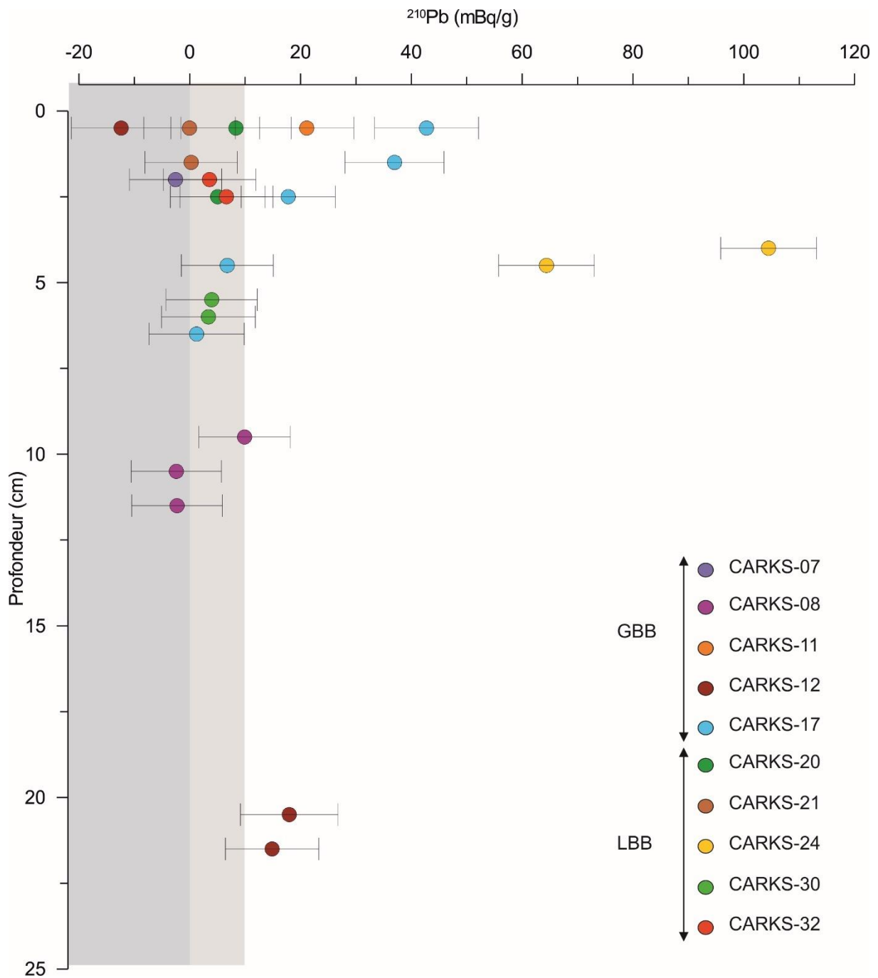
Figure 1-4: Profils du ^{210}\text{Pb}_{\text{xs}} (mBq/g) en fonction de la profondeur (cm) pour les carottes CARKE-07 à CARKE-32. Les zones grises regroupent les valeurs qui ne sont pas significatives.
