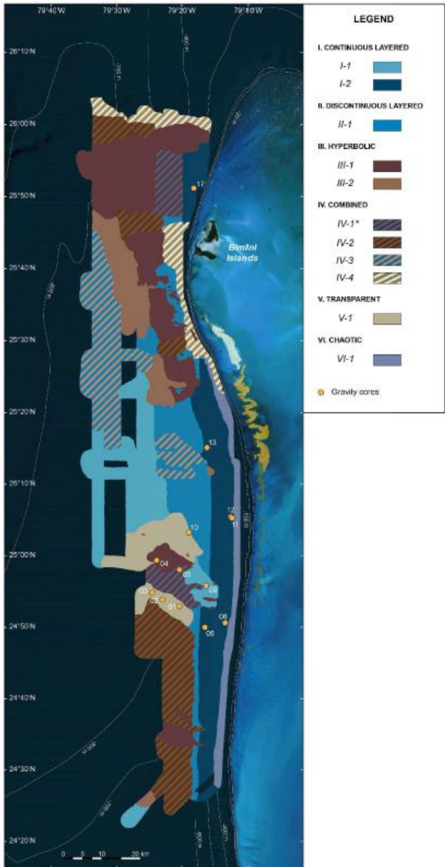
Figure 2-2: Carte de distribution des écho-faciès sur la pente nord-ouest du Great Bahama Bank.
