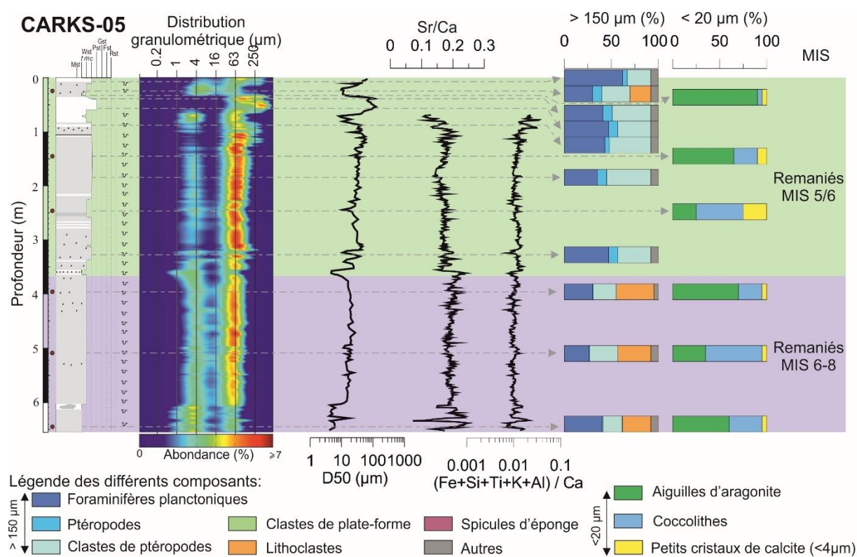
Figure 3-23: Synthèse de la lithologie de la carotte CARKS-05 montrant la distribution granulométrique, les courbes des rapports Sr/Ca et (\text{Fe}+\text{Si}+\text{Ti}+\text{K}+\text{Al})/\text{Ca} , les pourcentages des composants principaux des fractions > 150 \mu\text{m} et < 20 \mu\text{m} ainsi que la stratigraphie.
