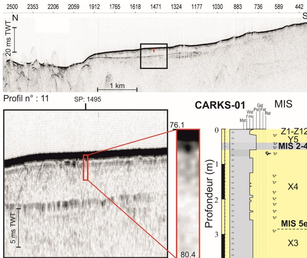
Figure 3-7: Section du profil sismique CHIRP n° 11 avec la position de la carotte CARKS-01 montrant le dépôt dans la zone proximale du lobe et la corrélation des données sismiques THR avec la lithologie et la stratigraphie de la carotte.
