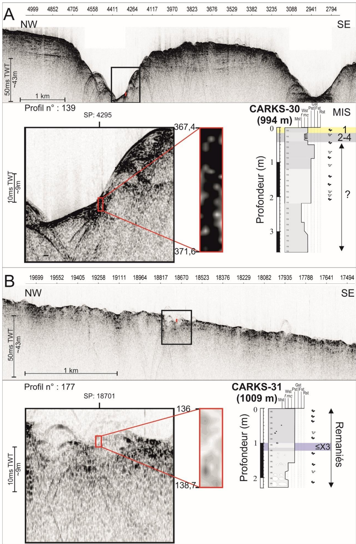
Figure 2-10: A) Section du profil sismique CHIRP n° 139 montrant la position de la carotte CARKS-30 dans le sillon distributaire et corrélation avec la lithologie de la carotte ; B) Section du profil sismique CHIRP n° 177 montrant la position de la carotte CARKS-31.
