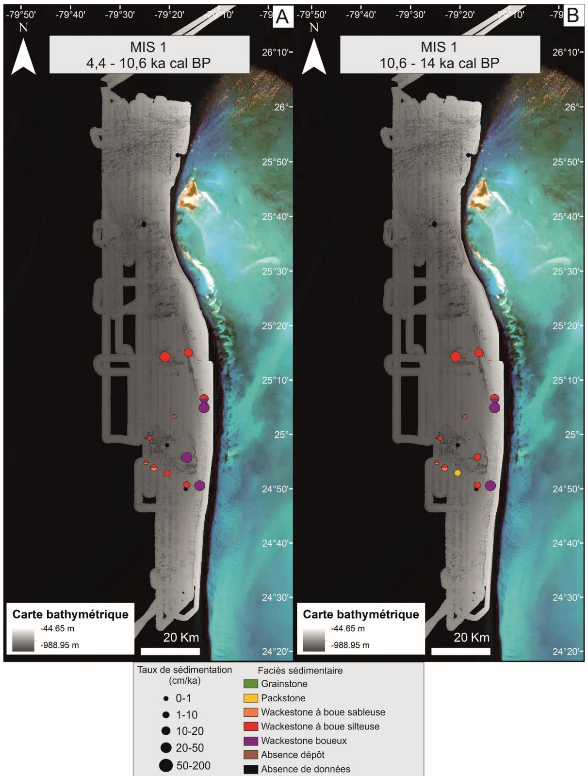
Figure 3-43: Synthèse des faciès sédimentaires et des taux de sédimentation par carotte pendant le MIS 1 A) de 6 à 10,6 ka cal BP et B) de 10,6 à 14,4 ka cal BP). La carte morpho-bathymétrique est issue du travail de thèse de Principaud (2015).
