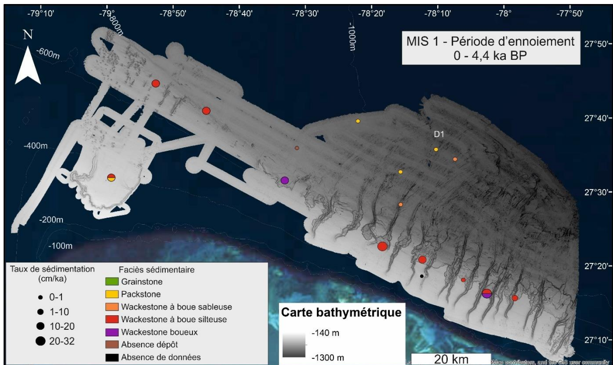
Figure 2-26: Synthèse des faciès sédimentaires et des taux de sédimentation par carotte pendant la période d'enneolement maximal de la plate-forme du MIS 1 (0-4,4 ka cal BP). La carte morpho-bathymétrique est issue du travail de thèse de Tournadour (2015).
