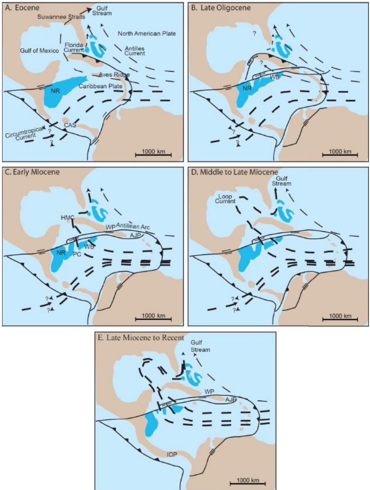
Figure 2-10: Circulation océanique de surface des régions caribéennes et bahamiennes en lien avec l'évolution tectonique (Bergman, 2005 ; modifié de Drozler et al., 1988). Les zones bleues foncées marquent les eaux peu profondes des plates-formes carbonatées.
