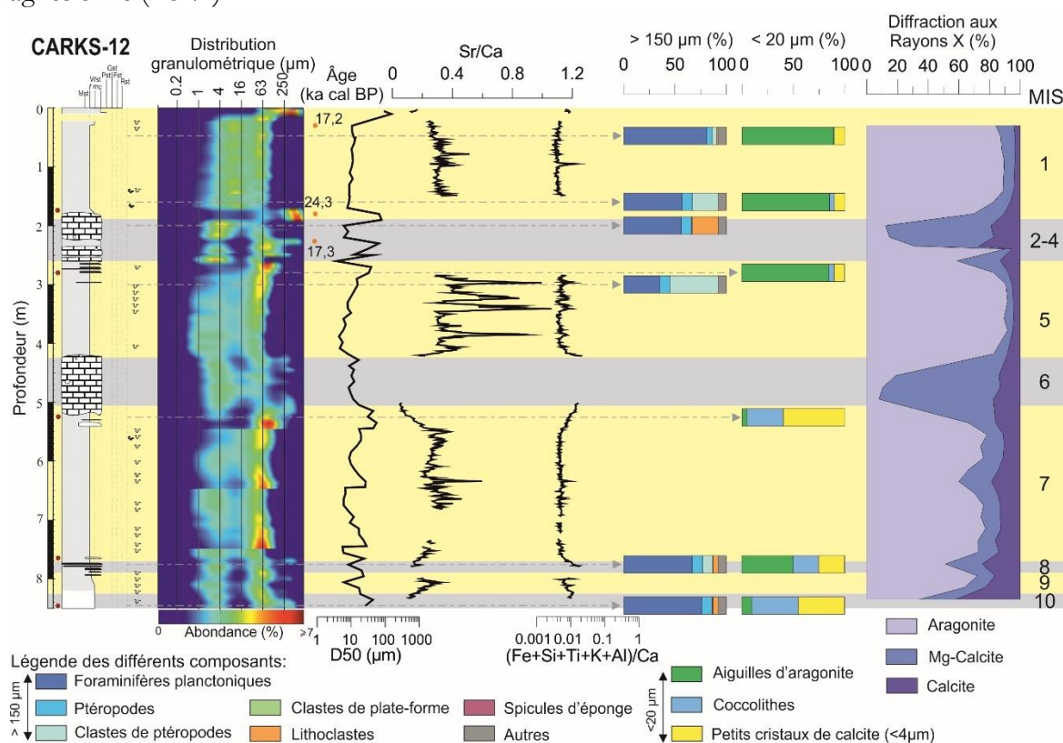
Figure 3-28: Synthèse de la lithologie de la carotte CARKS-12 montrant la distribution granulométrique, les courbes des rapports Sr/Ca et (\text{Fe}+\text{Si}+\text{Ti}+\text{K}+\text{Al})/\text{Ca} , les pourcentages des composants principaux des fractions > 150 \mu\text{m} et < 20 \mu\text{m} ainsi que la stratigraphie et les données DRX.
