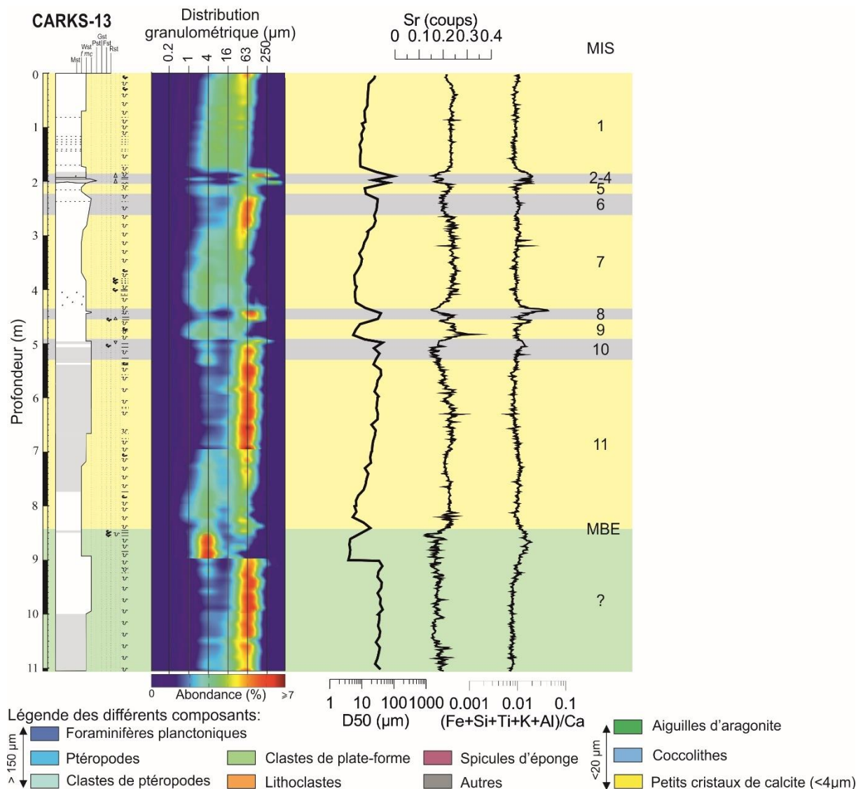
Figure 3-34: Synthèse de la lithologie de la carotte CARKS-13 montrant la distribution granulométrique, les courbes des rapports Sr/Ca et (\text{Fe}+\text{Si}+\text{Ti}+\text{K}+\text{Al})/\text{Ca} , les pourcentages des composants principaux des fractions > 150 \mu\text{m} et < 20 \mu\text{m} ainsi que la stratigraphie.
