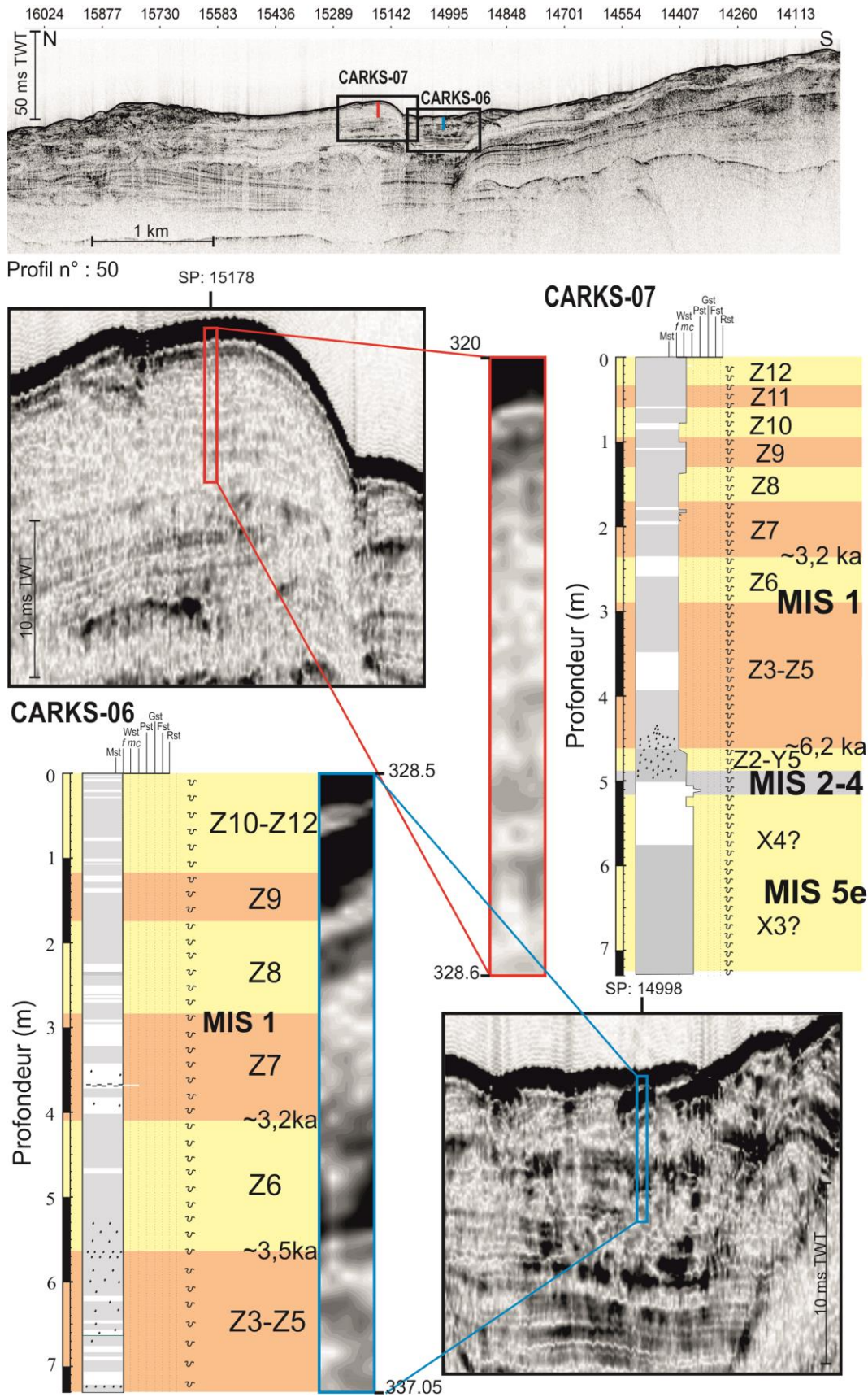
Figure 3-5: Section du profil sismique CHIRP n° 50 montrant les sédiments remplissant le système chenal-levées dans lesquels ont été prélevées les carottes CARKS-07 et CARKS-06 ainsi que la corrélation avec la lithologie et la stratigraphie des carottes.
