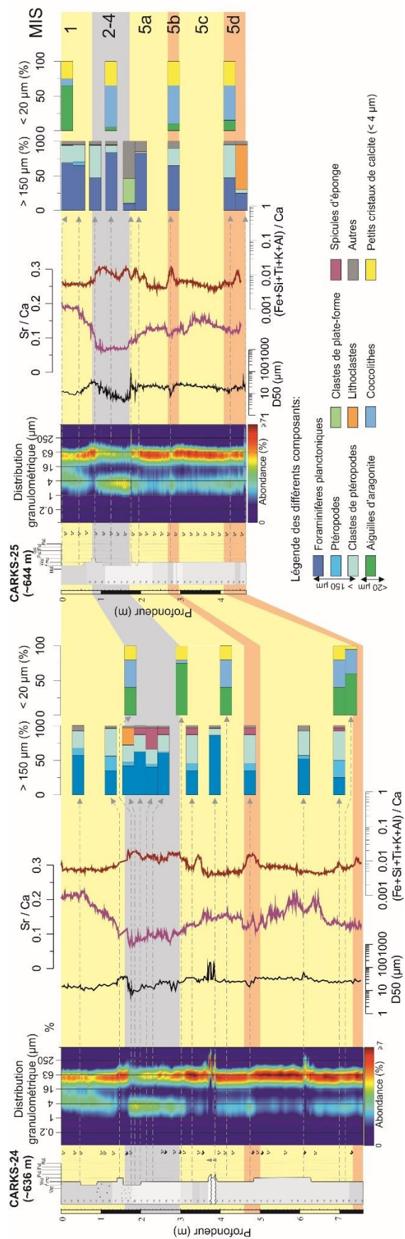
Figure 2-20: Synthèse des lithologies des carottes CARKS-24 et CARKS-25 montrant la distribution granulométrique, les courbes des rapports Sr/Ca et (\text{Fe}+\text{Si}+\text{Ti}+\text{K}+\text{Al})/\text{Ca} , les pourcentages des composants principaux des fractions > 150 \mu\text{m} et < 20 \mu\text{m} ainsi que leur stratigraphie.
