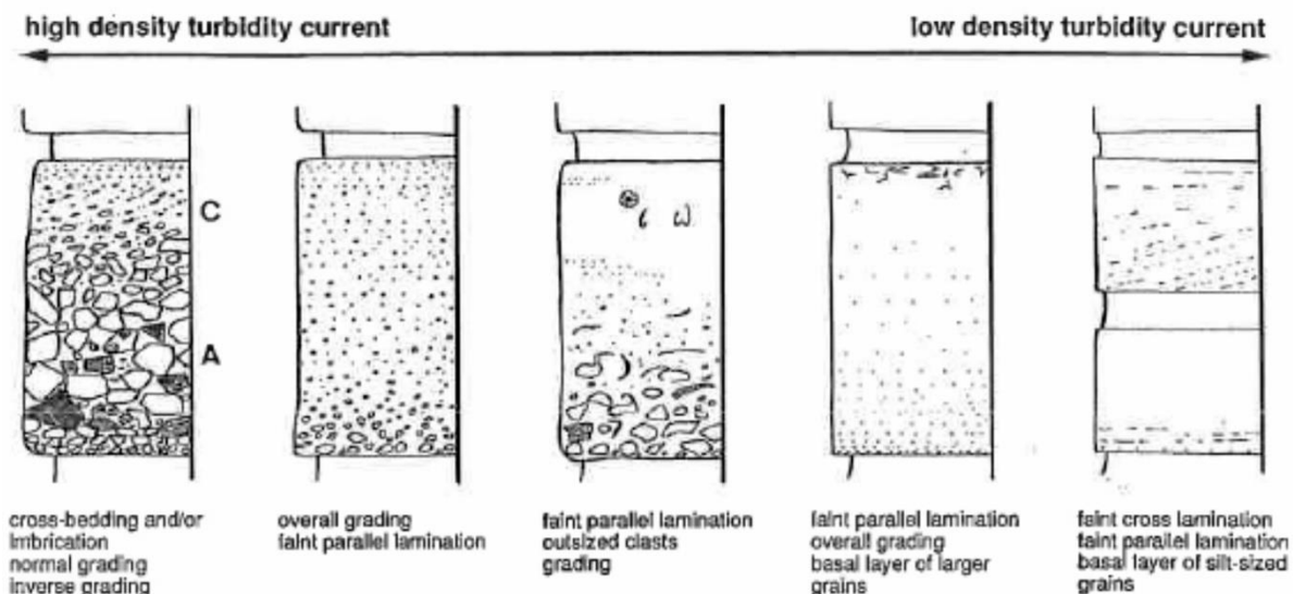
Figure 1-16: Variabilité des turbidites calcaires en raison des changements de densité du courant de turbidite (Eberli et al., 1991).
