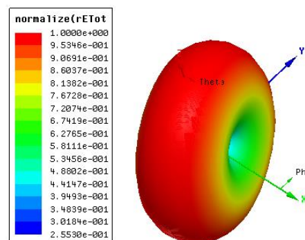
Figure 3.31 : Diagramme de rayonnement normalisé de l'antenne 868MHz obtenu avec HFSS.
