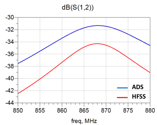
Figure 3.29 : Comparaison des coefficients de transmission calculés avec ADS et HFSS.
