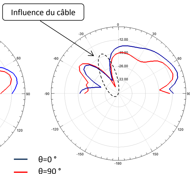
Figure 5.18 : Diagramme de rayonnement de l'antenne GPS.
