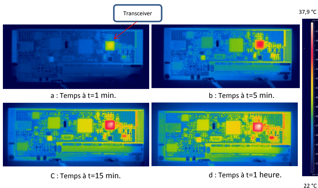
Figure 5.40 : Variation de la température du PCB du patch lors de la transmission RF.
