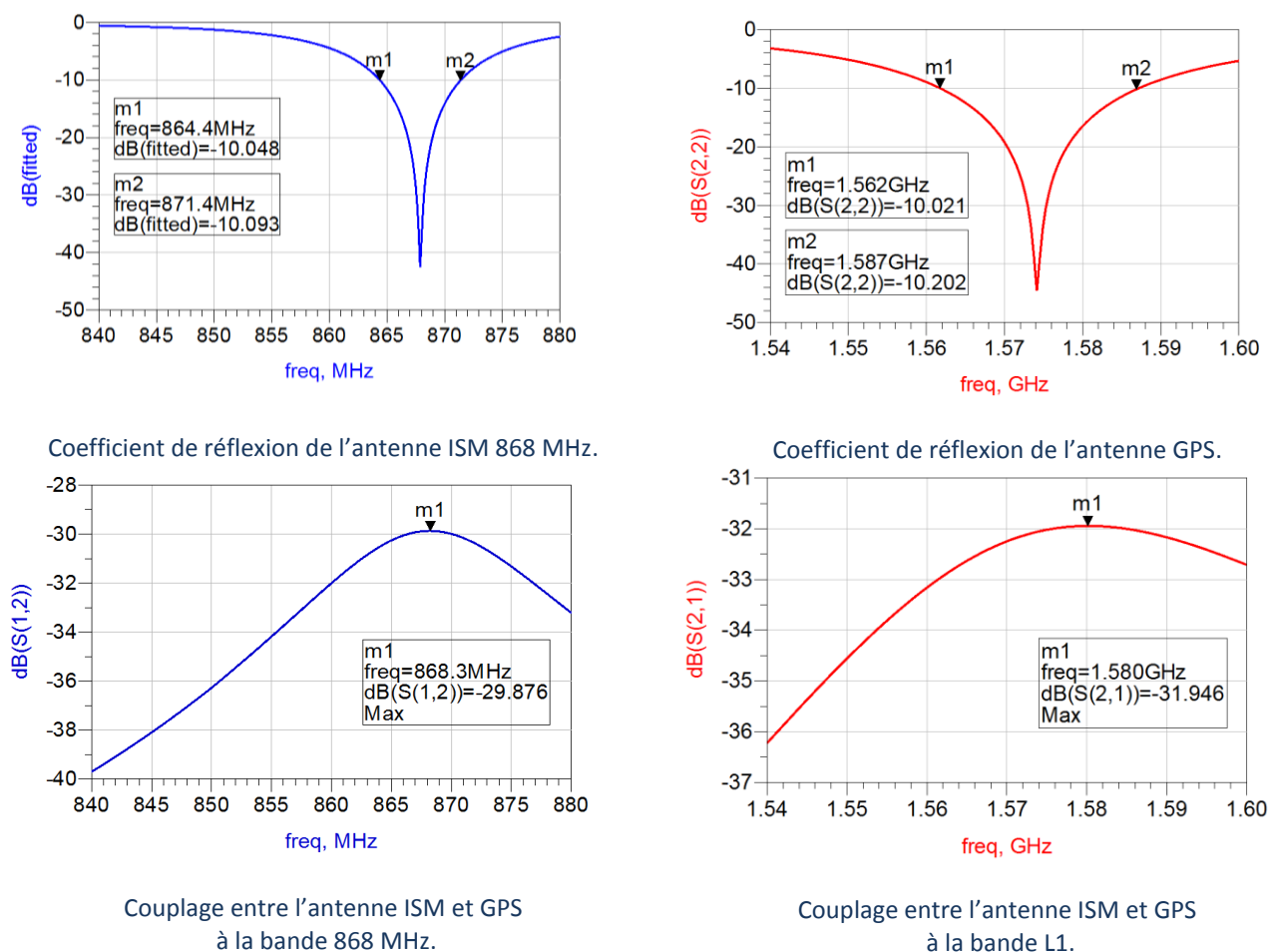
Figure 2.45 : Coefficients de réflexion et de transmission sur les bandes ISM et GPS.
