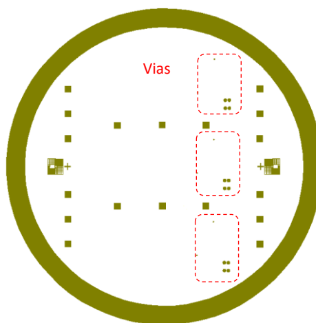
Figure 4.45 : Masque de croissance électrolytique des vias.
