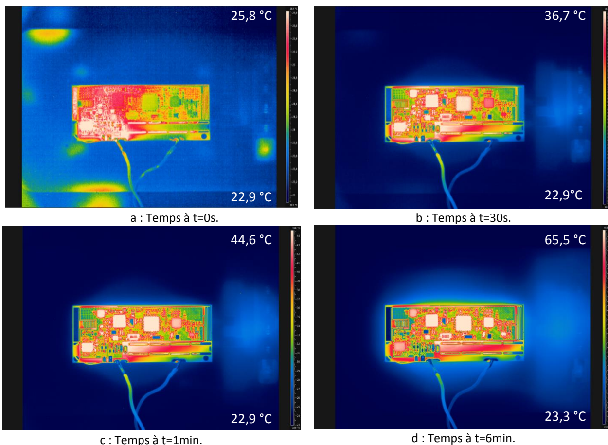
Figure 5.37 : Problématique de l'élévation thermique du patch ( T_{\max}=65^{\circ}\text{C} ) pendant la phase de recharge sans fil.
