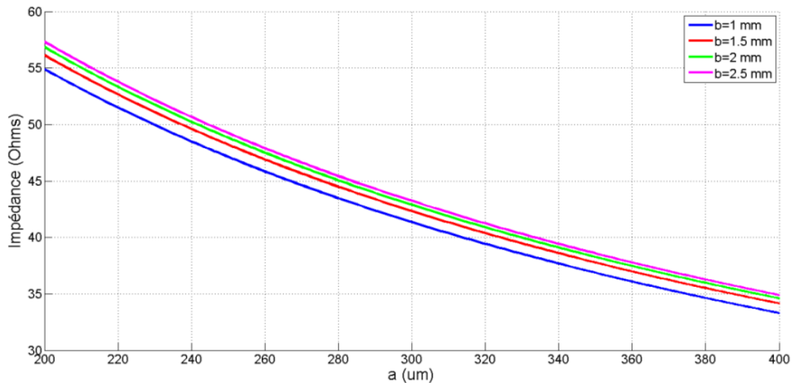
Figure 2.27 : Variation de l'impédance du guide d'onde en fonction de a ( t=40\ \mu\text{m} , h=120\ \mu\text{m} et substrat FR4).
