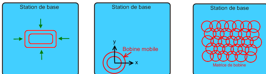
Figure 3.11 : Techniques d'alignement des bobines émettrice et réceptrice définies par le Qi.
