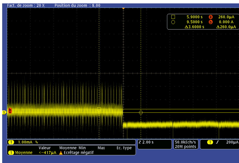
Figure 3.26 : Coupure du courant en fin de charge.
