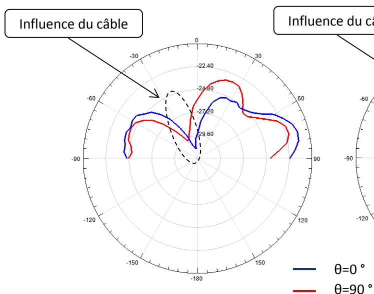
Figure 5.17 : Diagramme de rayonnement de l'antenne 868 MHz.
