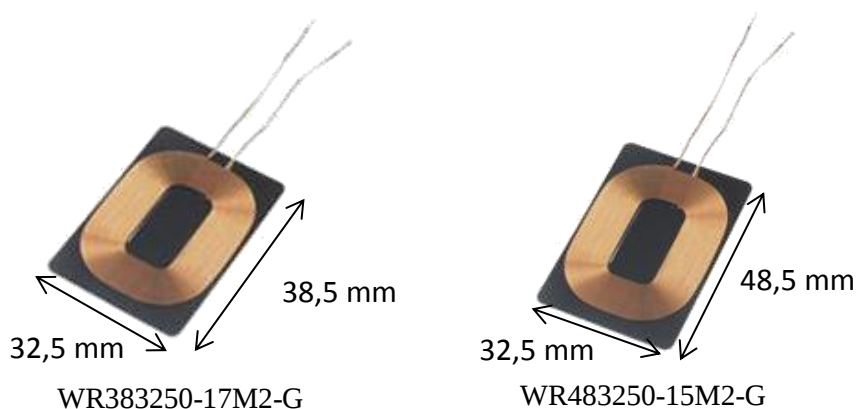
Figure 3.20 : Bobines pour la recharge sans fil [19, 20].
