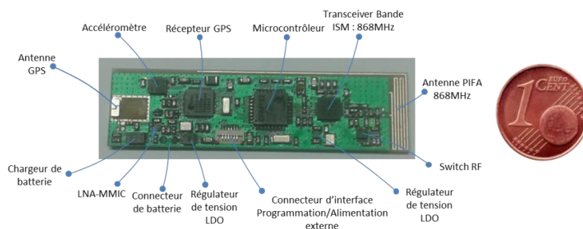
Figure 5.1 : Fonctionnalités intégrées dans le tracking patch.
