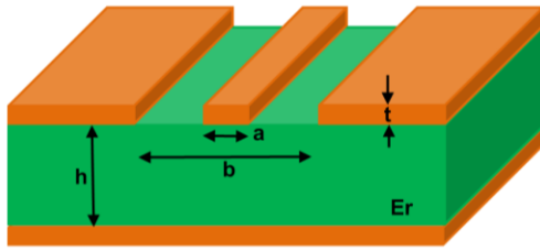
Figure 2.24 : Guide d'onde coplanaire avec plan de masse en dessous.
