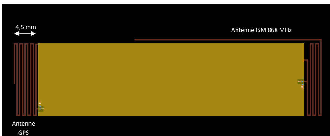
Figure 2.42 : Premier design de l'antenne GPS.
