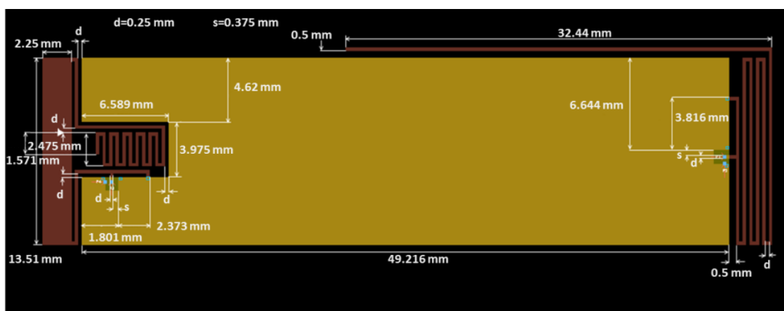
Figure 2.44 : Intégration des deux antennes GPS et ISM 868 MHz.
