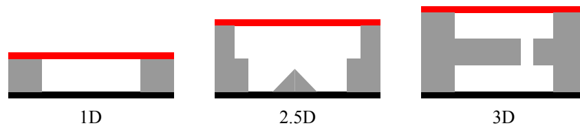
FIGURE 1.10 – Schéma de la terminologie employée pour les structures 2, 2.5D et 3D. Les couches noires et rouges représentent un substrat et un capot, respectivement. À noter : des géométries plus complexes (arcs de cercles, capillaires. . .) existent pour les structures 2.5D et 3D.
