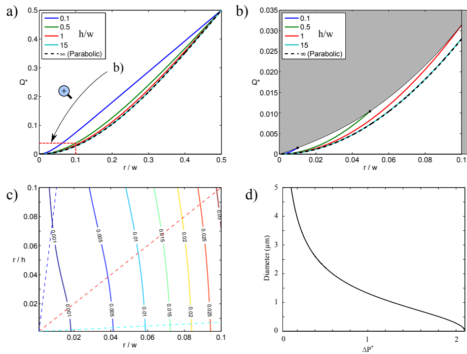
FIGURE 2.11 – Tracés pour l'étude du modèle analytique. a) Tracé de Q^* en fonction du rapport \frac{r}{w} pour différents rapports \frac{h}{w} . b) Vue zoomée de a), avec la zone grisée représentant les domaines "filtres", soit r \leq 0.1 \min(h, w) . c) Tracé de \frac{r}{h} en fonction de \frac{r}{w} pour différents Q^* . d) Variation du diamètre de coupure du dispositif 3D en fonction de \Delta P^* .
