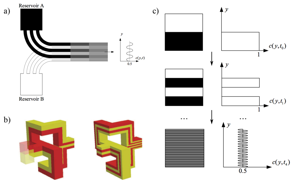
FIGURE 1.7 – Principe du laminage. a) Séparation des flux dès l'injection (nombre de fronts de diffusion déterminé) [47]. b) Structure proposée par Tan et al. [53] et étudiée numériquement par P. Carrière (illustration P. Carrière [54]). c) Principe des séparations-recombinaisons (transformation du boulanger) avec nombre de couches et profils de concentration [47].
