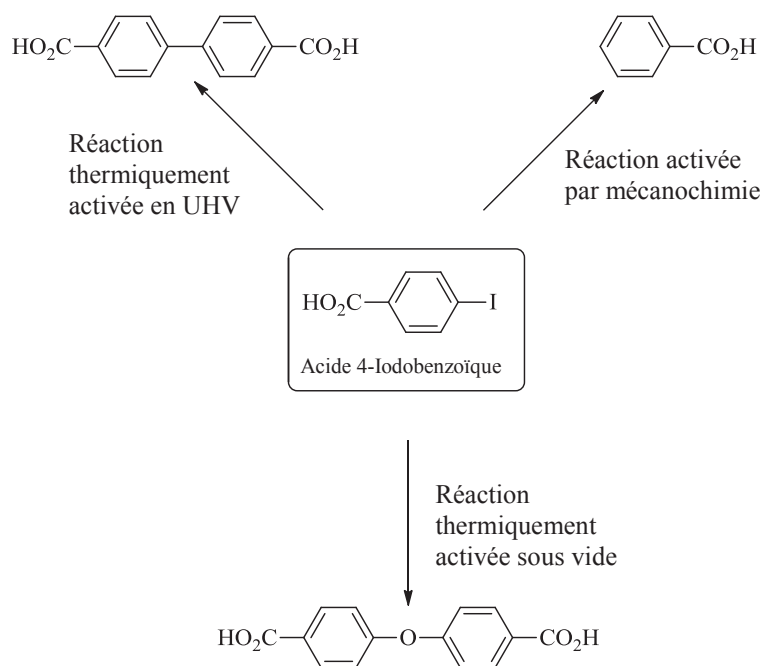
Figure 29 Schéma résumant les résultats suivant les différentes conditionnement de réaction.
