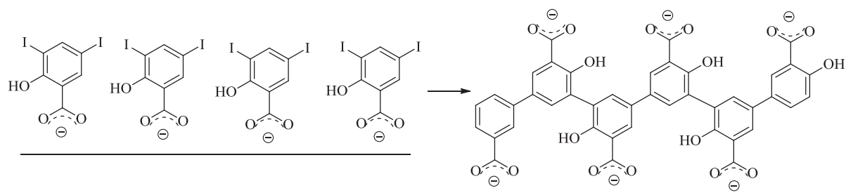
Figure 6 Mécanisme proposé pour la réaction de couplage de l'acide 3,5-diiodosalicylique (gauche vue de côté, droite vue de dessus).
