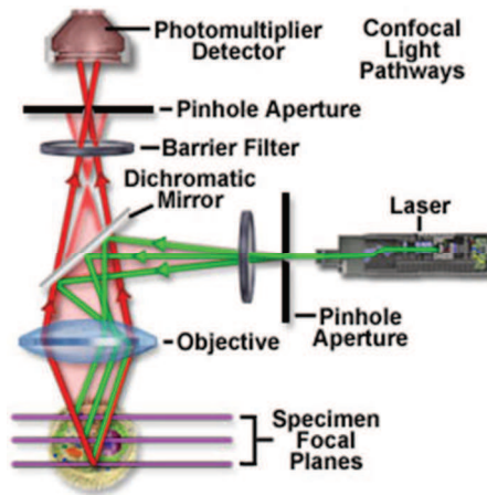
Figure 67 : Schéma du fonctionnement d'un microscope confocal.
