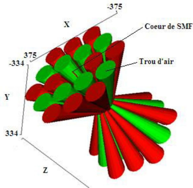
Figure II-13: Bitaper en 3D, illustrant la fibre SMF insérée dans une canne MAS
