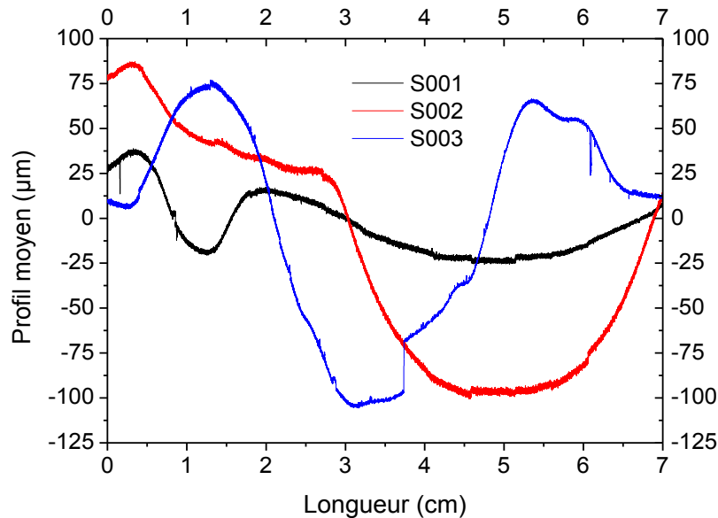
Figure IV-22: Variation du profil moyen des 3 structures dans le plan ZY
