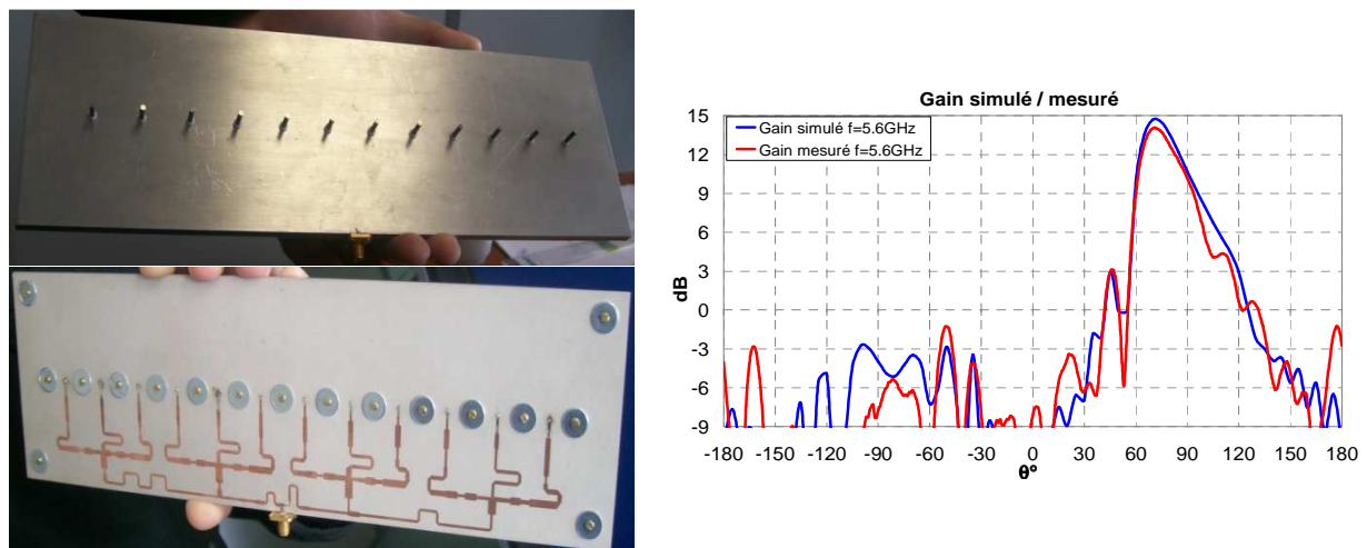
Figure I-31 : Antenne réseau composée de 12 monopoles avec le circuit de distribution (à gauche), diagramme de gain simulé et mesuré à 5.6 GHz [81].
