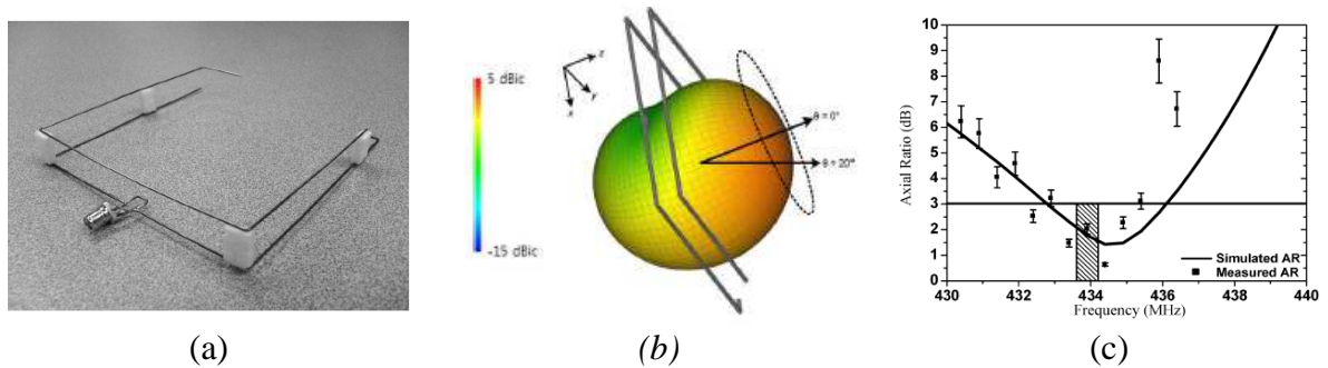
Figure I-13 : AEP à polarisation circulaire à simple excitation (a), diagramme de rayonnement 3D(b), et taux d'ellipticité dans la direction verticale à l'antenne (c) [30].
