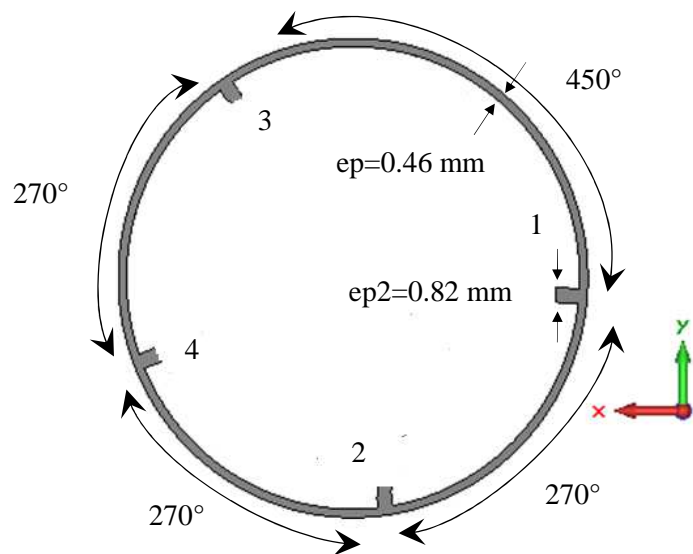
Figure III-61: Simulation d'un coupleur à 180° surdimensionné - son diamètre atteint 25.7mm, il s'inscrit dans l'emplacement disponible au dos de l'antenne plaquée.
