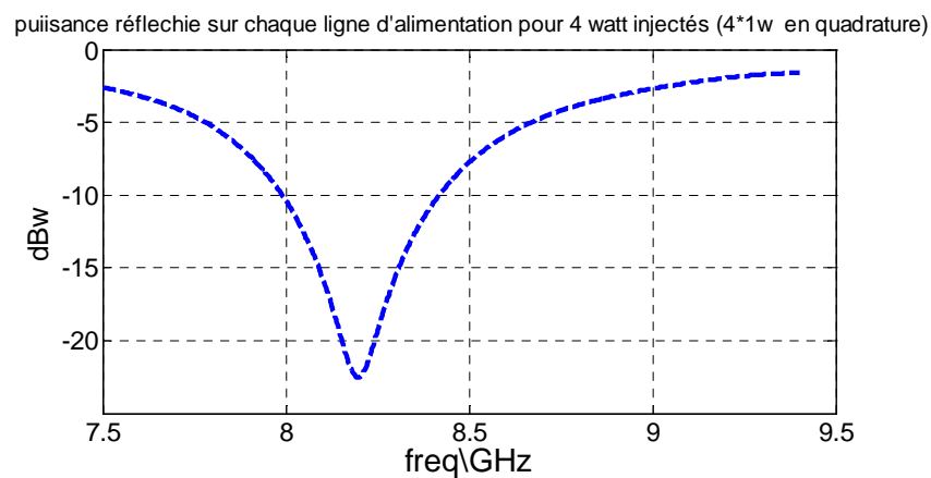
Figure III-46: Cette courbe représente la puissance réfléchie sur chaque sonde d'excitation du patch seul (Figure III-44) lorsque toutes les lignes sont alimentées simultanément en quadrature ( 4 \times 1\text{Watt} incident) en présence des lignes de découplage
