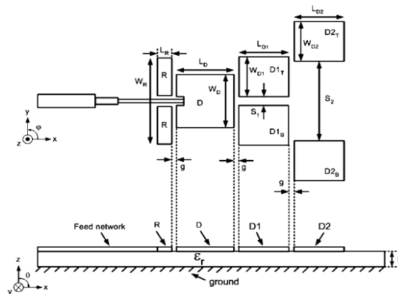
Figure I-7 : Structure d'antenne YAGI de type patch [19]
