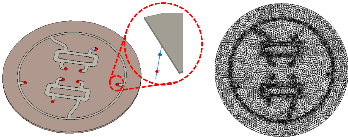
Figure A- 22 : Le circuit a été simulé avec le solveur fréquentiel de CST-MWS
