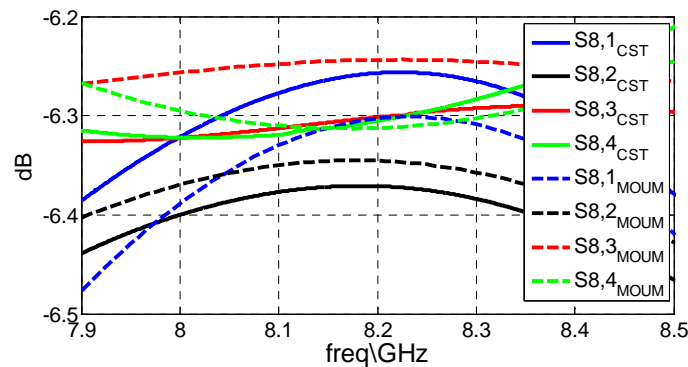
Figure A- 24: Comparaison CST et MOMENTUM des amplitudes des puissances transmises sur les 4 lignes d'alimentation du patch
