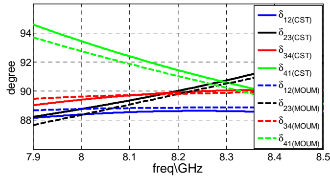
Figure A- 26 : Comparaison CST et MOMENTUM des écarts de phase [ \delta_{ij} = \angle(S_{i8}) - \angle(S_{j8}) ] montrent que l'erreur maximum reste inférieure à 2.5^\circ sur toute la bande ( |\delta_{ij}-90^\circ| < 2.5^\circ ).
