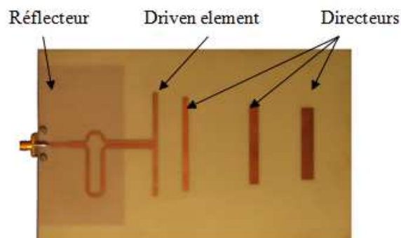
Figure I-3 : Exemple d'une antenne YAGI 5 éléments en version imprimée [7]
