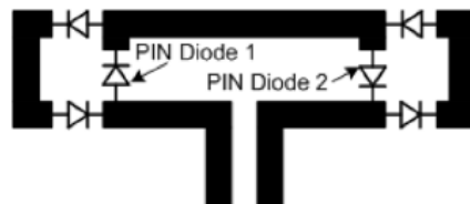
Figure I-25: Structure du dipôle replié avec des diodes PIN
