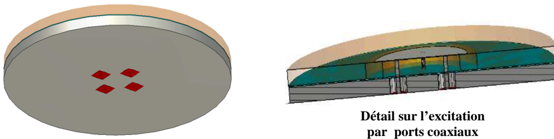
Figure A- 3 : Vue de dessus de l'antenne patch à excitation séquentielle alimentée par 4 ports coaxiaux, (à droite) détail de l'excitation
