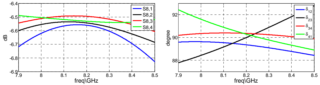
Figure IV-28 : Puissances disponibles sur les ports de sortie du circuit optimisé sur un substrat \epsilon_r=3.3
