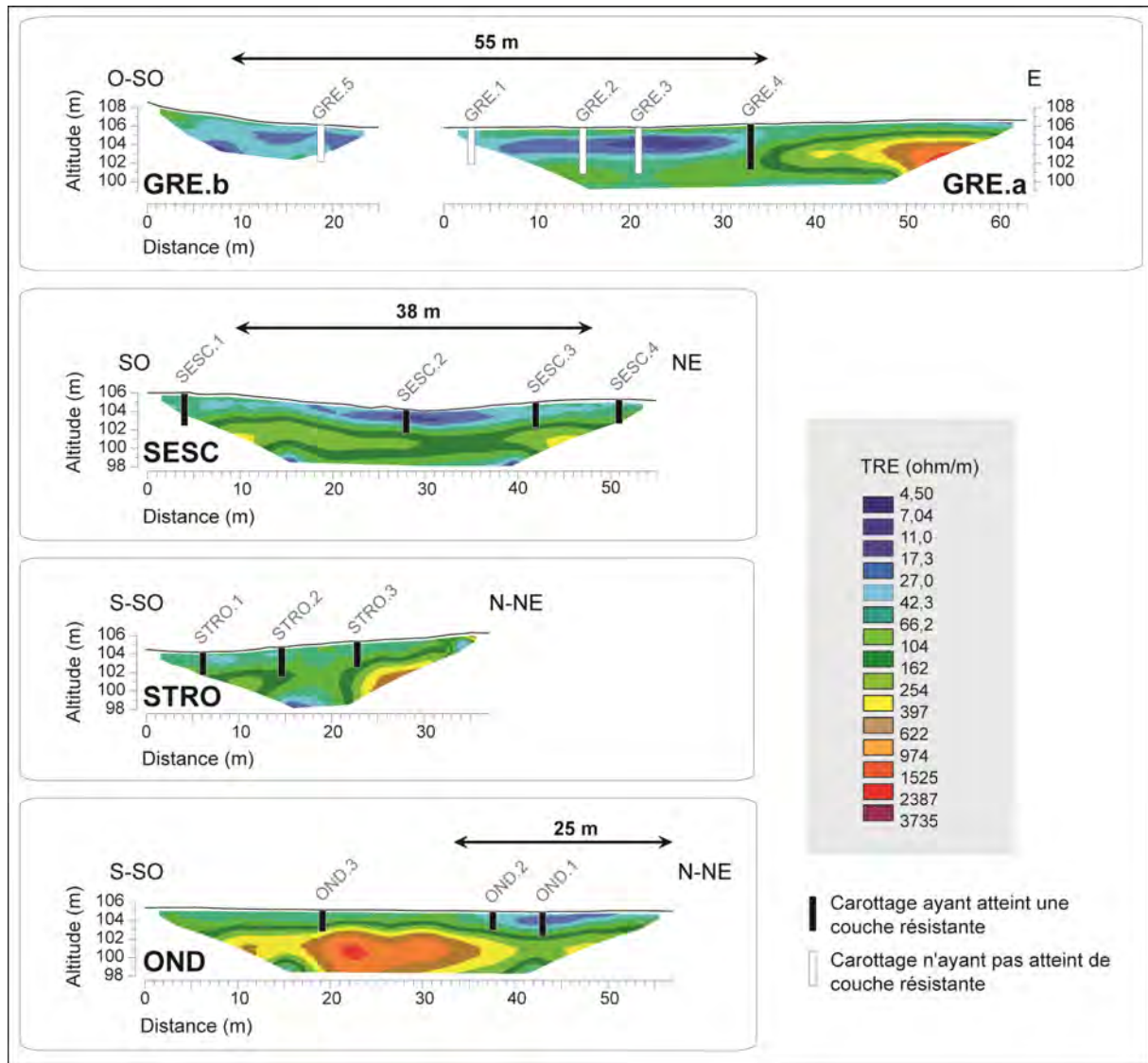
Figure 8.4 : TRE levées dans le secteur de Grenade/Ondes. Les corps dépressionnaires susceptibles de correspondre à des paléochenaux sont délimités par une double flèche.
