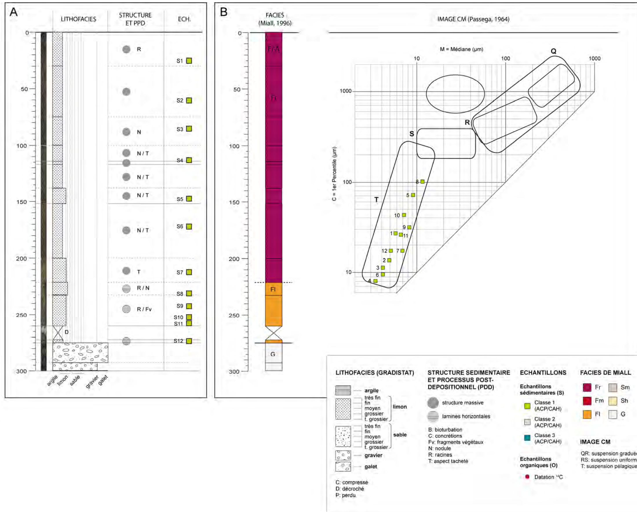
Figure 8.24 : Log sédimentaire de la carotte CORD1.1. A - Eléments de description. B - Eléments d'interprétation.
