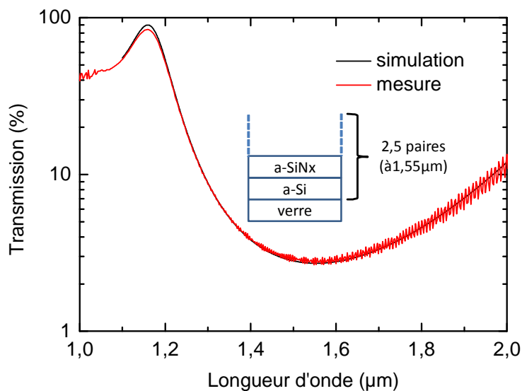
Figure II.12: spectre de transmission optique simulé et mesuré pour un miroir de Bragg composé de 2,5 paires de a-Si/a-SiN x , centré à 1,55μm et déposé sur un substrat de verre. En insert la structure utilisée
