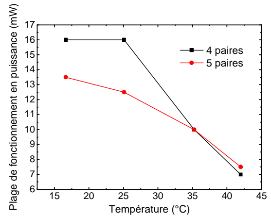
Figure III.8: Variation de la plage de fonctionnement en puissance de pompe \Delta P du VCSEL pour un miroir de 4 et 5 paires
