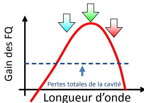
Figure II.52: principe de fonctionnement du VCSEL dans la plage du gain des FQs
