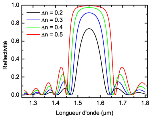
Figure I.4: réflectivité simulée d'un miroir de Bragg fictif de 20 périodes pour différents \Delta n et pour un milieu incident et un indice bas de 3.
