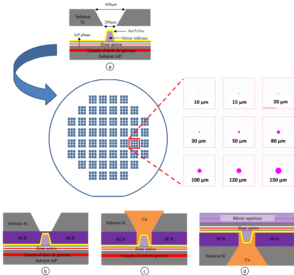
Figure IV.15 : Enchaînement des étapes technologiques des VCSELs élaborés selon le procédé de report TSHEC. L'insert au niveau de l'étape (a) représente la vue de dessus du substrat de Si au travers desquelles un alignement des miroirs de Bragg est effectué
