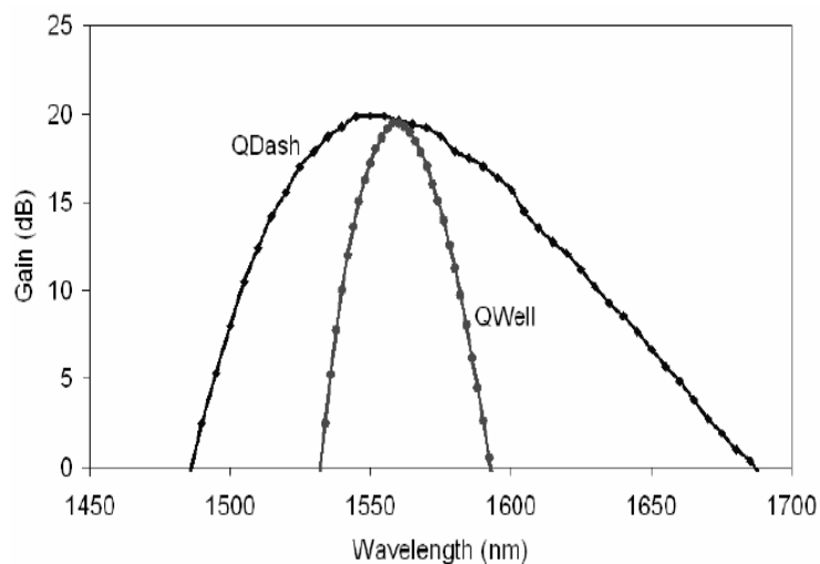
Figure II.1: Spectres de gain optique mesuré sur un SOA à FQs et PQs
