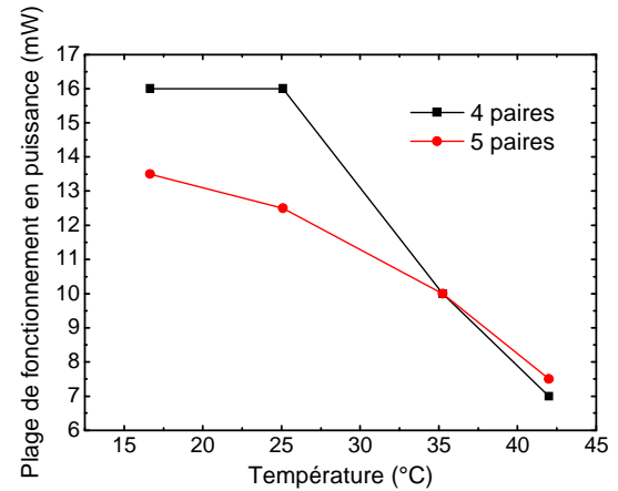
Figure III.8: Variation de la plage de fonctionnement en puissance de pompe \Delta P du VCSEL pour un miroir de 4 et 5 paires
