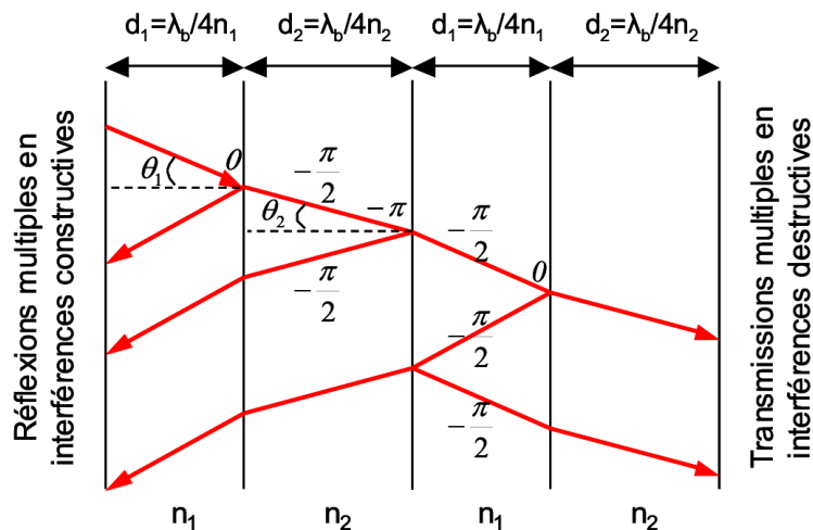
Figure I.3: Principe de fonctionnement d'un miroir de Bragg composé de deux périodes. Les déphasages induits au niveau de chaque dioptre et par la propagation dans les couches sont donnés sur la figure.
