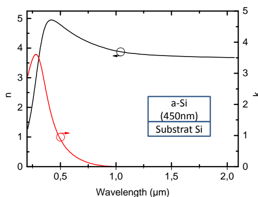
Figure II.11: indice et coefficient d'extinction du matériau a-Si, en insert la structure utilisée pour la mesure
