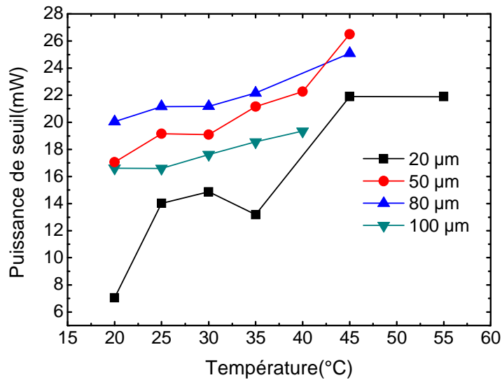
Figure IV.19: Variation de la puissance de seuil du VCSEL en fonction de la température, pour des diamètres de Bragg enterré de 20, 50, 80 et 100 µm
