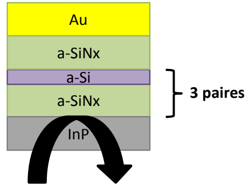
Figure III.14: miroir hybride composé d'une couche d'or et de 3,5 paires de a\text{-SiN}_x/a\text{-Si}
