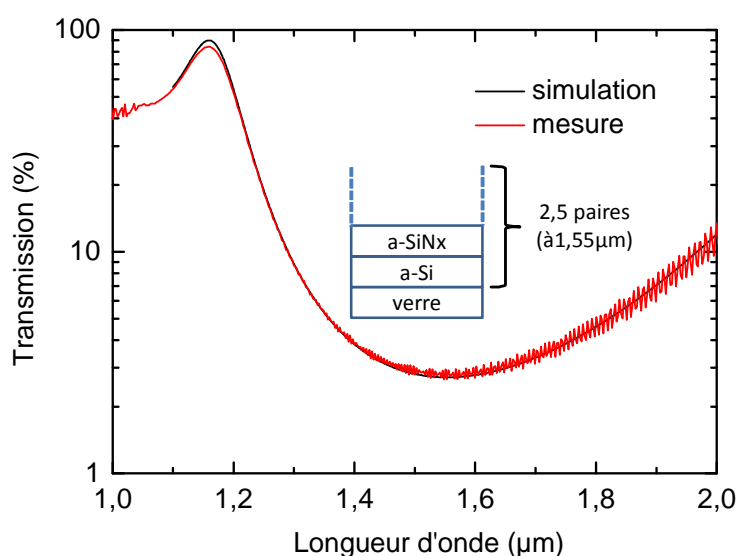
Figure II.12: spectre de transmission optique simulé et mesuré pour un miroir de Bragg composé de 2,5 paires de a-Si/a-SiN x , centré à 1,55µm et déposé sur un substrat de verre. En insert la structure utilisée
