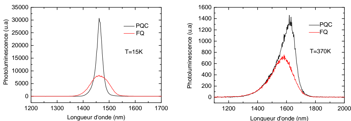
Figure II.25: Mesure de la photoluminescence sur des PQC et des FQs à deux températures différentes, avec une densité de puissance d'excitation de 700 W/cm 2
