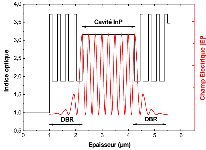
Figure 1.8: Répartition du champ et indice optique à l'intérieur d'une structure pour une émission à 1,55 μm, elle comprend une cavité d'épaisseur optique 4λ en InP et des miroirs en a-Si/a-SiN x . Le substrat est à droite de la structure et l'air est à gauche.
