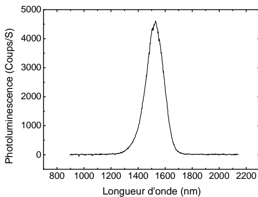
Figure II.21: Spectre de photoluminescence des FQs pris à 300 K
