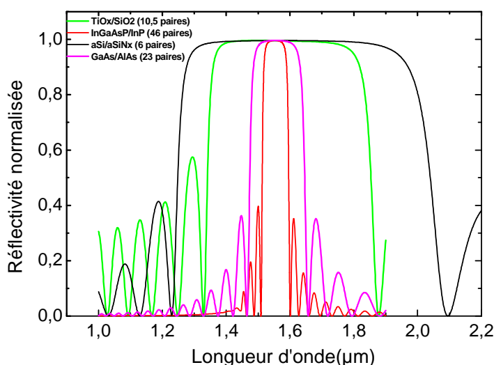
Figure II.2: Spectre de réflectivité de 4 types de miroirs: GaAs/AlAs, InGaAsP 1,44 /InP, TiO x /SiO 2 et a-Si/a-SiN x pour une résonance à 1,55 μm. Le nombre de paires de chaque miroir a été soigneusement choisi pour avoir une réflectivité maximale de 99,5%
