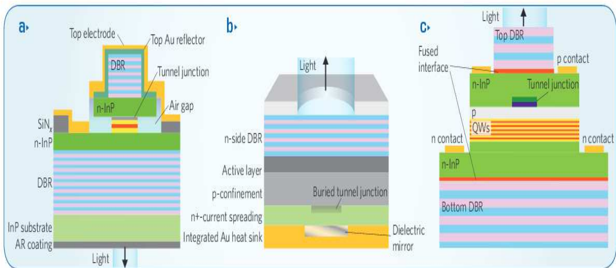
Figure 1.10: différentes configurations d'un VCSEL contenant une jonction tunnel [67], (a) : gravure sélective de la JT. (b), (c) : JT enterrée après reprise d'épitaxie
