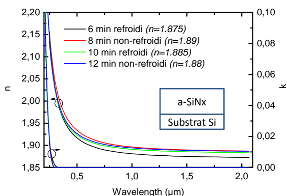
Figure II.10: indice et coefficient d'extinction du Matériau a-SiN x , en insert la structure utilisée pour la mesure
