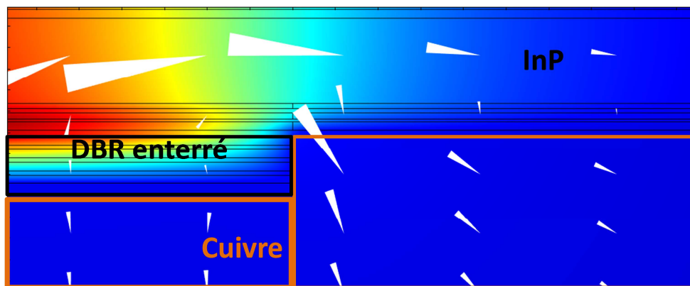
Figure III.31: Conduction thermique simulée dans un VCSEL à miroir enterré de 20 \mu\text{m} de diamètre
