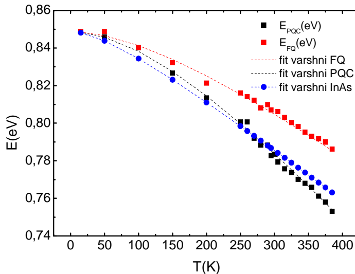
Figure II.28: Variation de l'énergie de transition (PQC et FQs) mesurée et de l'énergie de gap calculée par la loi de varshni sur toute la gamme de température
