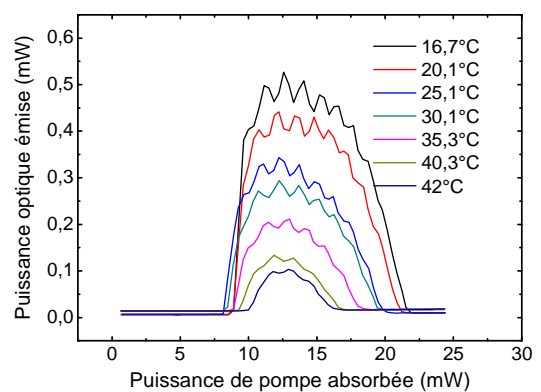
Figure III.6: Variation de la puissance émise en fonction de la température pour un miroir composé de 5 paires
