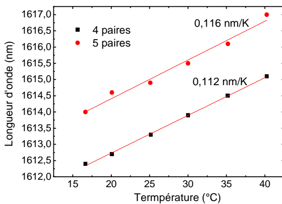
Figure III.9: Variation de la longueur d'onde d'émission du VCSEL en fonction de la température du Peltier pour un miroir de 4 et 5 paires
