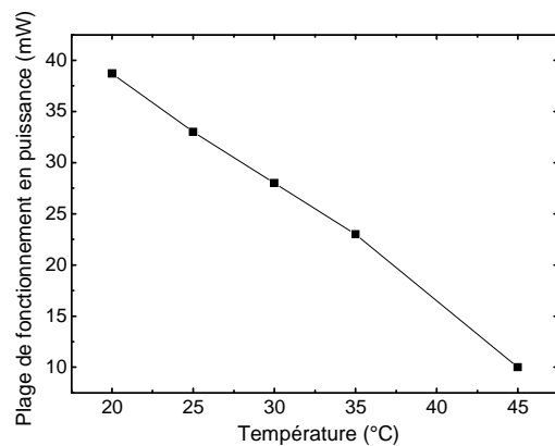
Figure III.27: Variation de la plage de fonctionnement en puissance du VCSEL hybride
