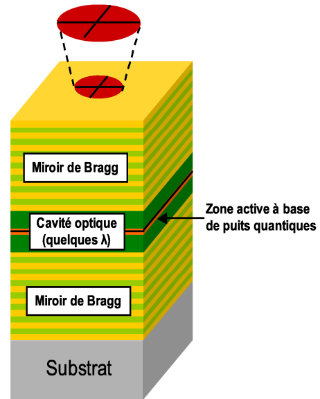
Figure I.2: Schéma d'un laser à semi-conducteurs à émission vertical
