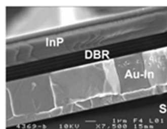
Figure II.30: Image MEB d'une demi-cavité reportée sur substrat de silicium[22]
