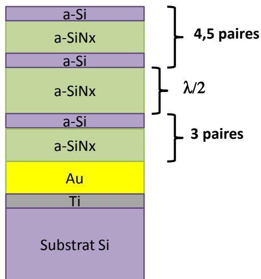
Figure III.19: Structure de la cavité froide employée. La couche de a-SiN x d'épaisseur \lambda/2 est réalisée selon le cas, soit en pulvérisation cathodique soit en PECVD.
