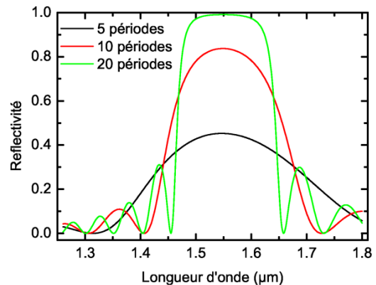
Figure I.5: réflectivité simulée d'un miroir de Bragg avec un \Delta n = 0,47 pour un nombre de périodes variable, un milieu incident et de sortie en GaAs.
