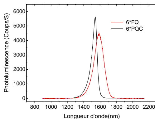
Figure II.45: Spectre de photoluminescence d'un échantillon de calibration comparé à celui des Puits quantique contraints
