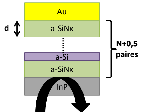
Figure III.18: Structure du miroir hybride composé d'un nombre impair de périodes
