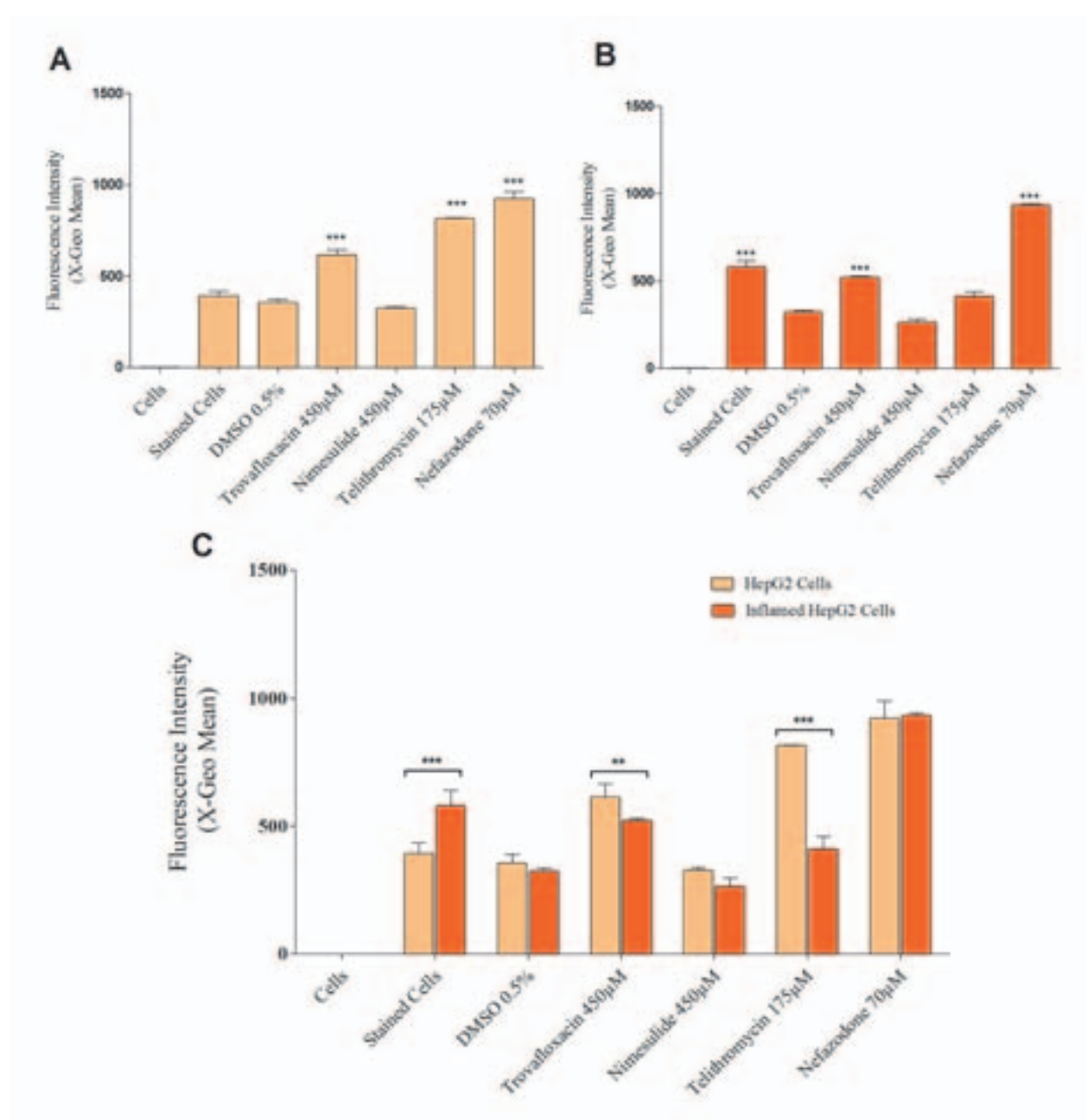
Figure 7.4. Effet stéatosique des quatre médicaments idiosyncrasiques sur cellules HepG2 non enflammées et enflammées. Les graphes représentent les effets stéatosiques des quatre médicaments testées après leur incubation dans les cellules HepG2 (A), en présence de LPS et de TNF- \alpha (B) et en absence et en présence de LPS et de TNF- \alpha pendant 24 heures (C). L'effet stéatosique est évalué en utilisant BODIPY 493/503 par cytométrie en flux. Les barres représentent la fluorescence intracellulaire accumulée de BODIPY 493/503. Les données sont représentées sous forme de moyenne \pm S.E.M (n = 3). L'analyse statistique est réalisée par test ANOVA suivi de Bonferroni post test. ** Et *** = P < 0,01 et P < 0,001 respectivement. Sur les graphes A et B, la valeur p représente la variation de l'effet stéatosique entre les cellules traitées et non-traitées (contrôle négatif). Sur le graphe C, la valeur p représente la variation de l'effet stéatosique entre les cellules HepG2 non-enflammées et enflammées.
