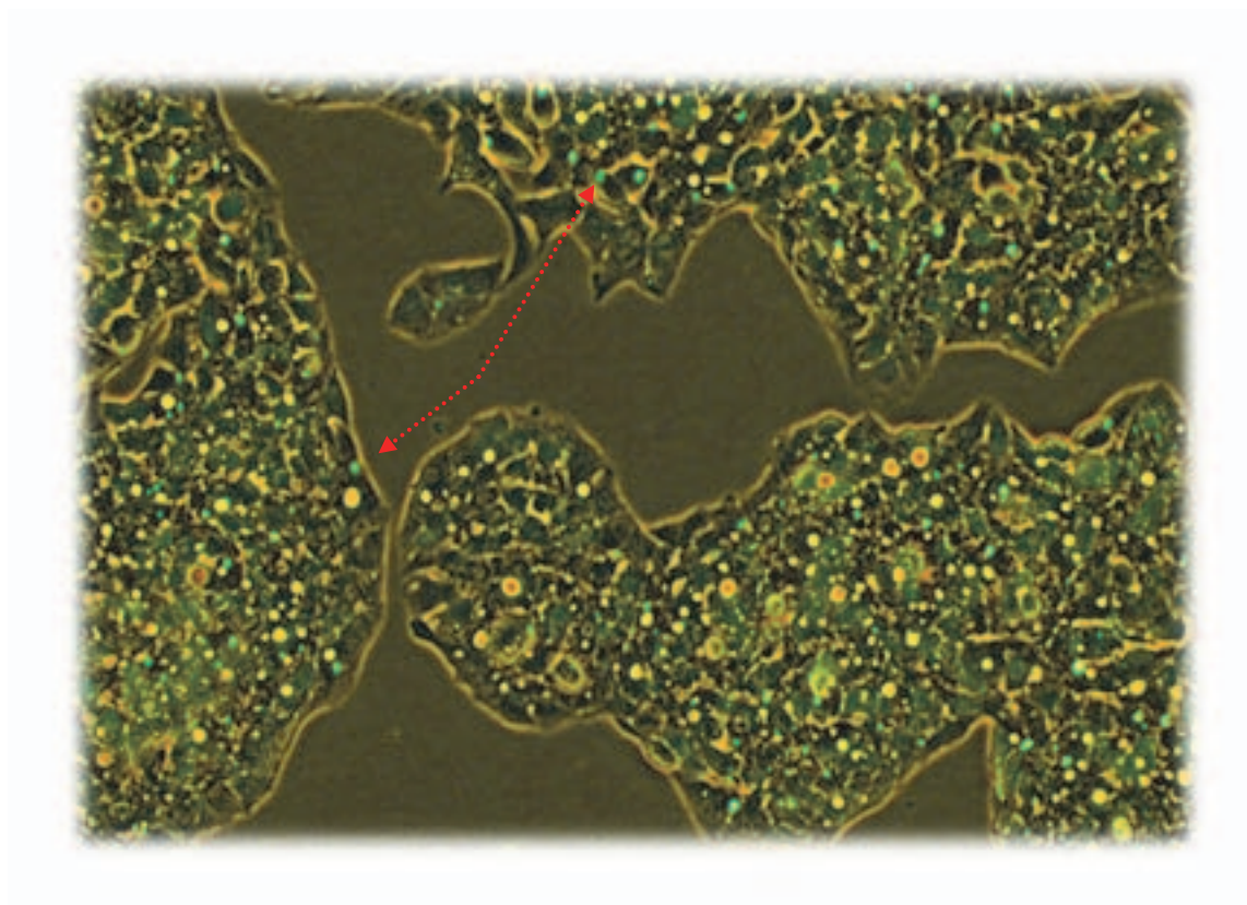
Figure 7.5. Localisation des pôles biliaires. Après incubation des cellules HepG2 avec du CDFDA, le diacetate de fluorescéine rendu fluorescent par estérification dans la cellule (CDF) est pris en charge par les transporteurs, et s'accumule aux pôles biliaires au niveau des canalicules si les pôles biliaires sont présents et fonctionnels. Les flèches rouges désignent ces pole biliaires (point vert brillant).
