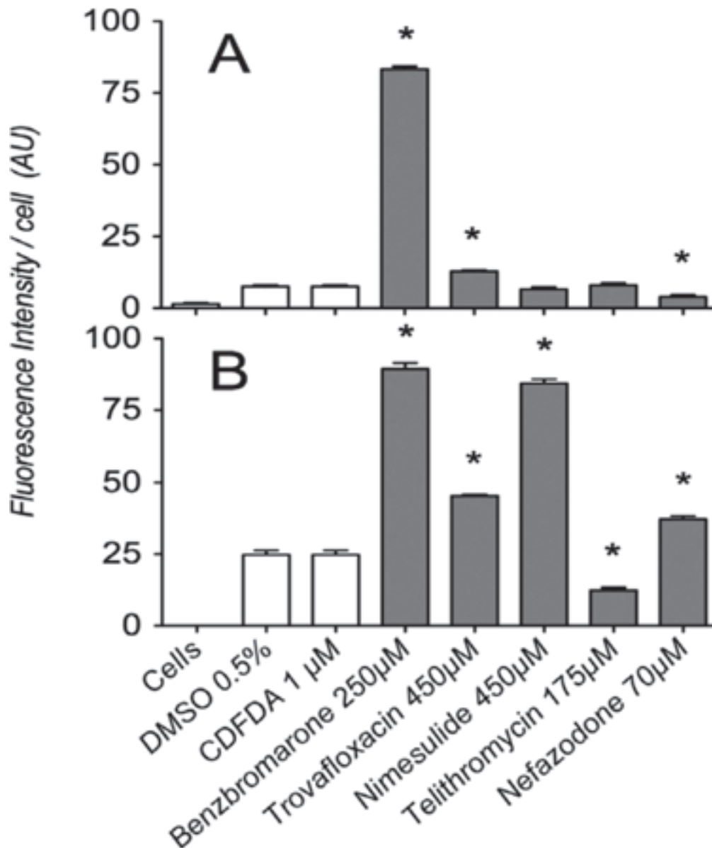
Figure 7.9. Effet des quatre médicaments idiosyncrasiques sur l'activité des transporteurs MRP2 dans les cellules HepG2 non enflammées et enflammées. Après incubation de cellules HepG2 avec les quatre médicaments idiosyncrasiques en absence (A) ou en présence (B) de LPS et de TNF- \alpha pendant 24 heures, l'activité des transporteurs MRP2 est évaluée à l'aide d'un test de transport fluorescent (CDF) par cytométrie en flux. Les barres représentent l'intensité de la fluorescence intracellulaire accumulée du CDF. Les données sont représentées sous forme de moyenne \pm S.E.M (n = 4). L'analyse statistique est réalisée à l'aide d'un test t non apparié.
