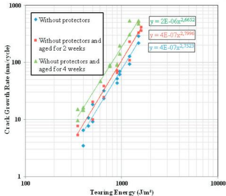
Figure 62 – Evolution de la vitesse de propagation de fissure en fonction du taux de restitution d'énergie d'un SBR réticulé au soufre et chargées, vieilli à 80°C sous air – Déterminée par traction cyclique d'éprouvette PS à 5Hz – Roche et al [6]
