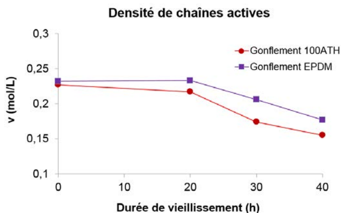
Figure 140 - Estimation de l'évolution de la densité de chaînes actives au cours du vieillissement, calculée à partir des mesures de gonflement du mélange 100 ATH (courbe rouge) et du mélange non chargé (courbe mauve)
