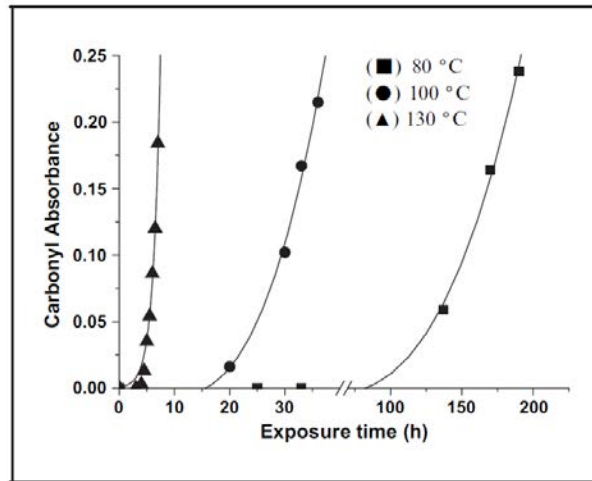
Figure 28 – Cinétique de formation des espèces carbonyles dans un film d'EPDM non chargé (100 μm d'épaisseur) – Kumar et al [3]
