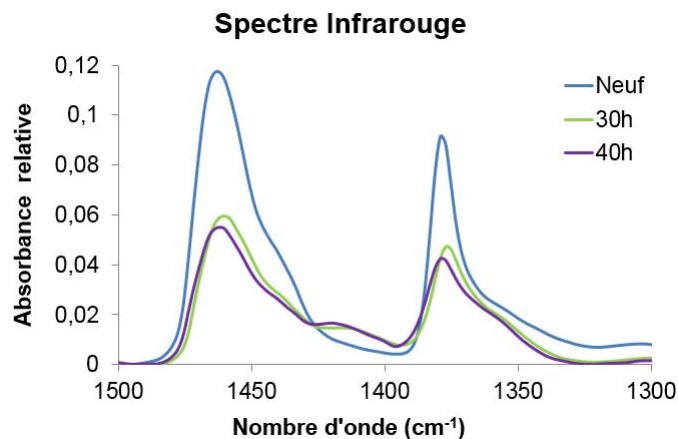
Figure 121 - Spectres infrarouge d'échantillon EPDM neuf et vieilli (mode ATR)
