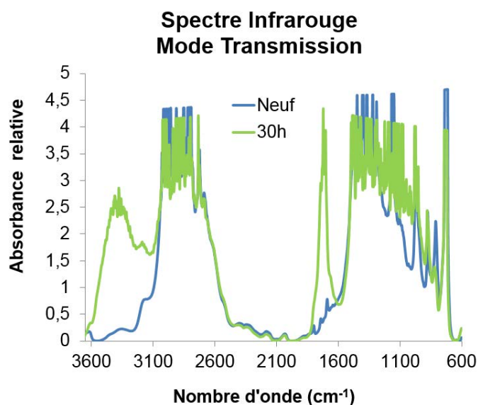
Figure 115 - Spectres infrarouge du mélange non chargé neuf et vieillis 30h – Mesures effectuées en transmission
