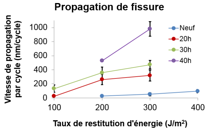
Figure 166 – Vitesse de propagation de fissure par cycle en fonction du taux de restitution d'énergie G du mélange 100 ATH – Epreuves PS sollicitées à 2Hz - Moyennes et écarts-types sur 5 mesures
