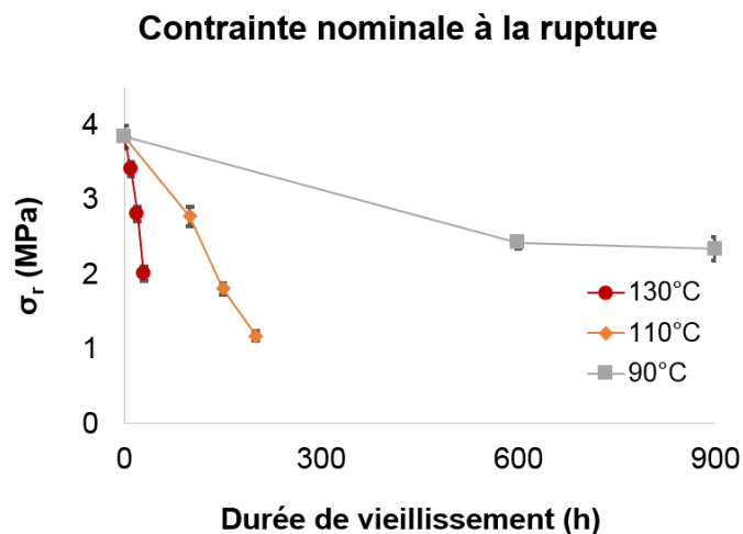
Figure 209 - Evolution en fonction de la durée de vieillissement de la contrainte nominale à la rupture du mélange 100 ATH vieillis à 130°C, 110°C et 90°C
