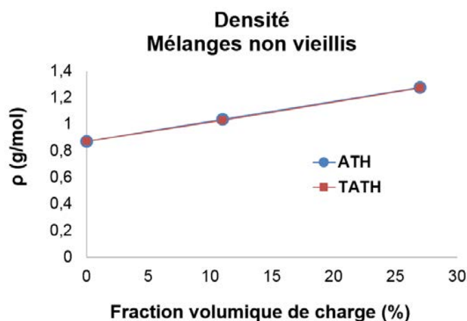
Figure 110 – Evolution, en fonction du taux de charges, de la densité – Courbe bleue : charges ATH – Courbe rouge : charges TATH - Valeurs moyennes déterminés à partir de 5 mesures
