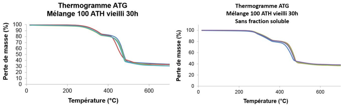
Figure 205 – Thermogramme ATG du mélange 100 ATH vieilli 30h – Echantillon avec fraction soluble (à gauche) – Echantillon sans fraction soluble (à droite)
