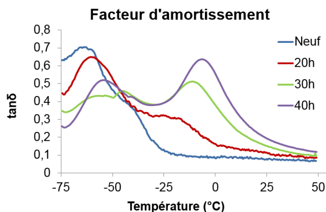
Figure 125 – Evolution du facteur d’amortissement en fonction de la température d’essai pour des échantillons neuf et vieillis
