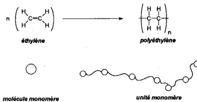
Figure 1 – Illustration de la notion de monomère [1]
