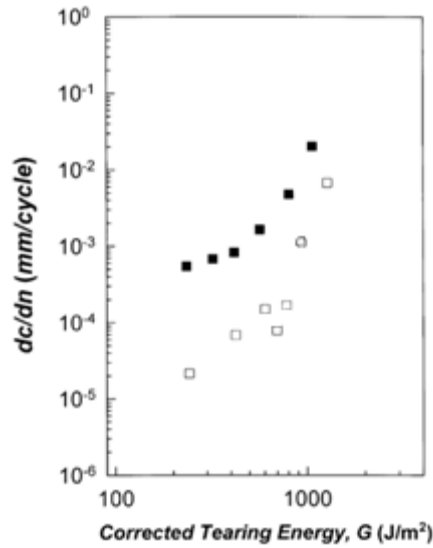
Figure 49 - Evolution de la vitesse de propagation de fissure en fonction du taux de restitution d'énergie d'un SBR non chargé – Eprouvettes PS ( e=1.8\text{mm} ) sollicitées à 10\text{mm}/\text{min} – Carrés vides : sec, Carrés noirs : gonflé – Cho et al [2]
