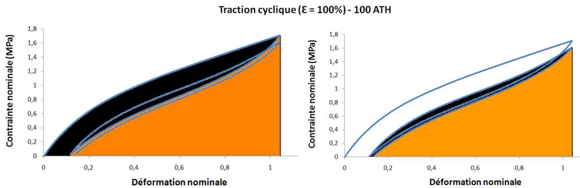
Figure 162 – Courbes contraintes-déformation en traction cyclique du mélange 100 ATH, composées de deux cycles à 100% de déformation – A gauche : hystérèse de Mullins en noir – A droite : hystérèse stabilisée en noir
