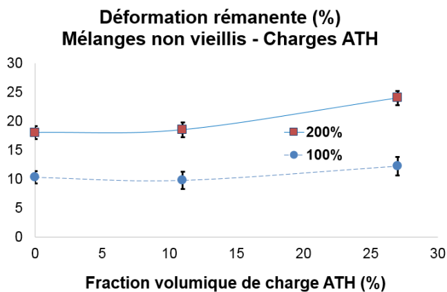
Figure 98 - Evolution, en fonction de la fraction de charges ATH, de la déformation rémanente après l'application d'une déformation de 100% (courbe bleue), et de 200% (courbe rouge) - Moyennes et écarts type déterminés à partir de 3 mesures
