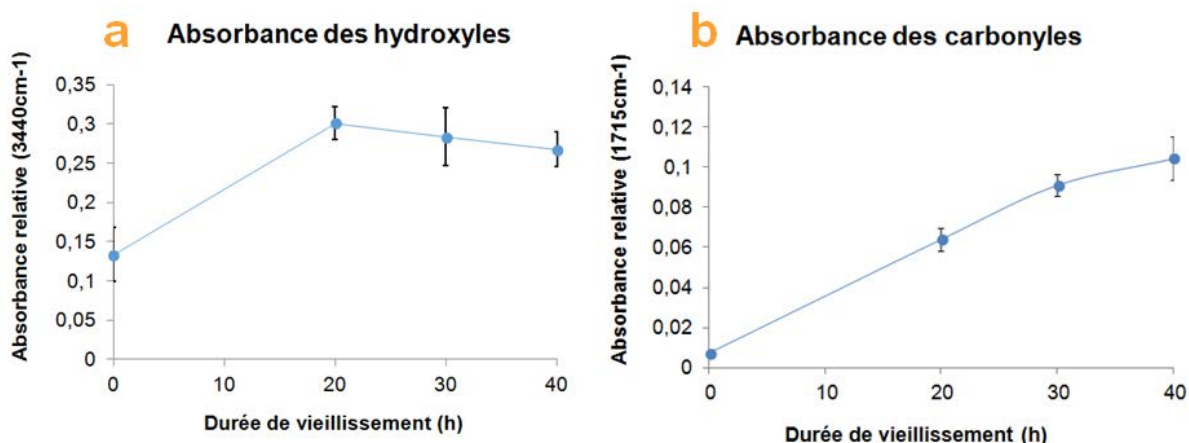
Figure 117 - a : Absorbance relative des hydroxyles ( 3440\text{ cm}^{-1} ) du mélange 100 ATH mesurée en mode ATR – b : Absorbance relative des carbonyles ( 1715\text{ cm}^{-1} ) du mélange 100 ATH mesurée en mode ATR
