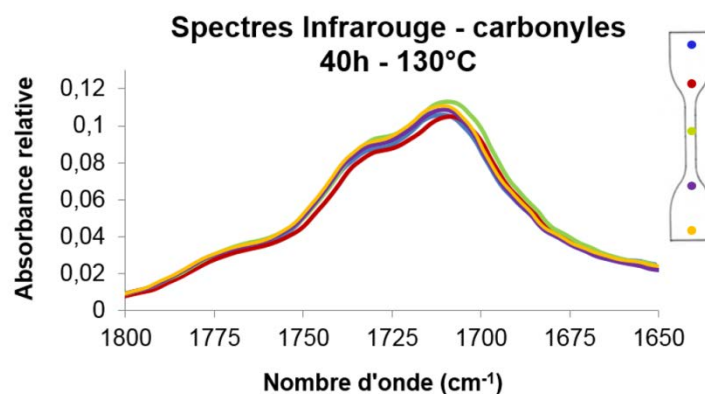
Figure 196 - Spectres infrarouge des espèces carbonyles mesurés en cinq zones superficielles d'une éprouvette de traction
