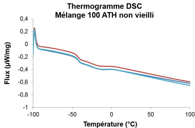
Figure 195 – Thermogramme DSC du mélange 100 ATH non vieilli
