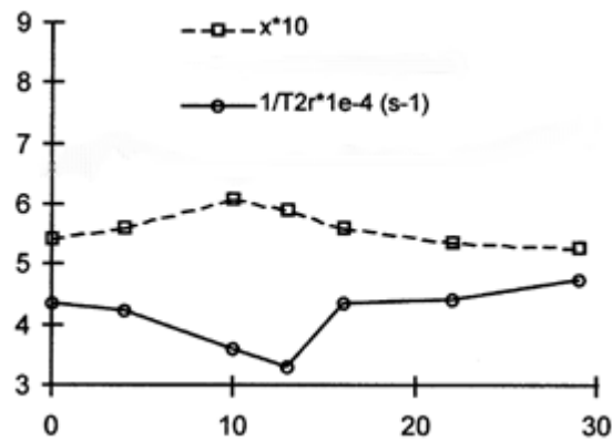
Figure 33 – Evolution de l'inverse du temps de relaxation ( T_2 ) et de x (paramètre représentatif de la mobilité du réseau) au cours du vieillissement d'un EPDM non chargé, vieilli 13 jours à 200°C puis 16 jours à 270°C en absence d'oxygène – Palmas et al [6]
