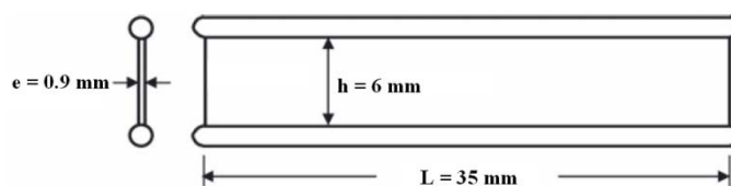
Figure 74 – Géométrie et dimensions des éprouvettes Pure-Shear (PS) - Image provenant de [33]
