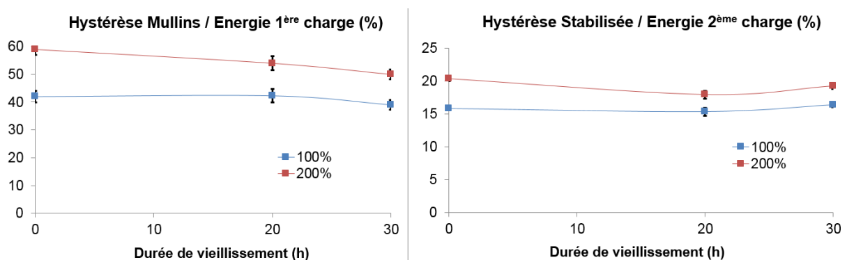
Figure 163 - Evolution au cours du vieillissement de la dissipation d'énergie du mélange 100 ATH obtenue par traction cyclique – A gauche : Rapport de l'hystérèse de Mullins sur l'énergie de première charge – A droite : Rapport de l'hystérèse de stabilisée sur l'énergie de la seconde charge - Moyennes et écarts-types sur 5 mesures
