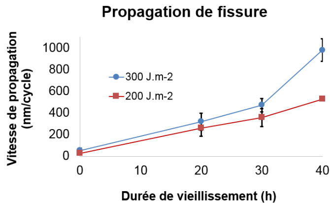
Figure 167 – Evolution au cours du vieillissement de la vitesse de propagation de fissure par cycle du mélange 100 ATH - Epreuves PS sollicitées à 2Hz – Courbe rouge : G = 200 J.m -2 – Courbe bleue : G = 300 J.m -2 - Moyennes et écarts-types sur 5 mesures
