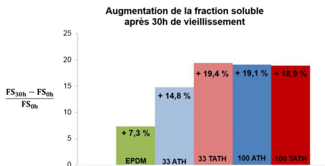
Figure 153 – Augmentation de la fraction soluble après 30h de vieillissement
