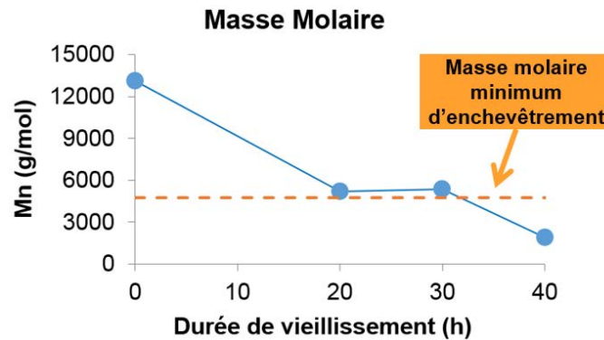
Figure 141 – Evolution au cours du vieillissement de la masse molaire en nombre (Mn) de la fraction soluble du mélange 100 ATH
