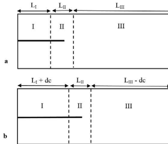
Figure 46 – Eprouvettes PS entaillée, avant propagation (schéma a) et après propagation (schéma b) de la fissure d'une longueur dc
