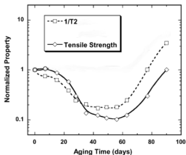
Figure 31 - Comparaison de l'inverse du temps de relaxation ( T_2 ) avec le module d'Young normalisé, en fonction de la durée de vieillissement d'un EPDM chargé vieilli à 140°C - Assink et al [7]
