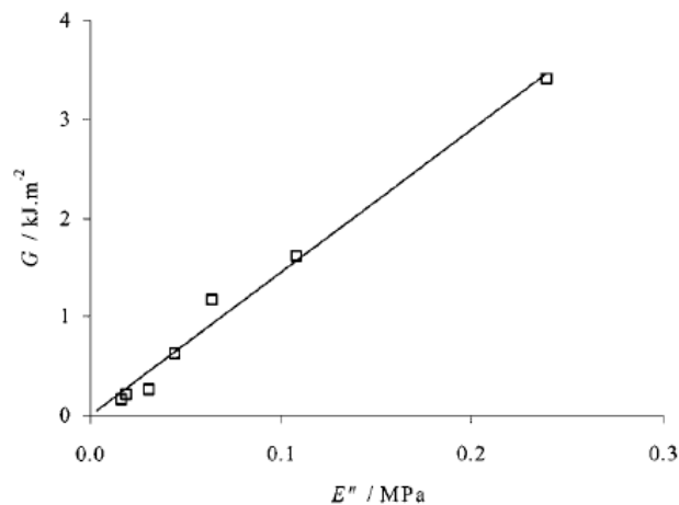
Figure 48 – Evolution du taux de restitution d'énergie critique G_c en fonction du module de perte d'un SBR (5phr oxyde de zinc) – Eprouvettes pantalon sollicitées à 7 \cdot 10^{-3} \text{s}^{-1} gonflées au Dibutyl adipate – Tsunoda et al [1]
