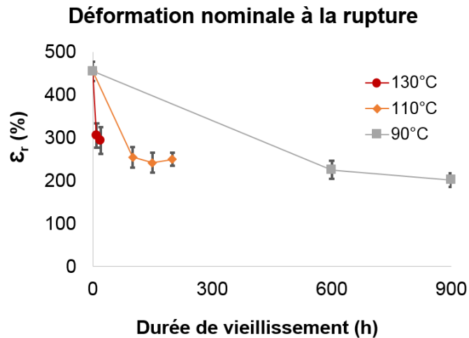
Figure 208 - Evolution en fonction de la durée de vieillissement de la déformation nominale à la rupture du mélange 100 ATH vieillis à 130°C, 110°C et 90°C
