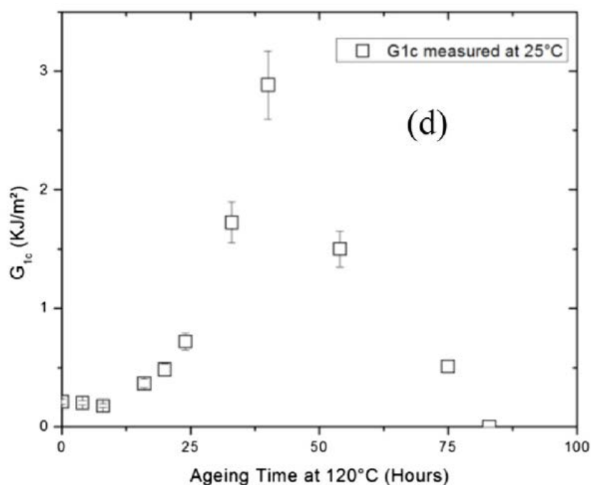
Figure 63 – Evolution du taux de restitution d'énergie critique en fonction de la durée de vieillissement pour un polybutadiène, réticulé au diisocyanate et non chargé, vieilli à 120°C – Déterminée par traction monotone d'éprouvettes lanières à double entailles - Le Gac et al [8]
