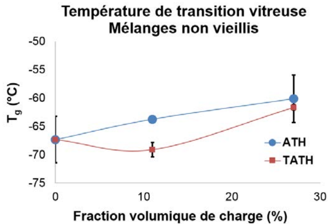
Figure 107 – Evolution, en fonction du taux de charges, de la température de transition vitreuse – Courbe bleue : charges ATH – Courbe rouge : charges TATH - Valeurs moyennes déterminés à partir de 3 mesures
