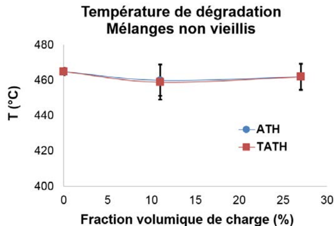
Figure 113 – Evolution, en fonction du taux de charges, de la température de dégradation – Courbe bleue : charges ATH – Courbe rouge : charges TATH - Valeurs moyennées déterminées à partir de 5 mesures
