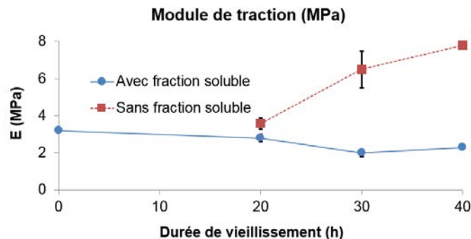
Figure 173 – Evolution du module de traction au cours du vieillissement d'échantillons avec fraction soluble (bleues) et sans fraction soluble (rouges) – Moyennes et écart-types sur 5 mesures
