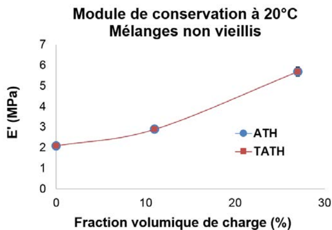
Figure 102 – Evolution, en fonction du taux de charges, du module de conservation à 20°C – Courbe bleue : charges ATH – Courbe rouge : charges TATH - Valeurs moyennes déterminés à partir de 3 mesures
