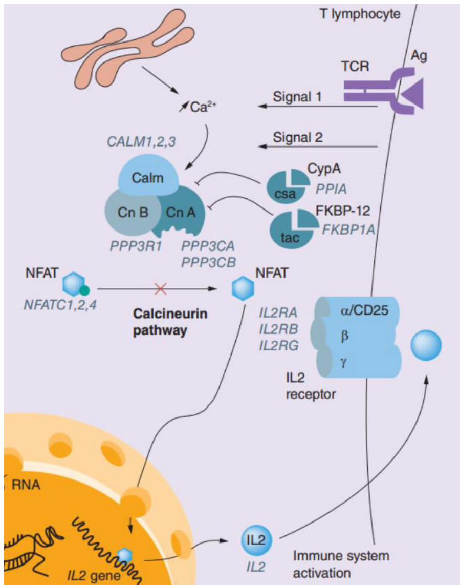
Figure 1. Voie de la calcineurine au sein du lymphocyte T (Ag : antigène ; Calm: Calmoduline; Cn A: Calcineurine A; Cn B: Calcineurine B; Csa: Ciclosporine; Cyp A: Cyclophiline A; NFAT: Nuclear factor activated T cell). L'état phosphorylé du facteur NFAT est indiqué par un cercle vert (7).
