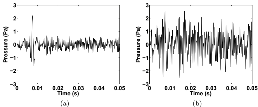
FIGURE 3.17 – Exemples de signaux mesurés sur un microphone de l'antenne double-couche pour deux valeurs différentes de rapport signal à bruit. (a) \sigma = 5 dB ; (b) \sigma = -5 dB
