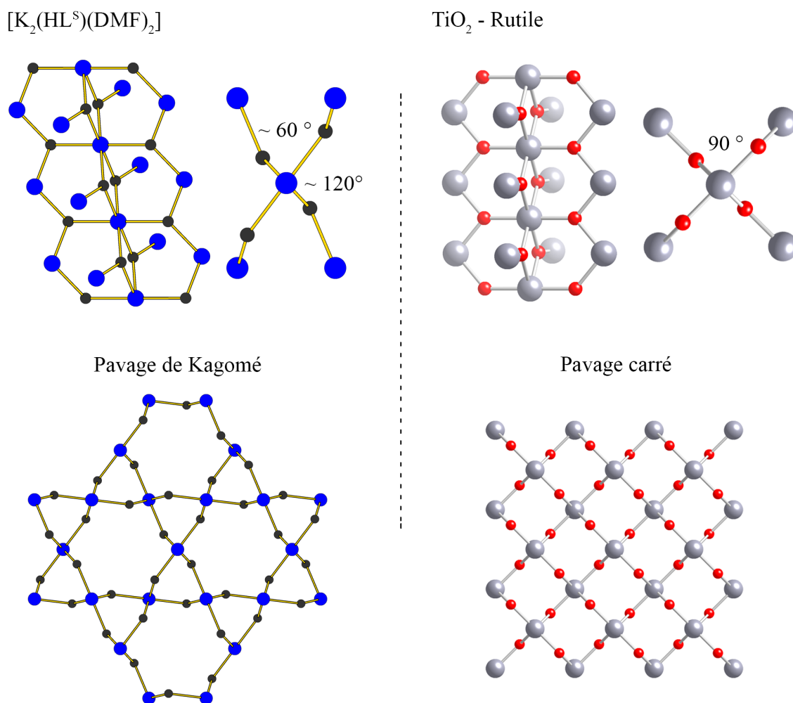
Figure 20. Comparaison des structures de [K_2(L^S)(DMF)_2] et du rutile le long de l'axe c (haut) et différenciation du pavage de ces deux structures dans le plan ab (bas). Atomes : Ti (gris) ; O (rouge). Nœuds : hexavalent (bleu) ; trivalent (noir).
