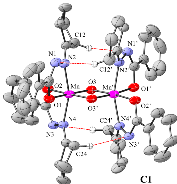
Figure 23. Vue ORTEP de C1 avec numérotation partielle des atomes. Les atomes d'hydrogène ne sont pas inclus par soucis de clarté à l'exception les atomes d'hydrogène représentés par de petites sphères participants aux interactions CH-X (pointillés rouges). Les ellipsoïdes contiennent 50 % de la densité électronique.
