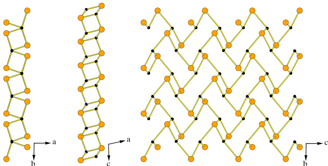
Figure 40. Structure simplifiée de BaL^S . Nœuds : Ba (jaune) ; ligand (noir).
