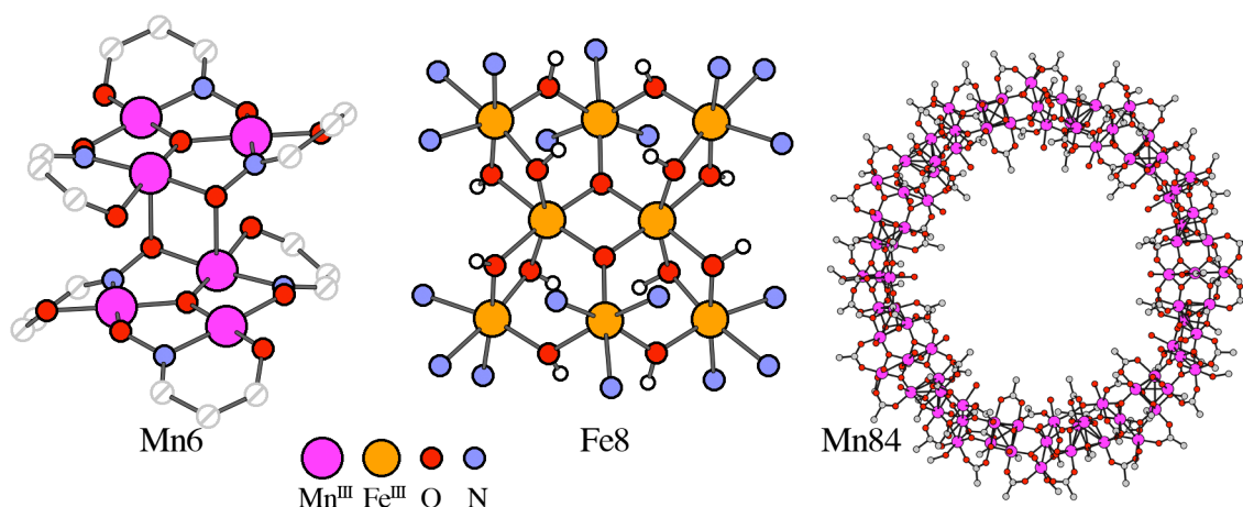
Figure 4. Complexe hexanucléaire de Mn (III), complexe octanucléaire de Fe (III) et complexe de 84 Mn (III) d'après réf. 14-16.
