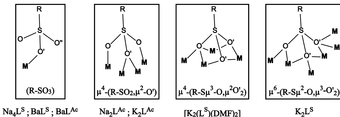
Figure 51. Modes de coordination du sulfonate dans les complexes étudiés.
