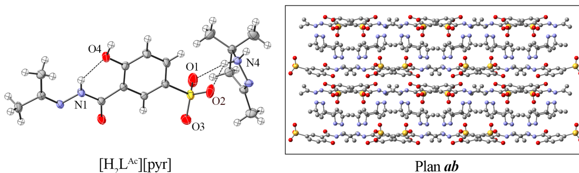
Figure 25. Vue ORTEP du sel [L Ac ][pyr] (gauche) et arrangement par couche de la structure (droite). Les liaisons hydrogène intramoléculaires sont représentées par des pointillées noires. Les ellipsoïdes contiennent 50 % de la densité électronique.
