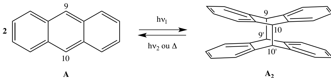
Figure 3. Photodimérisation « classique » de l'anthracène (A), la dissociation du photodimère (A 2 ) par un processus thermique ou photochimique permet de revenir à l'anthracène. Cette réaction se déroule également pour de nombreux dérivés substitués de l'anthracène.
