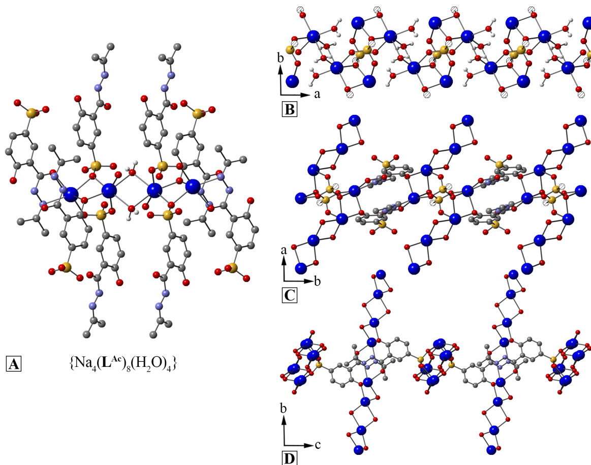
Figure 42. Structure du complexe tétranucléaire \{Na_4(L^{Ac})_8(H_2O)_4\} (gauche) et réseaux formés le long des axes a , b et c entre ces complexes (droite). Par soucis de clarté certains atomes ne participant pas à la formation des réseaux ne sont pas inclus, dans certains cas seul la fonction pontante du ligand est affichée et le reste de la molécule est symbolisée par une sphère hachurée.
