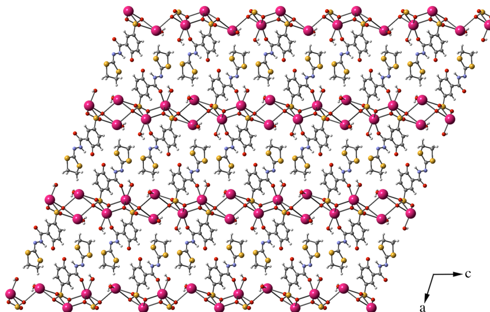
Figure 36. Packing de K_2L^S sur le plan ac . Atomes : K (rose) ; S (jaune) ; O (rouge) ; N (bleu) ; C (gris) ; H (blanc).
