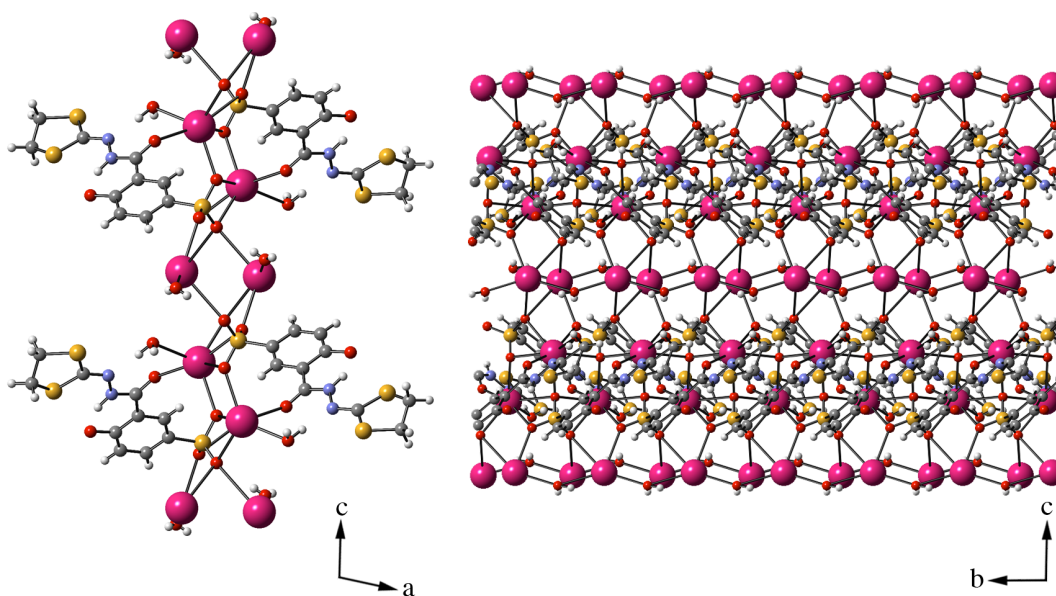
Figure 35. Réseau de coordination 2-D de K_2L^S dans les plans ac et bc . Atomes : K (rose) ; S (jaune) ; O (rouge) ; N (bleu) ; C (gris) ; H (blanc).
