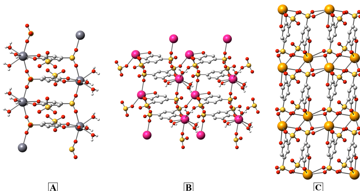
Figure 13. Structures 1, 2 et 3-D des complexes de calcium (A), strontium (B) et baryum (C) du ligand 4,5-dihydroxybenzene-1,3-disulfonate. A l'exception des molécules de H 2 O, les atomes d'hydrogène ne sont pas représentés par soucis de clarté. Atomes : Ca (gris) ; Sr (rose) ; Ba (jaune) ; S (jaune) ; O (rouge) ; C (gris).
