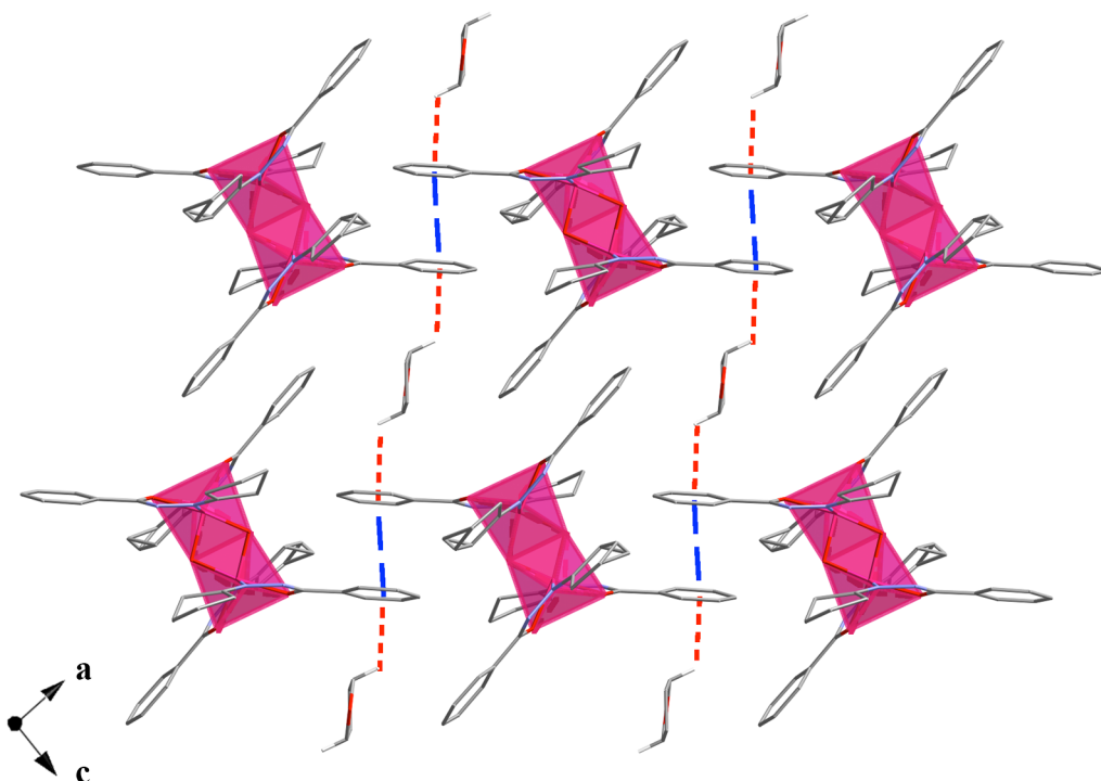
Figure 24. Packing cristallin de C1 , réseau d'interactions \pi - \pi (pointillés bleu) et CH- \pi (pointillés rouge).
