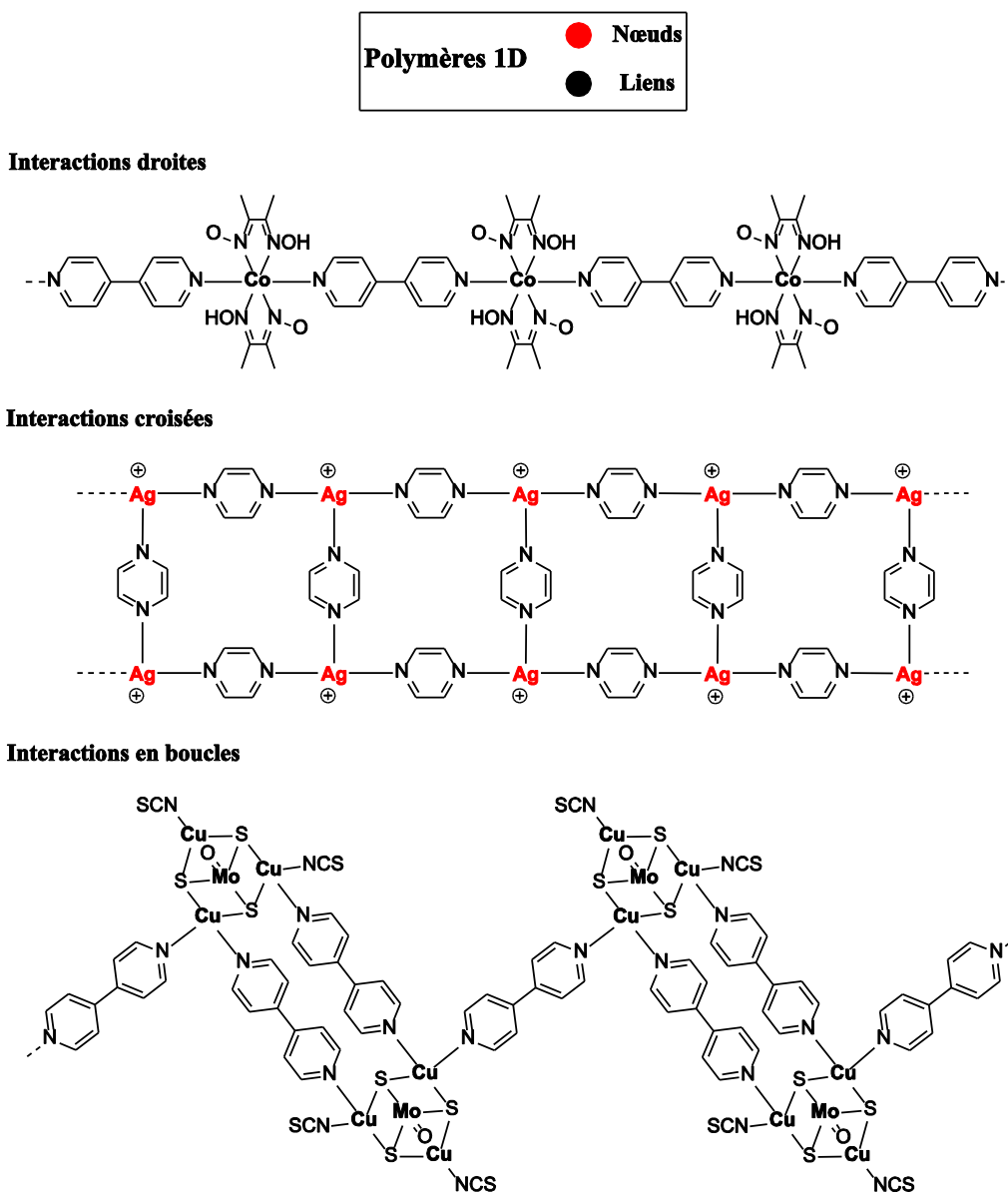
Figure 2. Réseaux 1-D montrant différentes connectivités. 3
