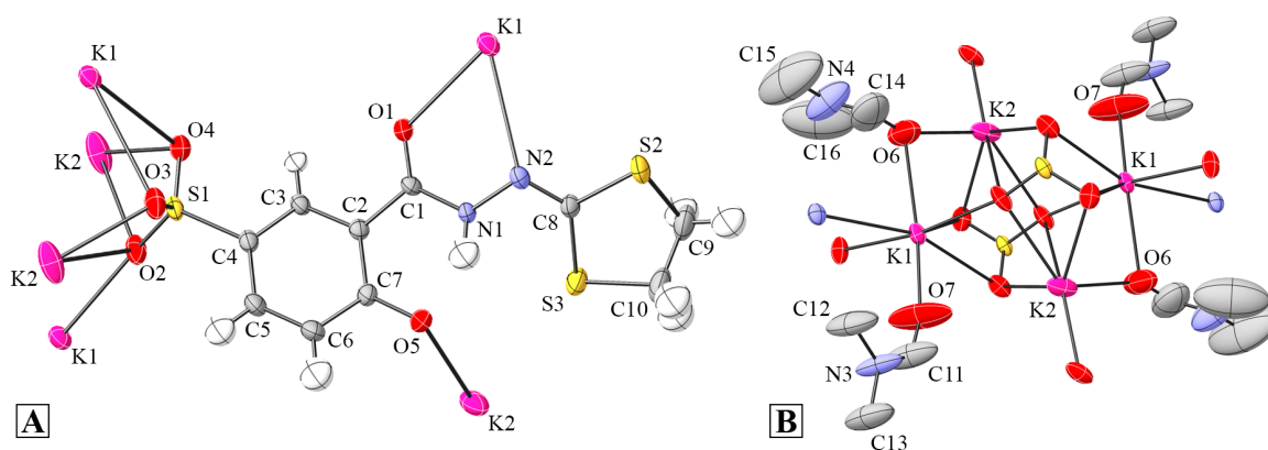
Figure 17. Vue ORTEP de la complexation d'un ligand (A) et du complexe tétranucléaire de potassium (B) avec numérotation partielle des atomes. Les ellipsoïdes contiennent 50 % de la densité électronique.
