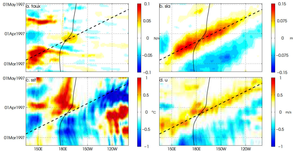
FIGURE I.22 – Anomalies intrasaisonnières associées au coup de vent de mars 1997 moyennées dans la bande 2^{\circ}\text{N} - 2^{\circ}\text{S} : (a) tension de vent zonale, (b) niveau de la mer, (c) SST, (d) courant de surface zonal. Sur chaque panneau, la ligne pleine représente le bord est du réservoir d’eau chaude. La ligne tiretée indique la trajectoire théorique de l’onde de Kelvin (d’après Drushka et al., 2015 ).
