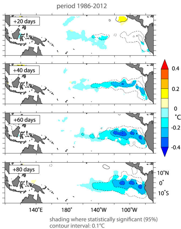
FIGURE I.25 – Composite des anomalies de SST les mois suivant l'occurrence d'un coup de vent d'est pendant la période 1986-2012. La couleur représente les valeurs significatives à 95% (d'après Chiodi et Harrison, 2015).
