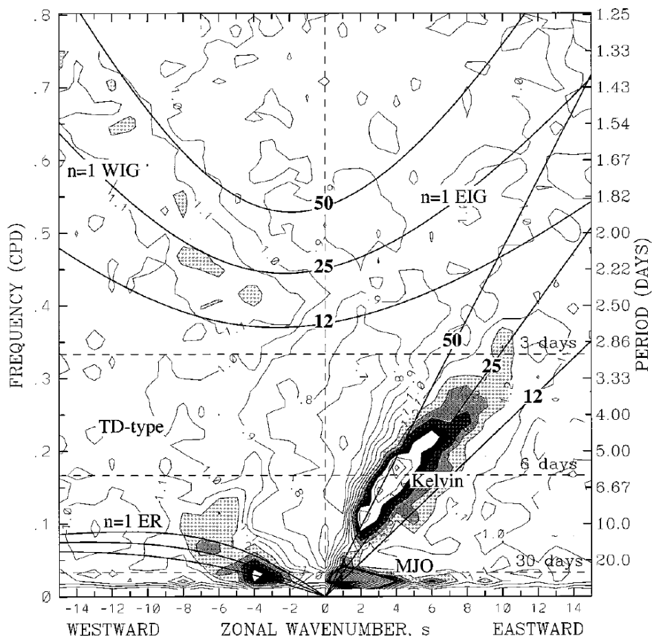
FIGURE I.18 – Les contours montrent le spectre en fréquence (axe des ordonnées) et nombre d'ondes zonales (axe des abscisses) du champ d'OLR symétrique divisé par le « spectre de fond ». L'intervalle des contours de ce ratio est 0.1, avec tous les contours inférieurs à 1.1 supprimés (d'après Wheeler et Kiladis, 1999 ).
