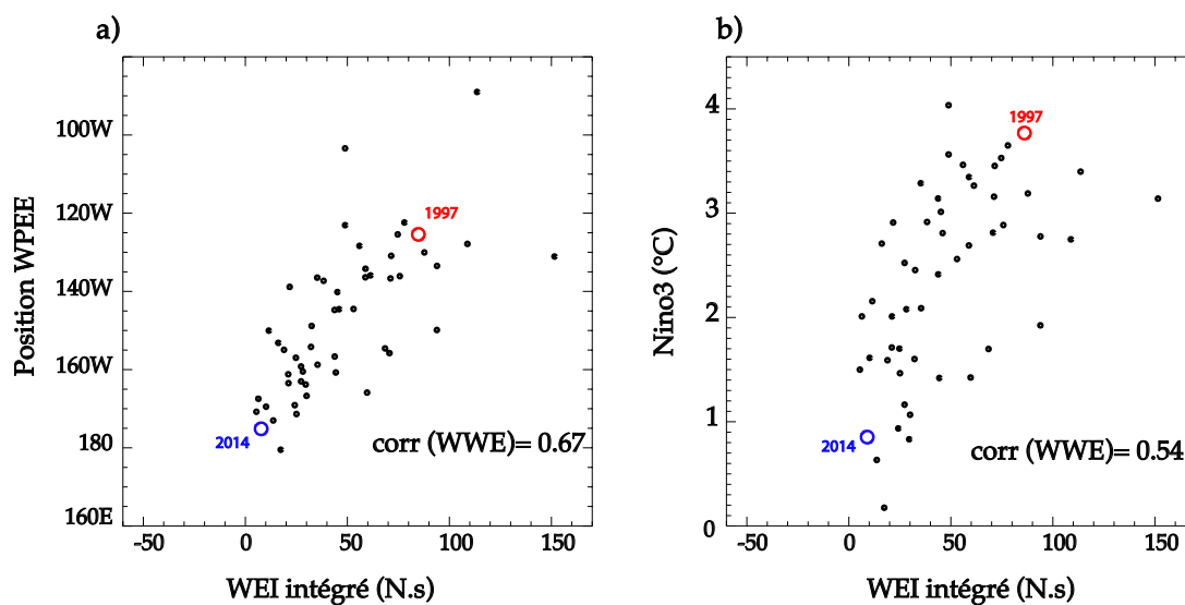
FIGURE V.19 – Scatterplot entre la somme des WEI des WWEs entre juin et octobre 2154 et (a) la position du WPEE et (b) l’amplitude des anomalies de SST dans la région Niño3 en Décembre 2154 pour chacun des membres de la simulation d’ensemble. Le point rouge (resp. bleu) représente l’année 1997 (resp. 2014) dans les observations
