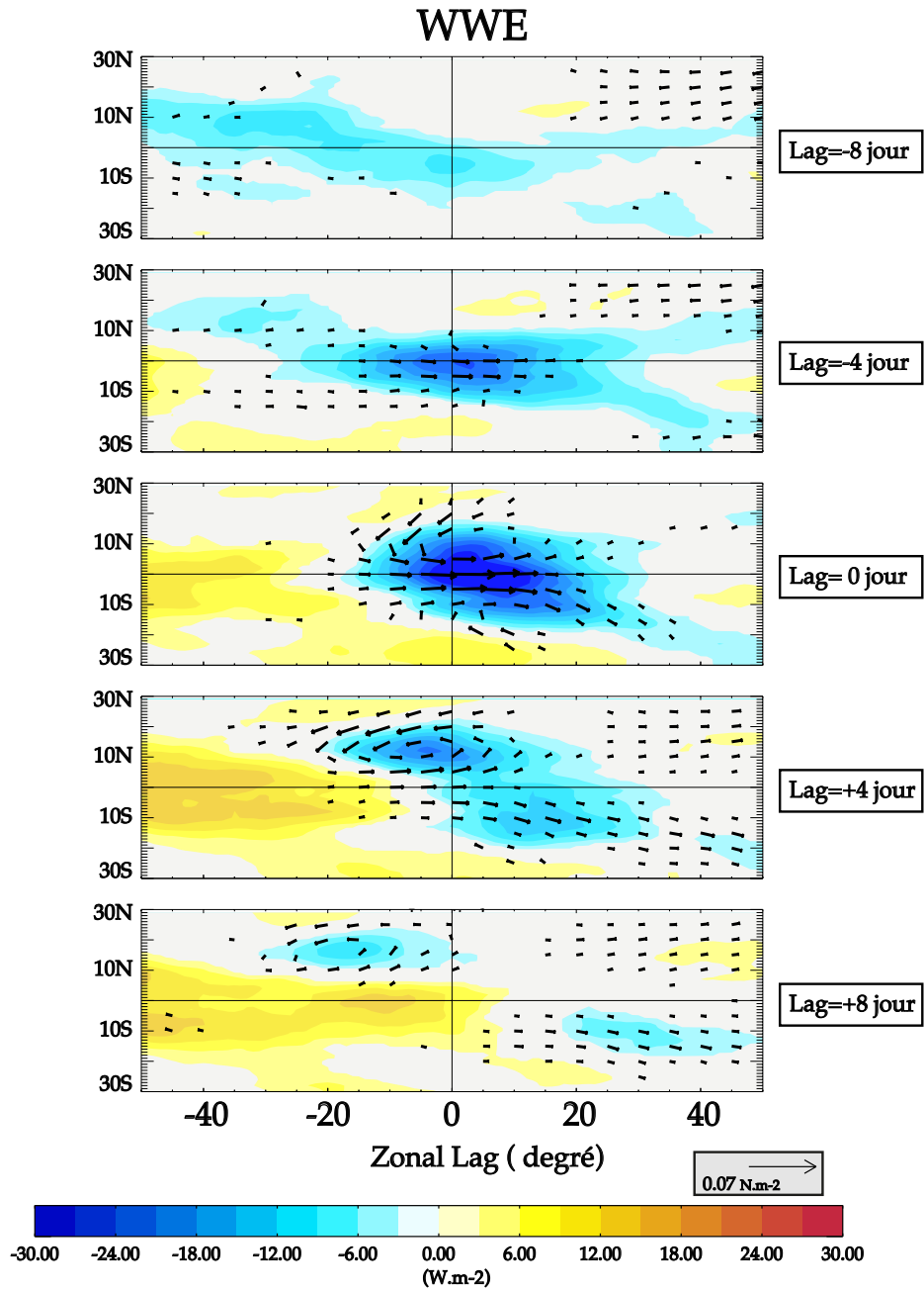
FIGURE I.16 – Composite spatial des anomalies intrasaisonnieres de tension de vent (vecteur) et OLR (couleur) 8 jours avant jusqu'à 8 jours après un WWE. Les composites sont centrés à la longitude et la date du WWE.
