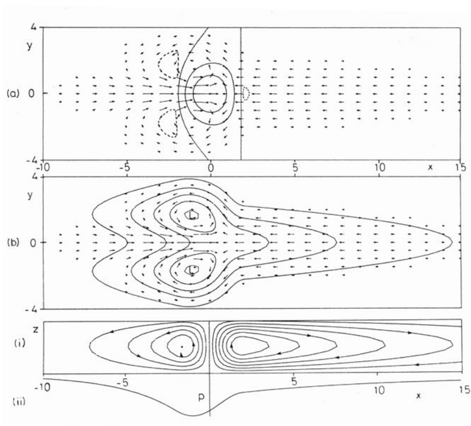
FIGURE I.11 – Réponse de l’atmosphère à un chauffage équatorial dans la région |x| < 2 : Anomalies de (a) Vitesse verticale w (trait continu correspondent à des vitesses de 0, 0.3, 0.6, et tireté à -0.1) et (b) de pression de surface (intervalle de 0.3 hPa) superposée au champ de vent de basses couches. (c) Lignes de courant à l’équateur illustrant la cellule de Walker et anomalie de pression surface (d’après Gill, 1980).
