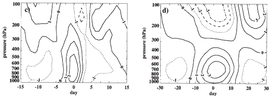
FIGURE I.17 – Composite de l'évolution temporelle de la structure spatiale des anomalies intrasaisonnières de vent zonal pendant un WWE court (a) et un WWE soutenu (b). Ces composites sont basés sur les réanalyses de vent ECMWF. Les lignes pointillées et tiretées représentent des vents d'est et les traits pleins, des vents d'ouest (d'après Fasullo et Webster, 2000 ).
