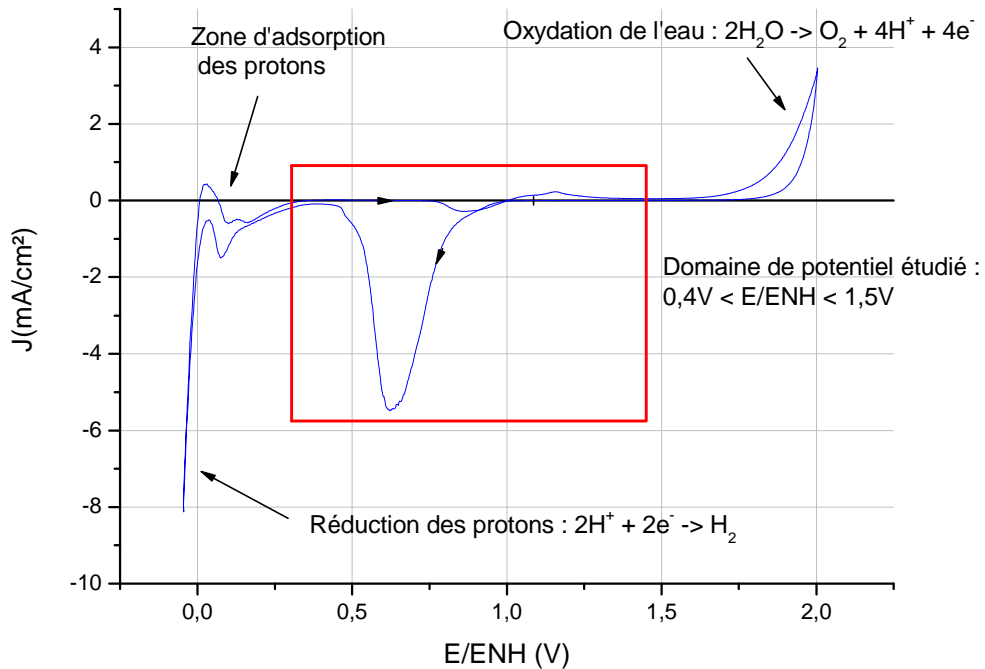
Figure 3.3 : Domaine d'électroactivité d'une solution de \text{HNO}_3 4 \text{ mol.L}^{-1} , électrode de Pt, vitesse de balayage v = 20 \text{ mV.s}^{-1} , T = 40^\circ\text{C}
