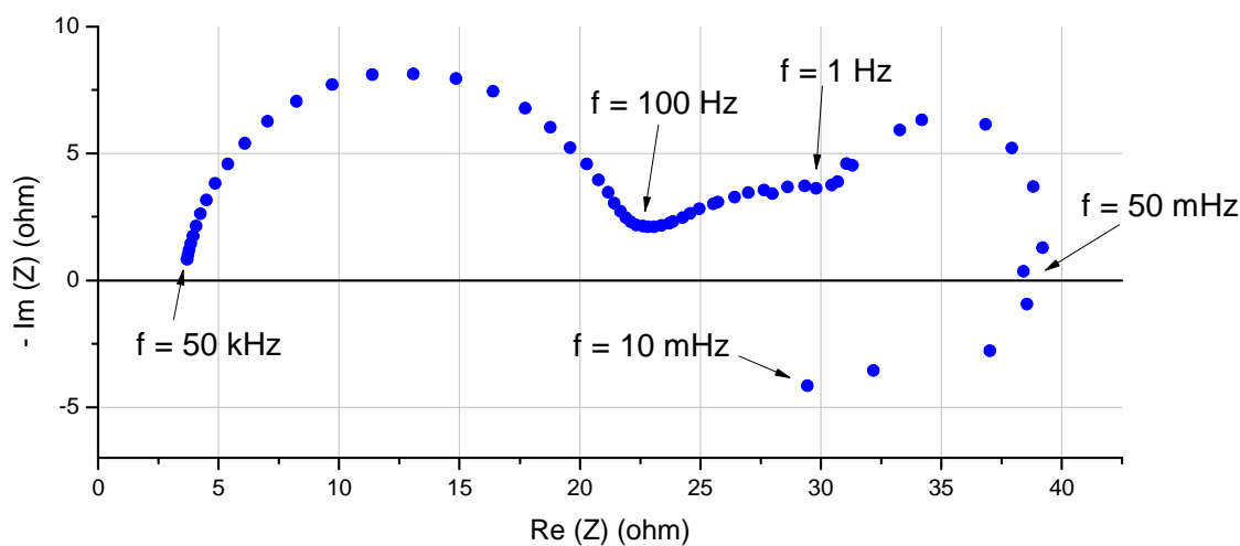
Figure 3.27 : Diagramme d'impédance dans le plan de Nyquist, E = 0,55 \text{ V/ENH} , \Delta E = 50 \text{ mV} , disque d'or tournant à 50 rpm, solution de \text{HNO}_3 \text{ } 4 \text{ mol.L}^{-1} , T = 40^\circ\text{C}
