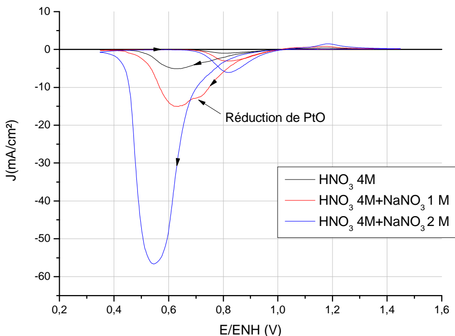
Figure 3.7 : Influence de l'ajout de nitrates sur la réduction de \text{HNO}_3 , électrode de Pt, v = 20\text{mV}\cdot\text{s}^{-1} , T = 40^\circ\text{C}
