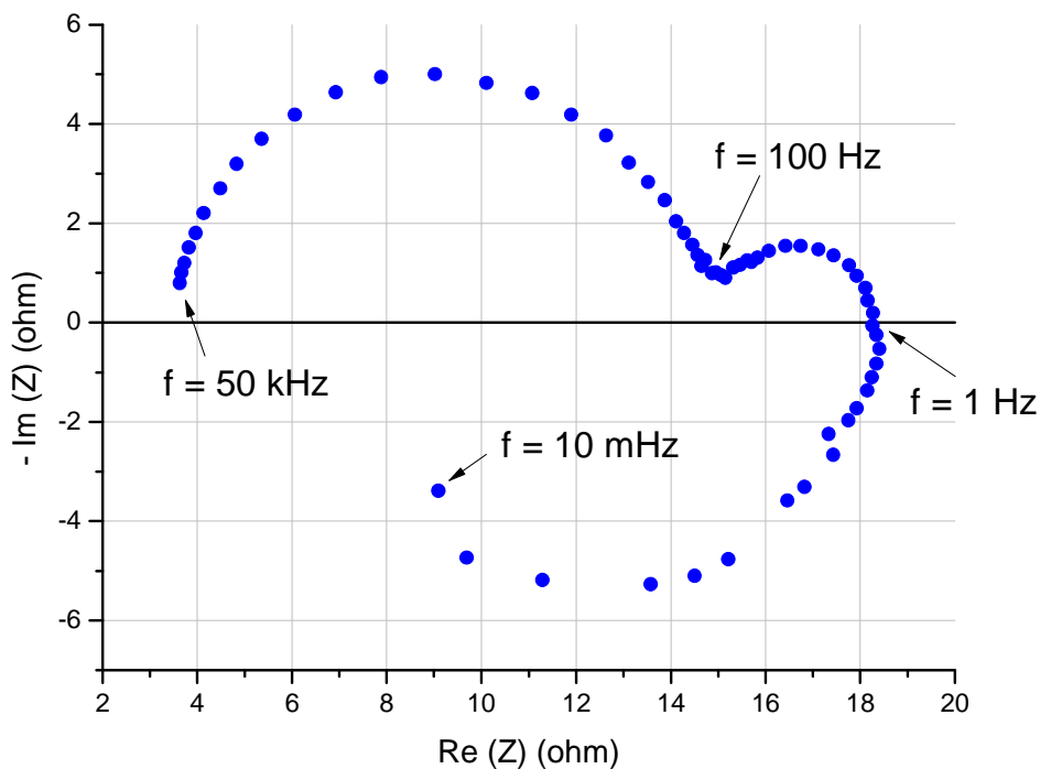
Figure 3.26 : Diagramme d'impédance dans le plan de Nyquist, E = 0,8 \text{ V/ENH} , \Delta E = 5 \text{ mV} , disque d'or tournant à 50 rpm, solution de \text{HNO}_3 \text{ } 4 \text{ mol.L}^{-1} , T = 40^\circ\text{C}
