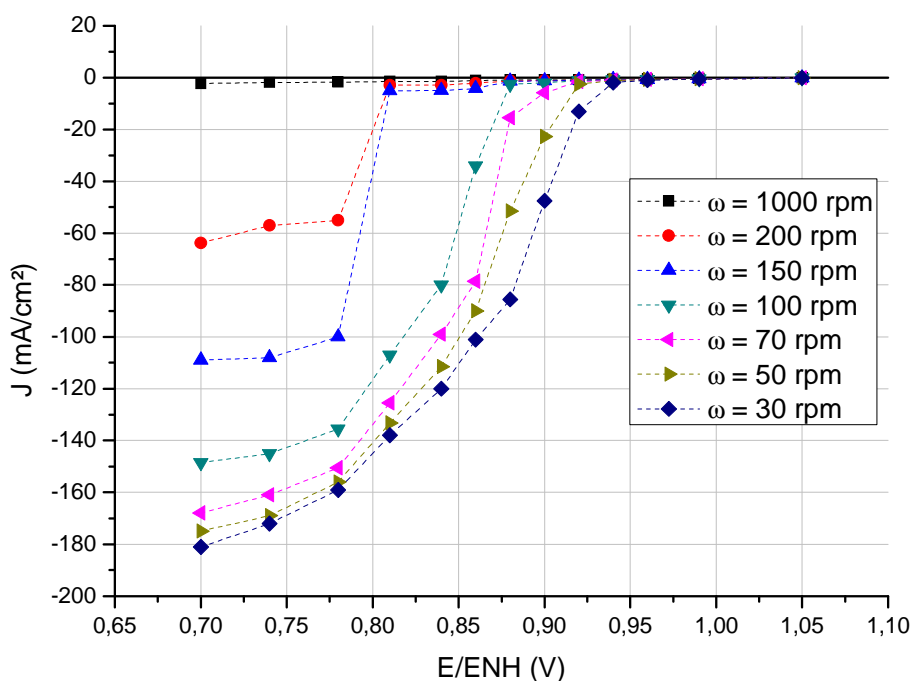
Figure 3.13 : Représentation du courant stationnaire en fonction du potentiel et influence de la vitesse de rotation de l'électrode, disque d'or tournant, solution de \text{HNO}_3 4 \text{ mol.L}^{-1} + \text{NaNO}_2 10^{-3} \text{ mol.L}^{-1} , T = 40^\circ\text{C}
