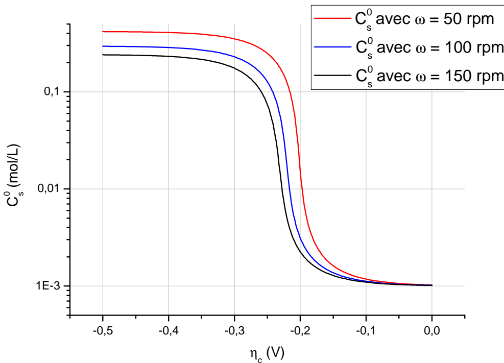
Figure 4.9 : Evolution de la concentration interfaciale stationnaire de \text{HNO}_2 C_s^0 en fonction de la surtension cathodique, selon l'équation 4.32
