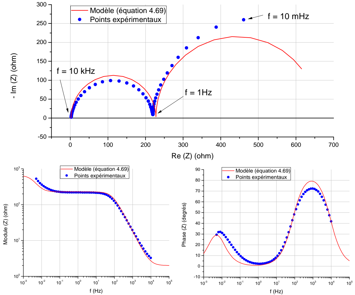
Figure 4.15 : Représentation de l'impédance pour une polarisation correspondant à la première zone de potentiels. Modèle : équation 4.69. Expérience : Impédance sur disque d'or tournant à 50 rpm, E = 1 \text{ V/ENH} , \Delta E = 10 \text{ mV} , solution de \text{HNO}_3 4 \text{ mol.L}^{-1} , T = 40^\circ\text{C}
