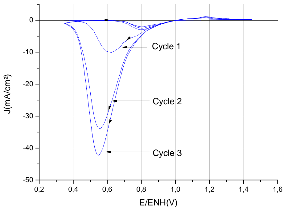
Figure 3.11 : Etude de cycles successifs lors d'essais de voltammétrie cyclique, électrode de Pt, solution de HNO 3 4 mol.L -1 , v = 20 \text{ mV.s}^{-1} , T = 40^\circ\text{C}
