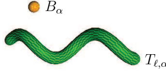
FIGURE 2.1.1 – Décomposition de g
