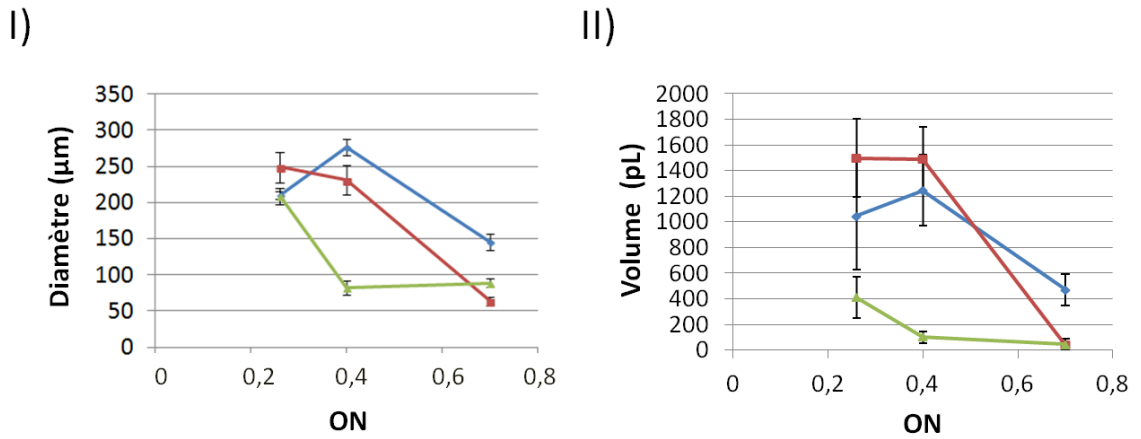
Figure 54 : Pour une énergie de 10 \mu\text{J} et une distance donneur-receveur de h_{\text{max}} : I) Diamètres des gouttes imprimées en fonction de l'Ouverture Numérique (ON) et de la bioencre (données extraites de [12]). II) Volumes des gouttes imprimées en fonction de l'Ouverture Numérique (ON) et de la bioencre.
