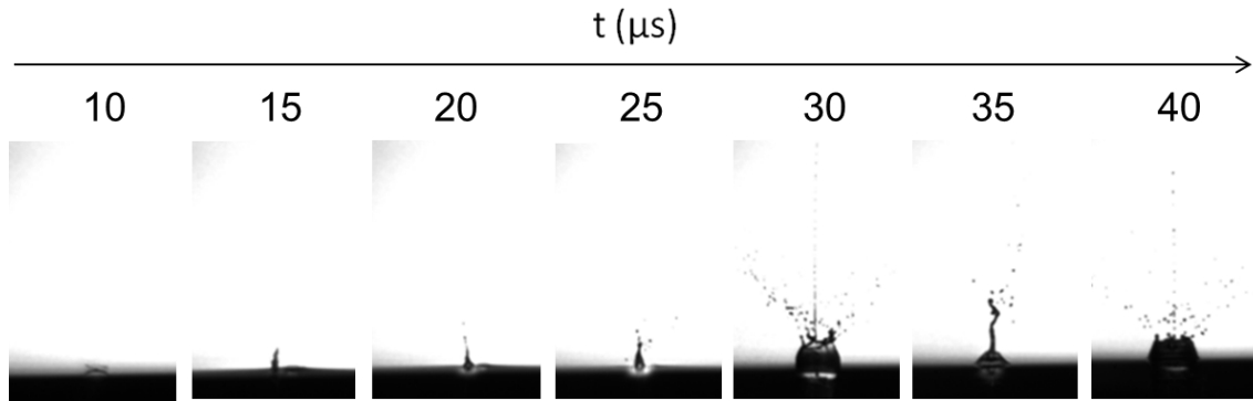
Figure 65 : Jet d'un train de 2 impulsions laser (appelé « mode burst » laser). Conditions expérimentales : bioencres A ; 30 \mu\text{m} d'épaisseur de bioencres ; 6 \mu\text{J} ; 1,4 ps de durée d'impulsion ; 200 kHz.
