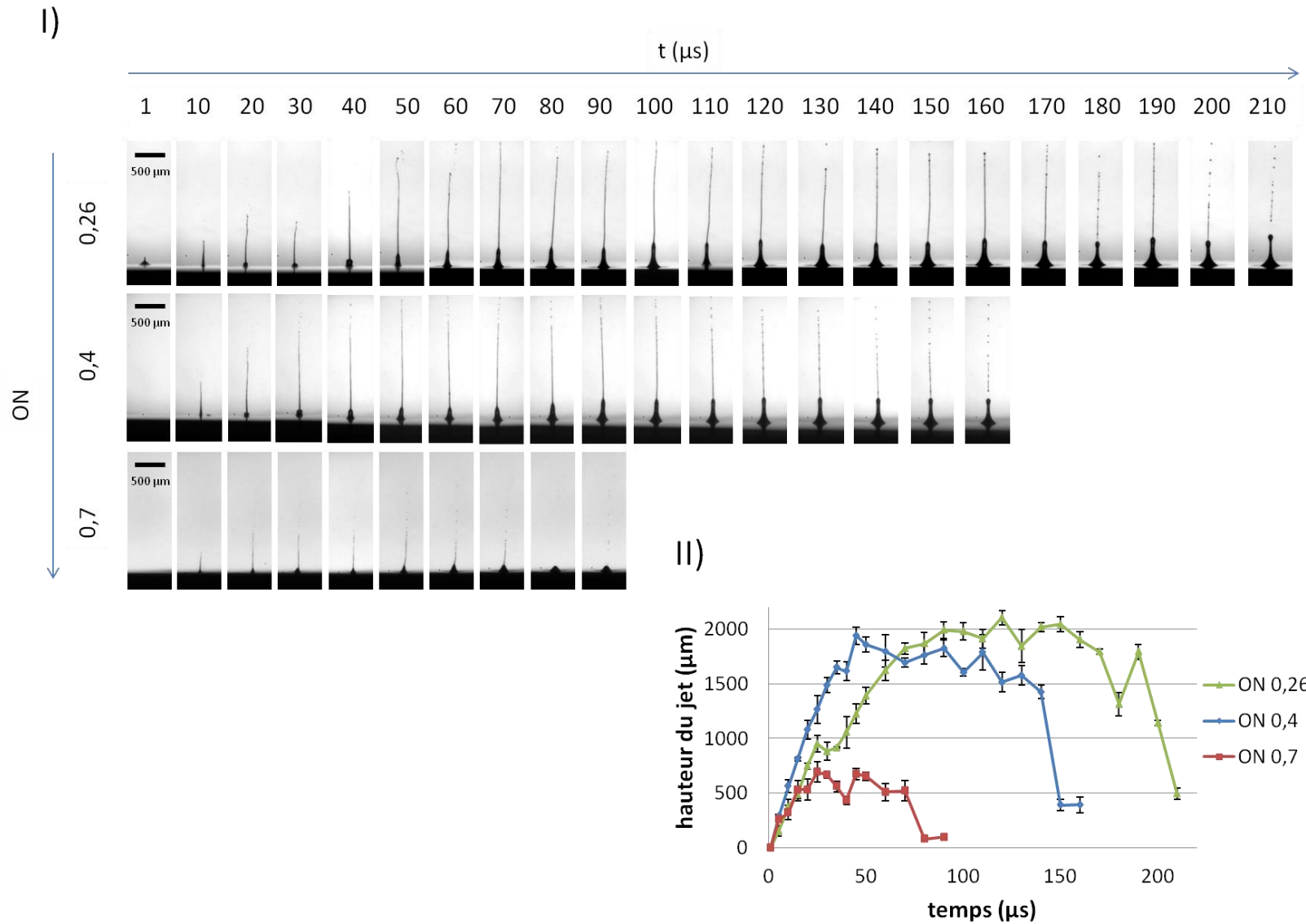
Figure 49: I) Images résolues en temps de l'évolution temporelle du jet induit par laser à 10 \mu\text{J} pour la bioencre E et une Ouverture Numérique (ON) de 0,26 à 0,7. II) Hauteur du jet mesurée sur les images de I) en fonction du temps.
