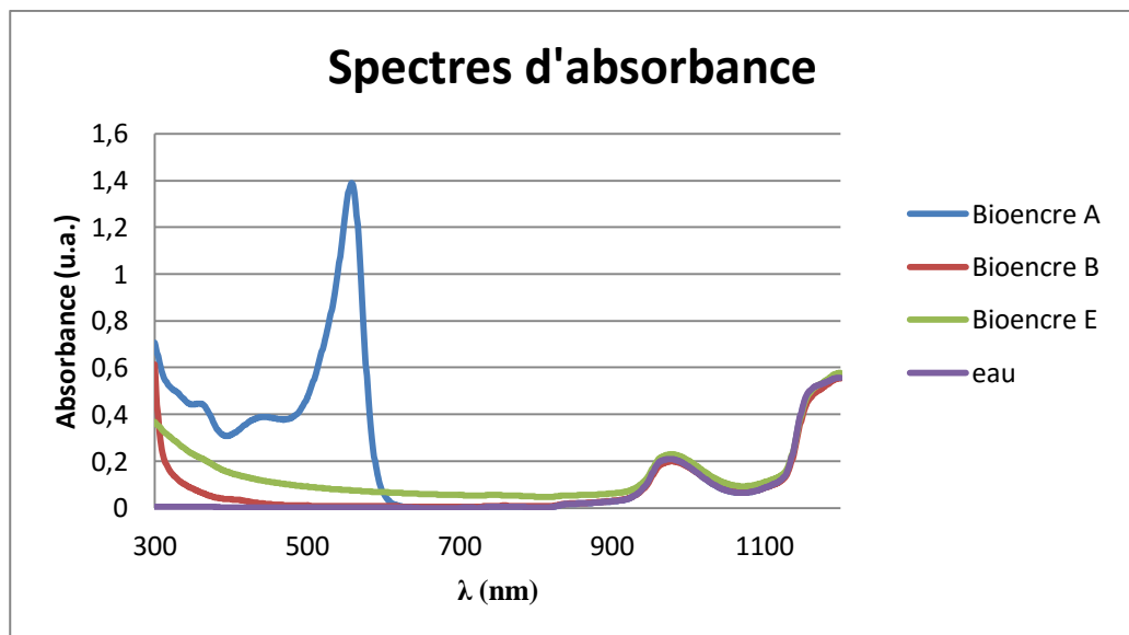
Figure 46 : Spectres d'absorbance pour les bioencres de la bioimpression sans couche absorbante (pour 1 cm d'épaisseur traversée).
