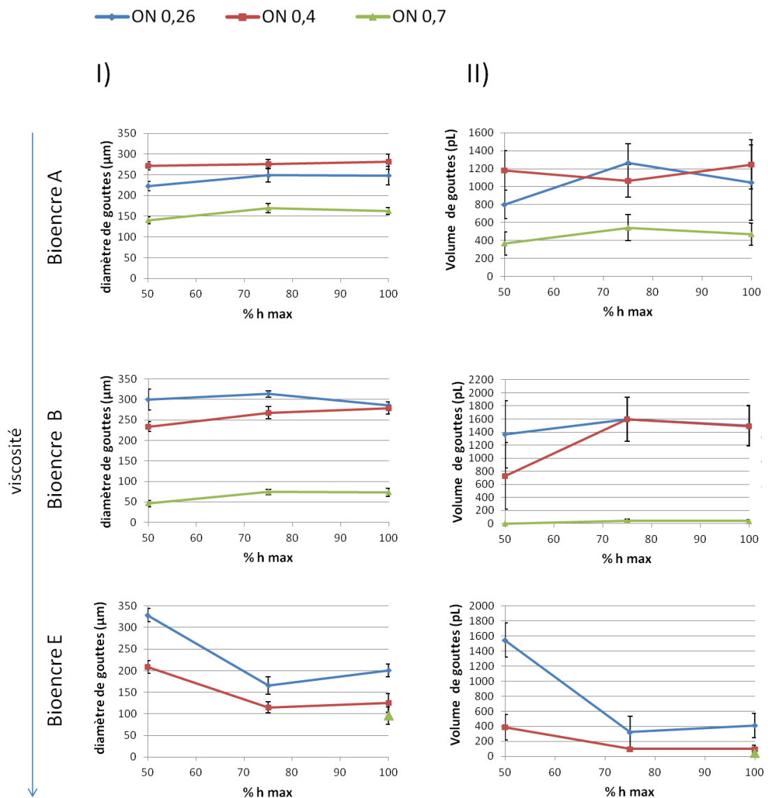
Figure 51 : Pour les bioencres A, B et E à 10 µJ : I) Diamètre de gouttes imprimées en fonction de la distance donneur-receveur. II) Volume de gouttes imprimées en fonction de la distance donneur-receveur. La distance donneur-receveur a été variée en fonction du pourcentage de la hauteur maximale ( h_{max} ) correspondant à une condition expérimentale.
