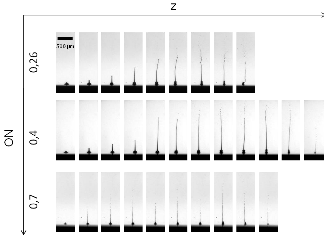
Figure 60 : Images résolues en temps du jet induit par laser lors de la variation de la position de focalisation laser pour la bioencre E et une Ouverture Numérique (ON) de 0,26 à 0,7. Les images sont prises 30 μs après l'arrivée de l'impulsion laser, à 8 μJ et entre 2 images successives la position de l'objectif de focalisation varie de 10 μm.
