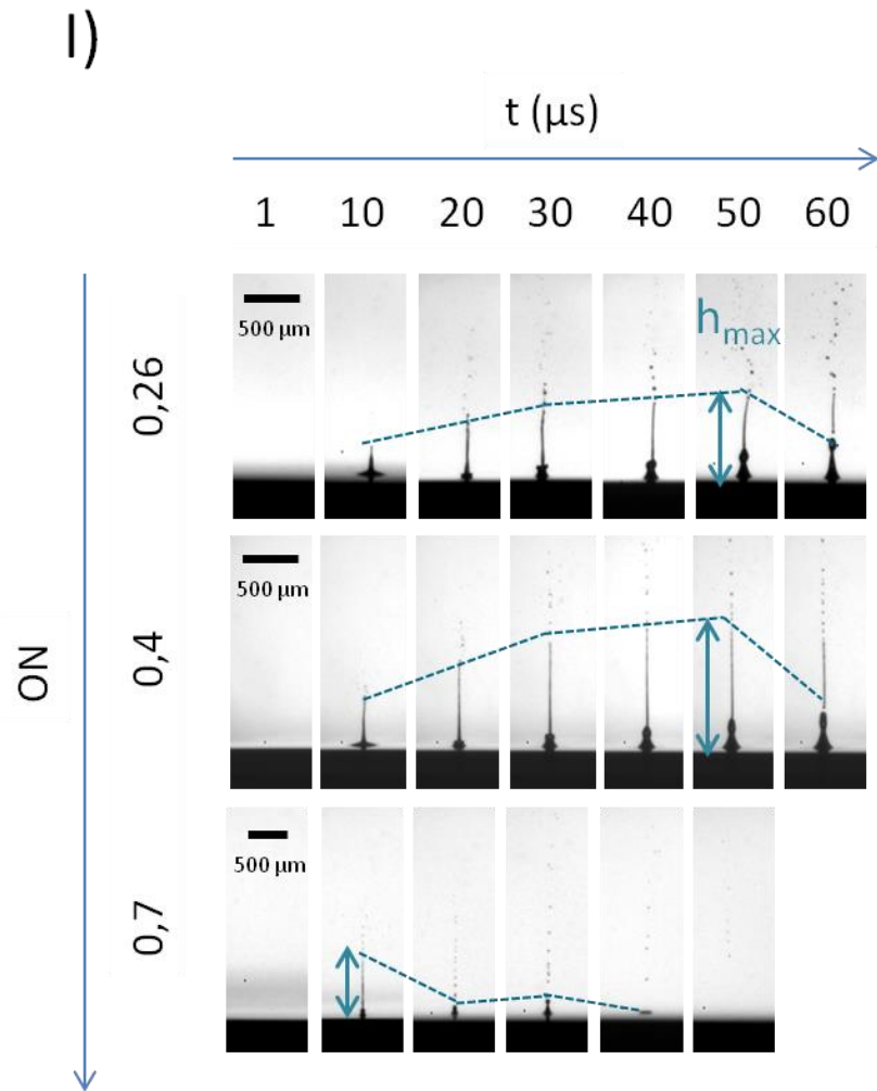
Figure 47: I) Images résolues en temps de l'évolution temporelle du jet induit par laser à 10 \mu\text{J} pour la bioencre A et une Ouverture Numérique (ON) de 0,26 à 0,7. II) Hauteur du jet mesurée sur les images de I) en fonction du temps.
