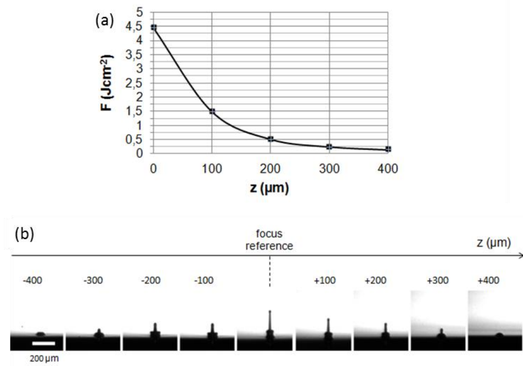
Figure 43 : Schéma de la variation de la position de focalisation laser pour la bioimpression avec couche absorbante.
