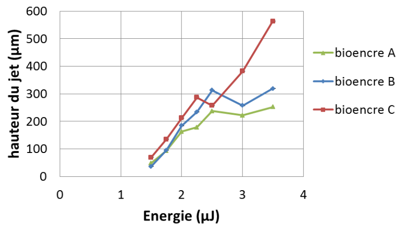
Figure 40 : Hauteur des jets en fonction de l'Énergie, 90 \mu\text{s} après l'impulsion laser, pour les bioencres A, B et C.
