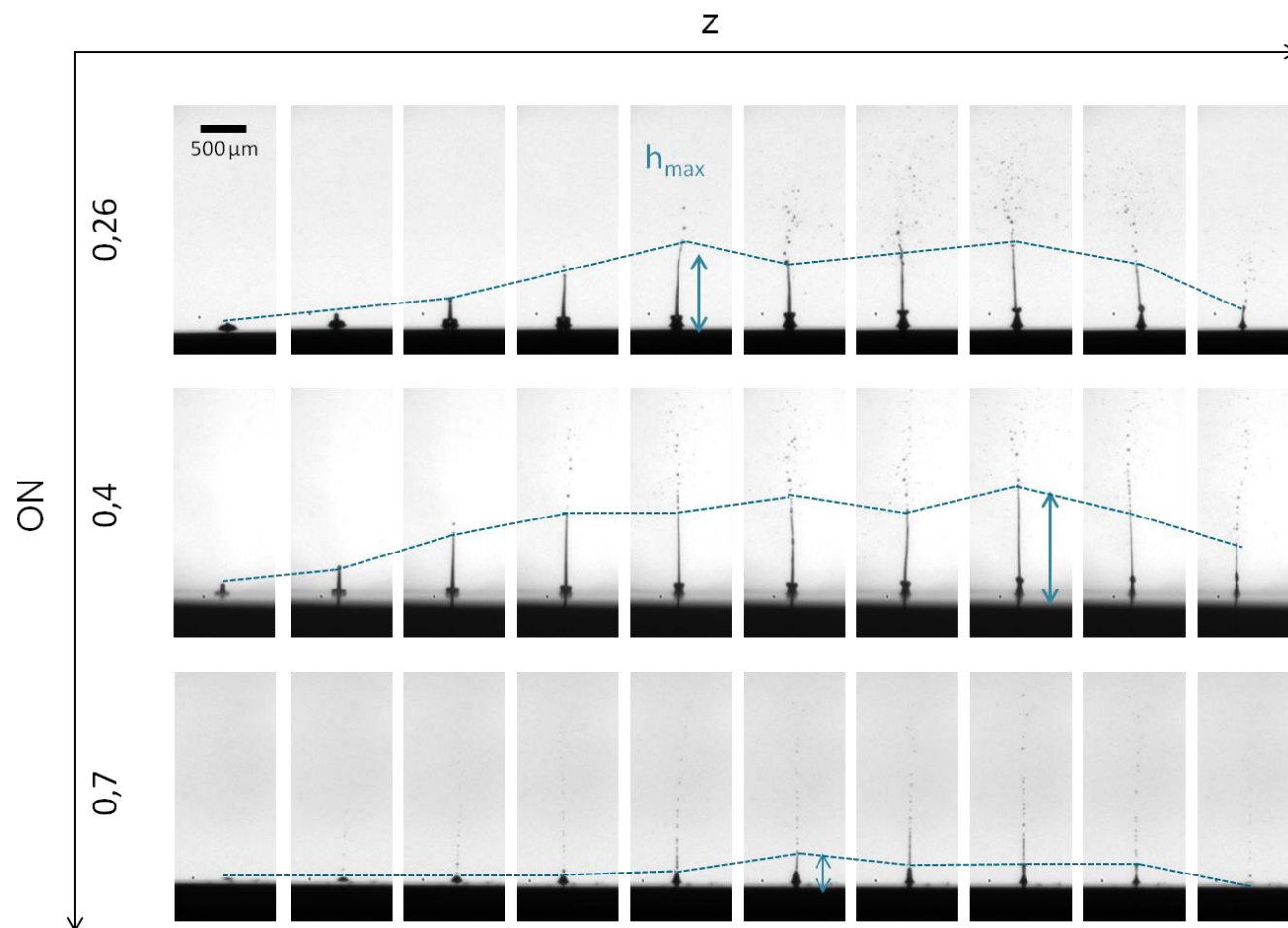
Figure 58 : Images résolues en temps du jet induit par laser lors de la variation de la position de focalisation laser pour la bioencre A et une Ouverture Numérique (ON) de 0,26 à 0,7 (données extraites de [12]). Les images sont prises 30 μs après l'arrivée de l'impulsion laser, à 8 μJ et entre 2 images successives la position de l'objectif de focalisation varie de 10 μm.
