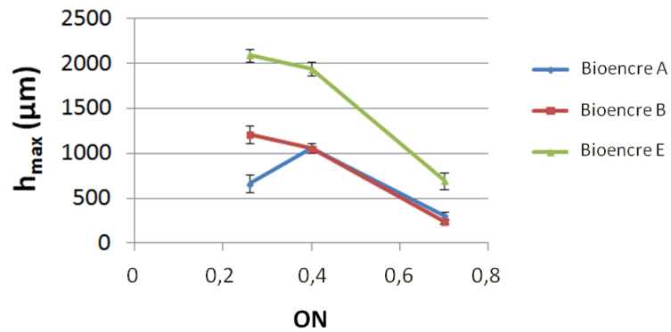
Figure 52 : Influence de l'Ouverture Numérique (ON) sur le jet de la bioimpression pour une énergie laser de 10\mu\text{J} . La hauteur maximale du jet h_{\text{max}} est donnée en fonction de l'ON pour les bioencres A, B et E (extrait de [11]).
