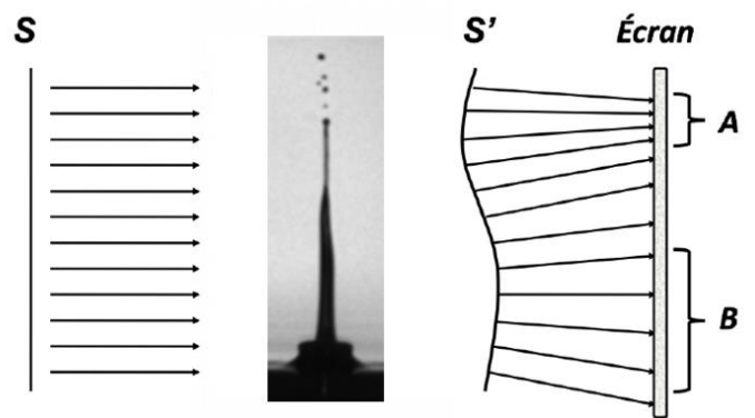
Figure 28 : Principe de l'ombroscopie.
