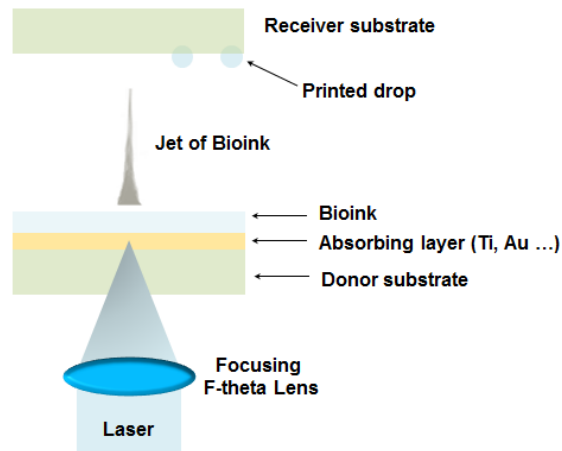
Figure 25 : Schéma de la bioimpression avec couche absorbante.
