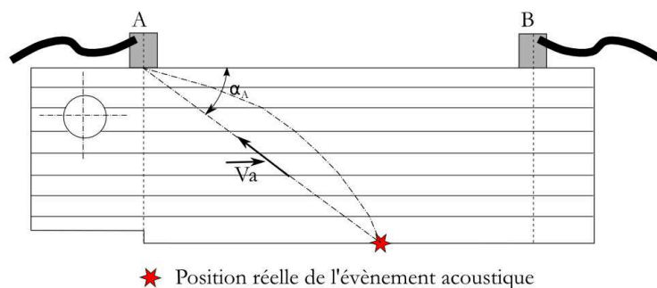
FIGURE 2.49: Cheminement supposé linéaire dans le cas de la localisation et cheminement réel dû à la diffraction.
