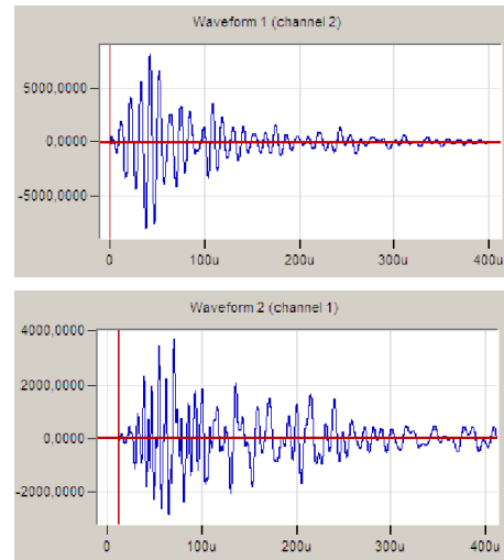
(b) Formes d'ondes enregistrées pour différents cassés de mine
