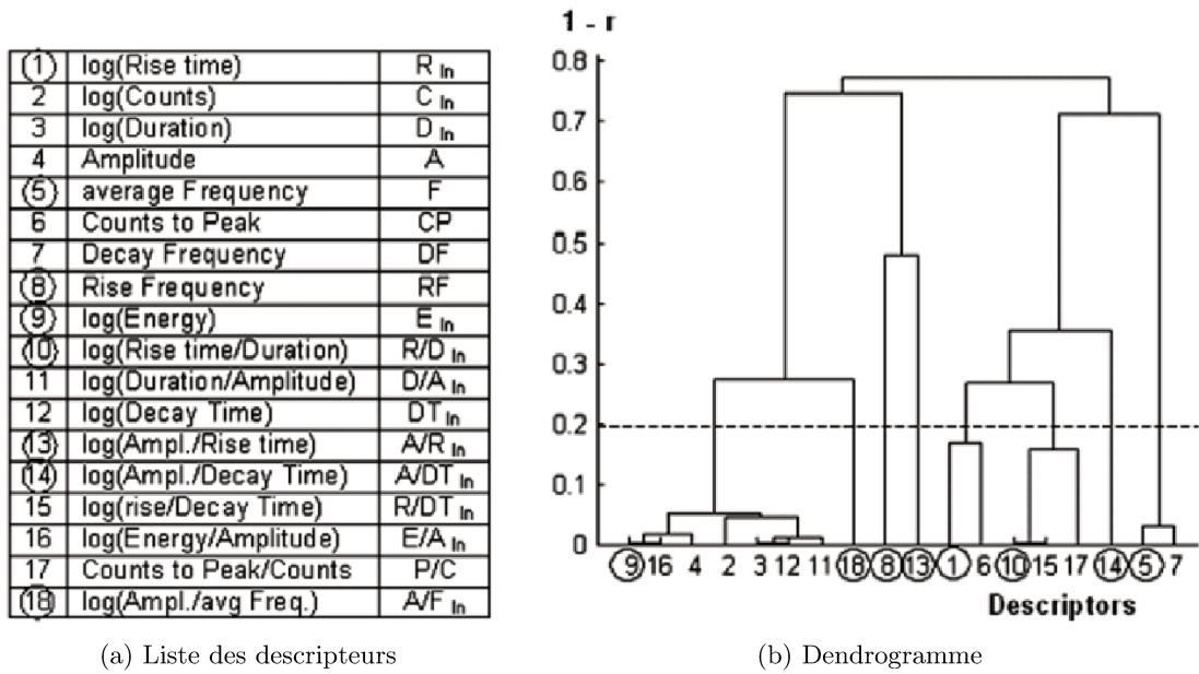
FIGURE 1.42: Dendrogramme de corrélation des descripteurs
