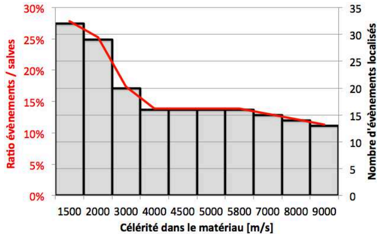
FIGURE 2.34: Effets de la vitesse effective sur la détection du nombre d'évènements pour l'aluminium
