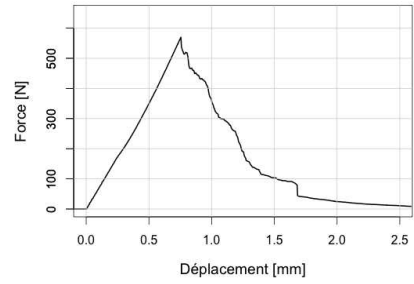
(d) Courbe force-déplacement
