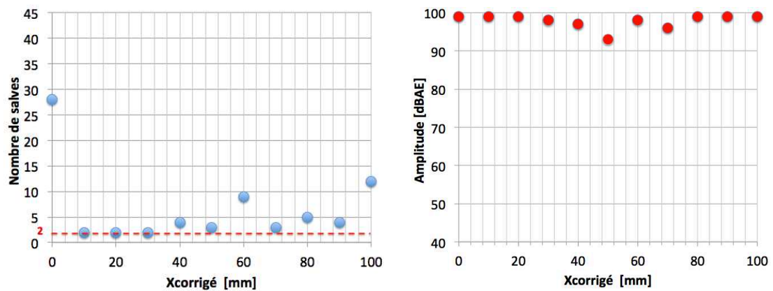
(a) Nombre de salves enregistrées pour chaque source pour une vitesse effective de 2200 [m/s] (b) Amplitude des évènements localisés pour une vitesse effective de 2200 [m/s]
