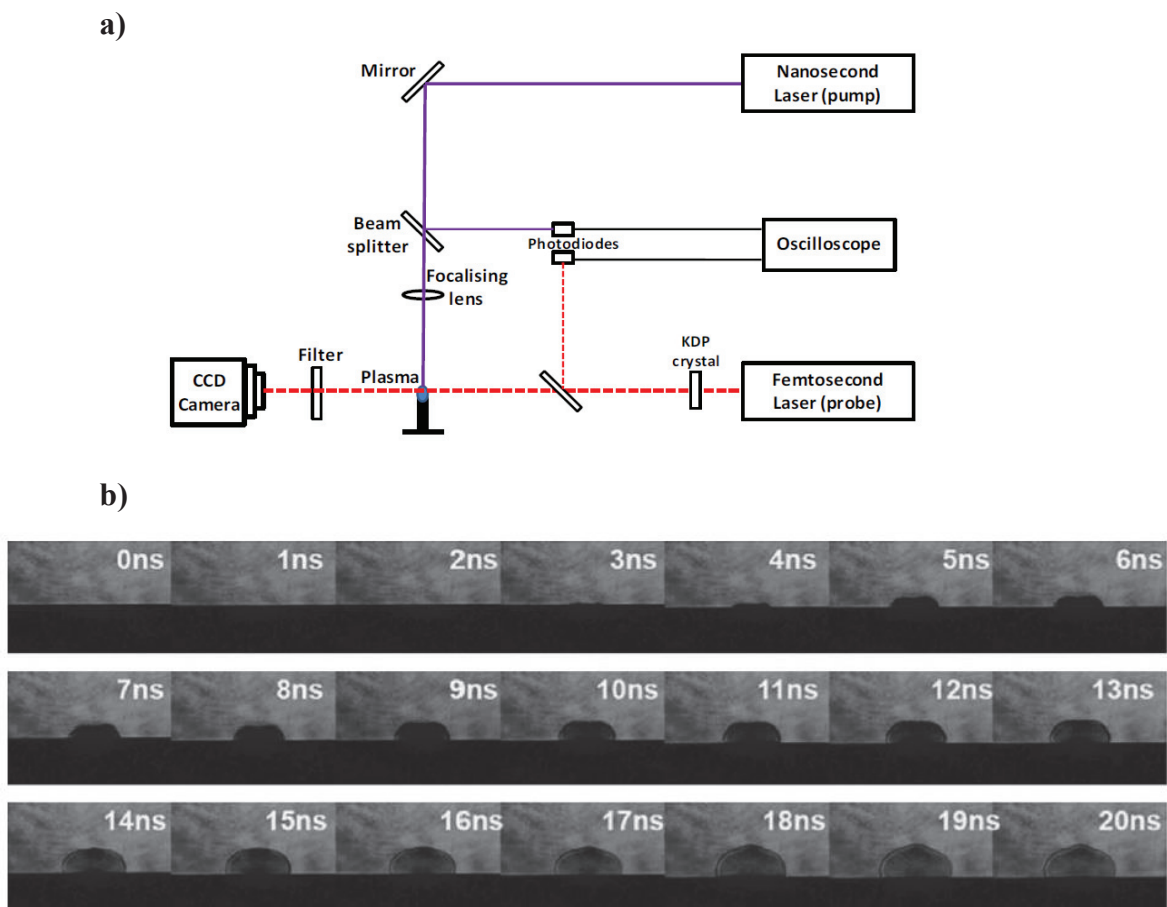
Figure 3.1 a) Exemple de montage expérimental d'ombroscopie et b) d'images de plasma obtenues par ce type de montage. Le montage est issu de [183] et les images de [184].
