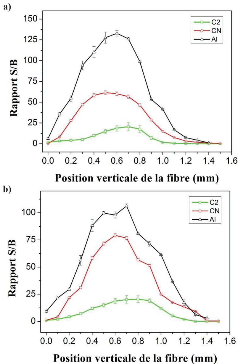
Figure 2.17 Evolution du rapport signal sur bruit en fonction de la position de la fibre de détection latérale reliée à un spectromètre a) Czerny-Turner et b) Echelle. Les intensités de la raie Al (305 nm) d'un échantillon d'Aluminium et des molécules C2 (512 nm) et CN (388 nm) d'un échantillon polymère PE ont été étudiées.
