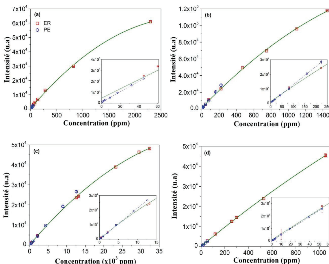
Figure 2.25 Intensités mesurées sur les échantillons « réels » ER (carrés rouges) et les perles (ronds bleus). Pour chaque élément, a) Ti, b) Cr, c)Ca et d) Ba, la courbe verte représente la modélisation quadratique de la courbe d'étalonnage des échantillons ER et la droite en pointillés bleus celle de la modélisation linéaire de l'étalonnage des perles PE. Un agrandissement de la zone correspondant aux basses concentrations est également visible.
