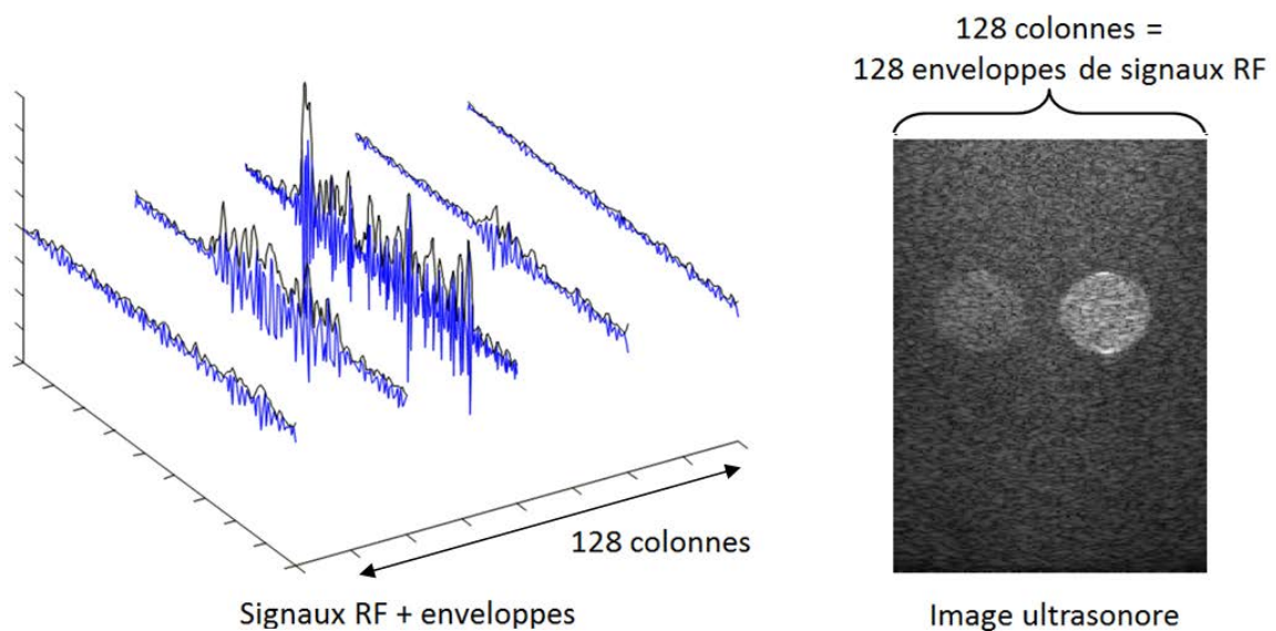
FIGURE 1.18 – Détection des enveloppes des signaux. Source : H.Liebgott
