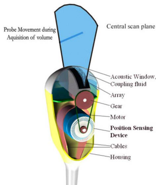
FIGURE 1.22 – Balayage automatisé d'une sonde 2D. Source : gehealthcare.com.
