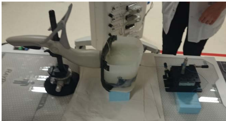
FIGURE 6.14 – Sonde US-TP au contact du fantôme dans lequel se trouve la prostate reliée à la plateforme mobile par un fil métallique.
