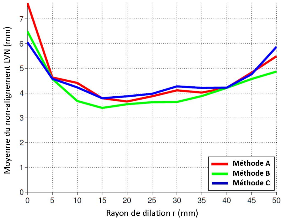
FIGURE 5.3 – Longueur moyenne des vecteurs de non-alignement LVN en fonction du rayon de dilation r et de la méthode de pré-traitement des images. Les résultats sont présentés par une ligne rouge, verte et bleue pour les méthodes A, B et C, respectivement.
