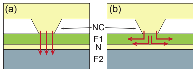
Figure I.21 – Extrait de [37]. On peut séparé le courant traversant l'échantillon en deux composantes; a) le courant CPP qui le traverse perpendiculairement au plan des couche et (b) le courant CIP qui le traverse parallèlement.
