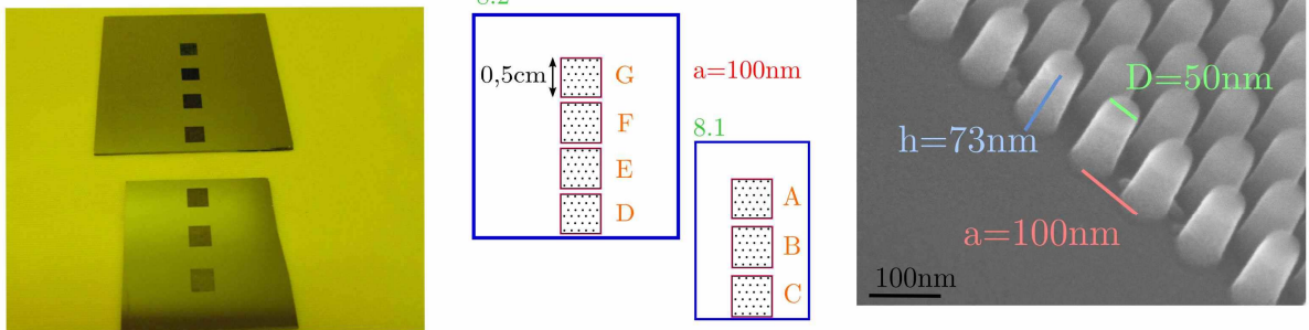
Figure 16 : Les différents moules de nano-impression réalisés au laboratoire, photographie, schémas, et Image MEB, des moules a) n°5, b) n°7, c) n°8.
