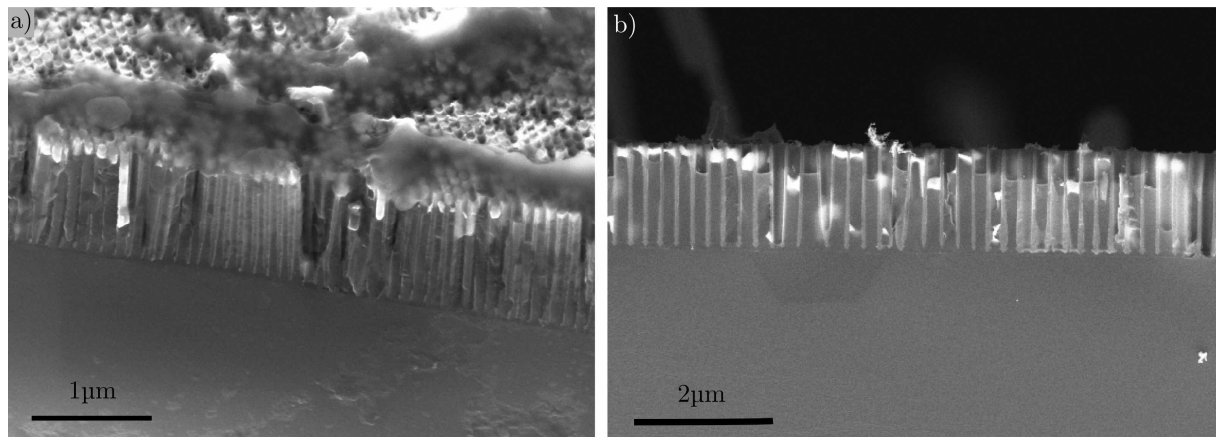
Figure 71 : Image MEB de réseau de fils de silicium crûs dans l'alumine super-organisée, a) période 100 nm diamètre 70 nm et hauteur environ 1400 nm, b) période 250 nm, diamètres 180 nm et hauteur 1280 nm.
