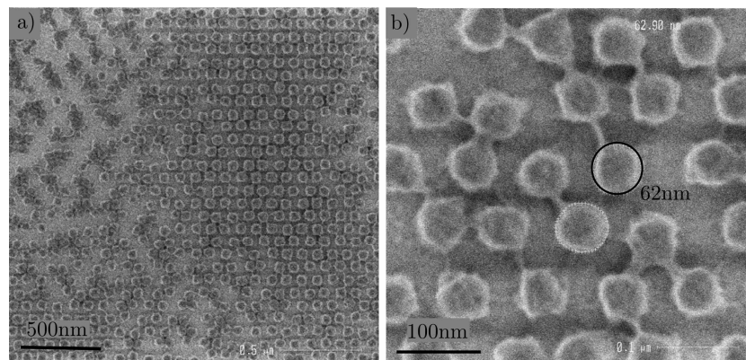
Figure 17 : Image MEB de la résine après développement des tests de moules de diamètres de plots de 30 nm, a) vue d'ensemble, b) zoom sur une zone avec des plots (zone surexposée donnant des plots plus grands que ceux visés).
