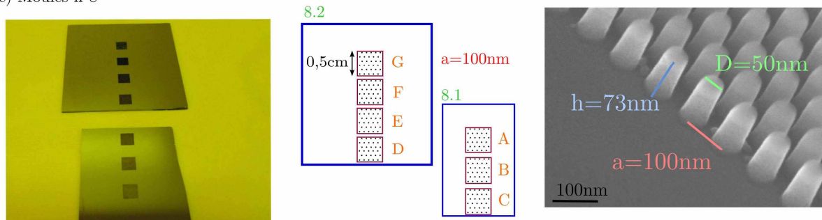
Figure 16 : Les différents moules de nano-impression réalisés au laboratoire, photographie, schémas, et Image MEB, des moules a) n°5, b) n°7, c) n°8.
