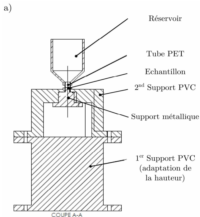
Figure 54 : Cellule électrochimique adaptée aux mesures GISAXS, a) schéma technique, b) photographie de la cellule sur la ligne SIXS.
