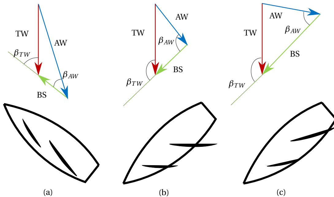
Figure E.1 – Triangles de vitesses pour différentes configurations. (a) au près (b) au portant (c) au portant avec un bateau plus rapide. TW: True wind, vent réel. AW: Apparent wind, vent apparent. BS: Boat Speed, vitesse du bateau.
