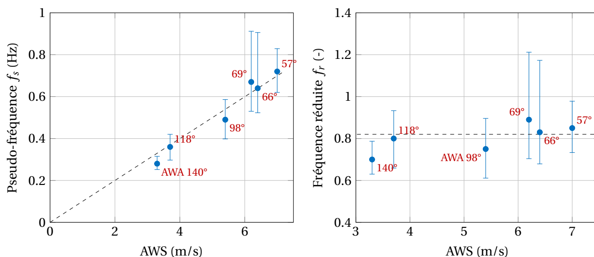
Figure E.18 – Pseudo-fréquence f_s (gauche) et fréquence réduite f_r (droite) du faseyement du spinnaker pour différents angles de vent apparents (AWA) en fonction de la vitesse du vent apparent (AWS). Une interpolation linéaire passe par les points expérimentaux.
