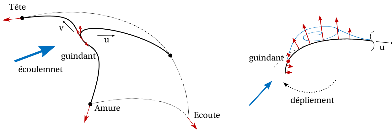
(a) Pendant le déplieement ( entre les instants C et D ). Du fait d'un important gradient de pression au guindant, la corde "écoulemnet" u se déplie. La taille de la bulle de séparation au bord d'attaque augmente.
