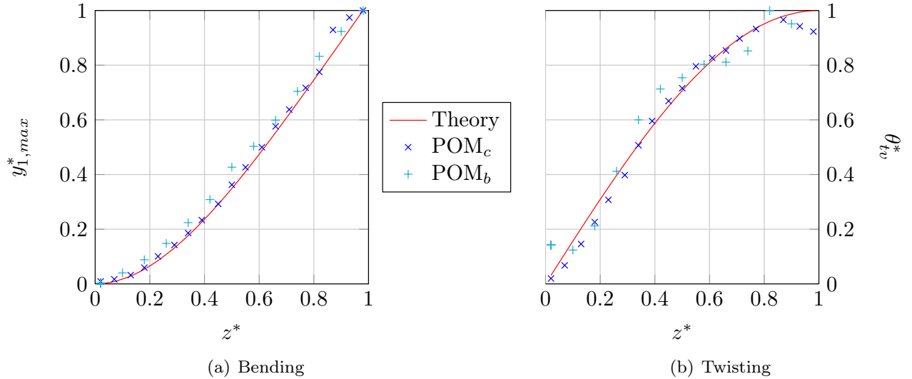
FIGURE 3.4 – Formes modales des profils POM_c et POM_b en écoulement, \alpha = 8^\circ et U = 6 \text{ m.s}^{-1} , comparées à la théorie des poutres
