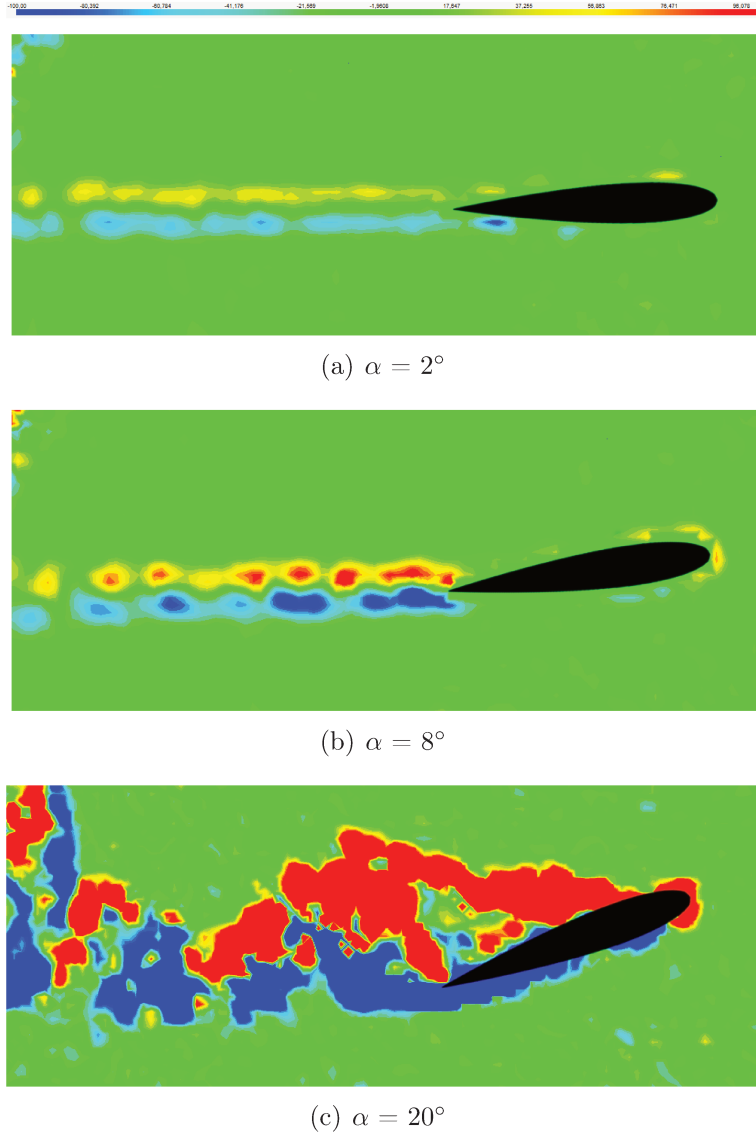
FIGURE 3.50 – Champs de vorticité expérimentaux autour du profil POM c ( Re = 5.10^5 )
