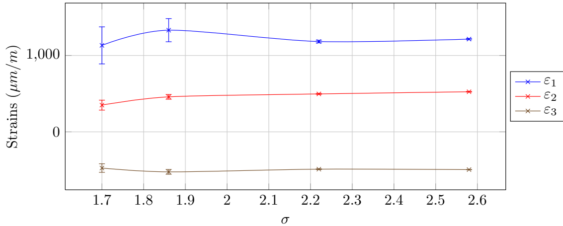
FIGURE 4.1 – Déformations moyennes mesurées sur le profil \text{POM}_c en fonction du nombre de cavitation. Les barres verticales représentent l'écart type
