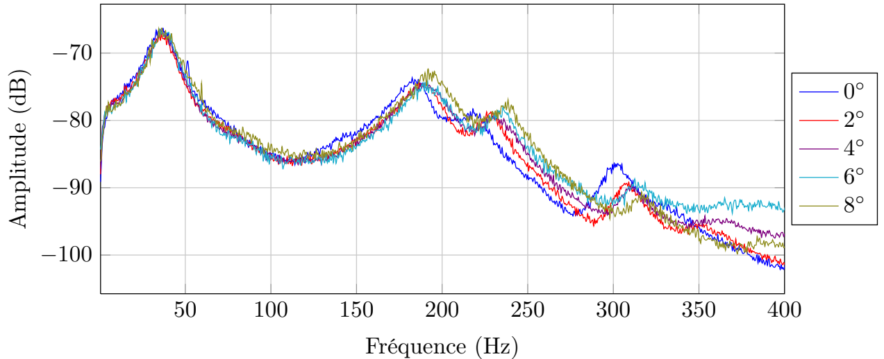
FIGURE 3.33 – Réponse vibratoire du profil POM c en écoulement, U = 6 \text{ m.s}^{-1} ( \text{Re} = 6.10^5 )
