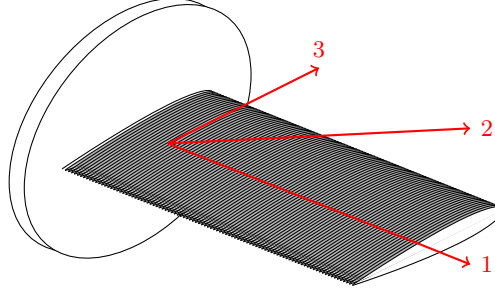
FIGURE 2.14 – Axes des jauges de contraintes du profil en POM
