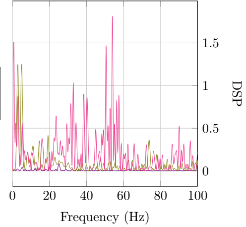
FFT des signaux de la caméra rapide ( x^* = 0,2 )
