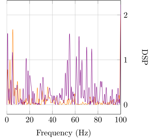
FFT des signaux de la caméra rapide ( x_v^* = 0,2 )
