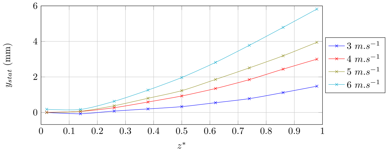
FIGURE 3.36 – Déformées statiques (flèche) du profil POM c en écoulement, \alpha = 8^\circ
