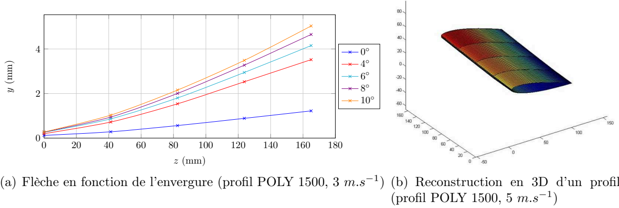
FIGURE 2.20 – Exemple de données obtenues grâce au télémètre laser
