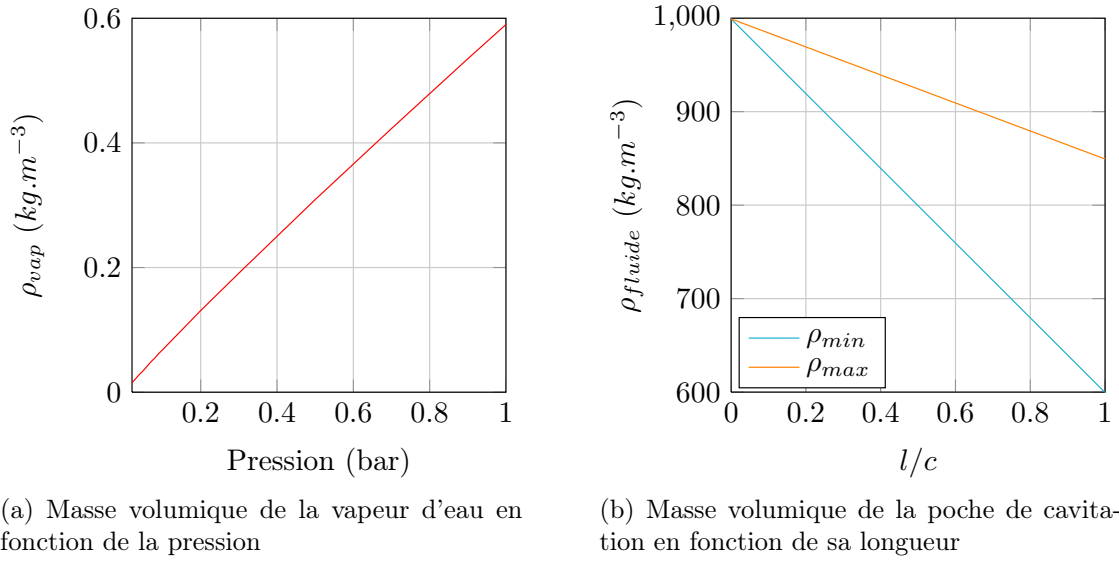
FIGURE 4.16 – Détermination de la masse volumique de la poche de cavitation
