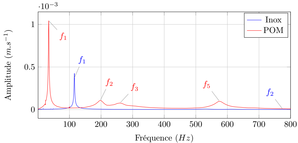
FIGURE 2.30 – Spectres des profils en acier inoxydable et POM c en réponse à une impulsion en eau
