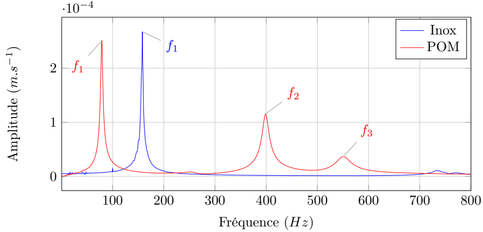
FIGURE 2.29 – Spectres des profils en acier inoxydable et POM c en réponse à une impulsion en air
