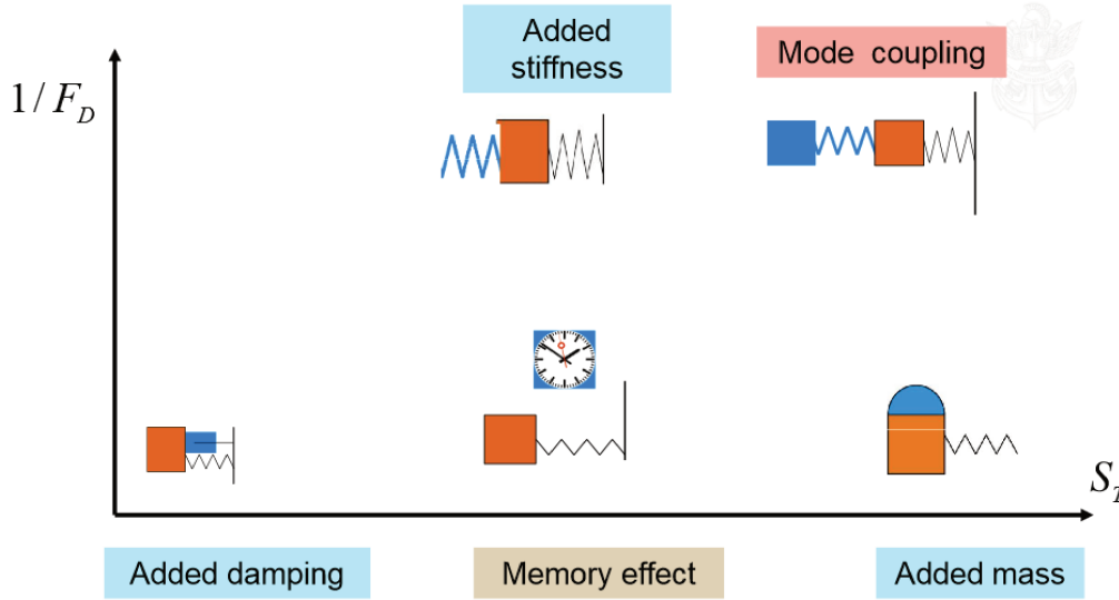
FIGURE 1.1 – Couplages mis en évidence entre un fluide et un solide par de Langre [36]. L'effet du fluide est modélisé en bleu : en fonction des grandeurs caractéristiques de l'écoulement, il peut être modélisé par un amortissement, une raideur ou une masse ajoutées au solide. Ce cas est développé au chapitre 1.5.
