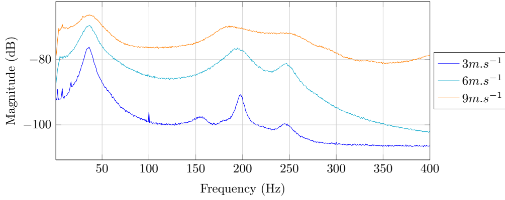
FIGURE 3.2 – Réponse vibratoire moyennée sur toute la surface du profil POM_c en écoulement, \alpha = 8^\circ
