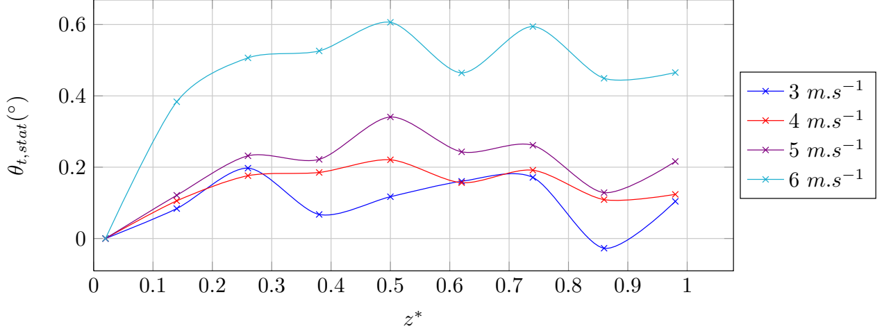
FIGURE 3.35 – Déformées statiques (torsion) du profil POM c en écoulement, \alpha = 8^\circ
