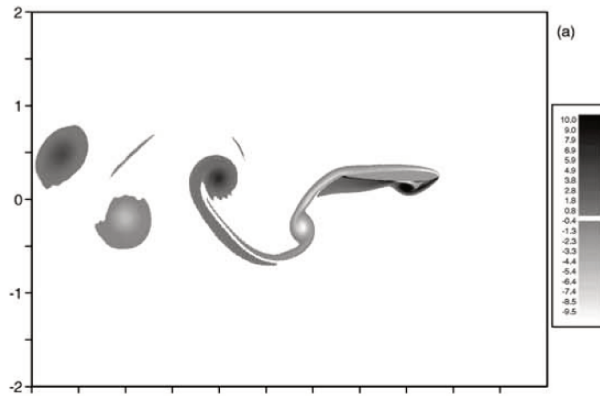
FIGURE 1.3 – Champs de vorticit  derri re un profil en tangage et pilonnement, Re = 1100 , par Guglielmini et Blondeaux [57]
