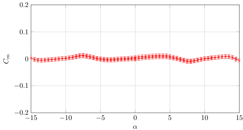
FIGURE 3.13 – Coefficient de moment C_m expérimental du profil POM b en fonction de l'incidence \alpha avec U = 5 \text{ m.s}^{-1} . Les barres d'erreur correspondent à l'incertitude sur les mesures
