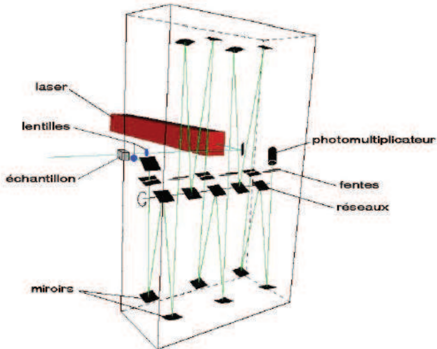
FIGURE 3.1 – Trajet optique dans le quintuple monochromateur Dilor Z40 [26]
