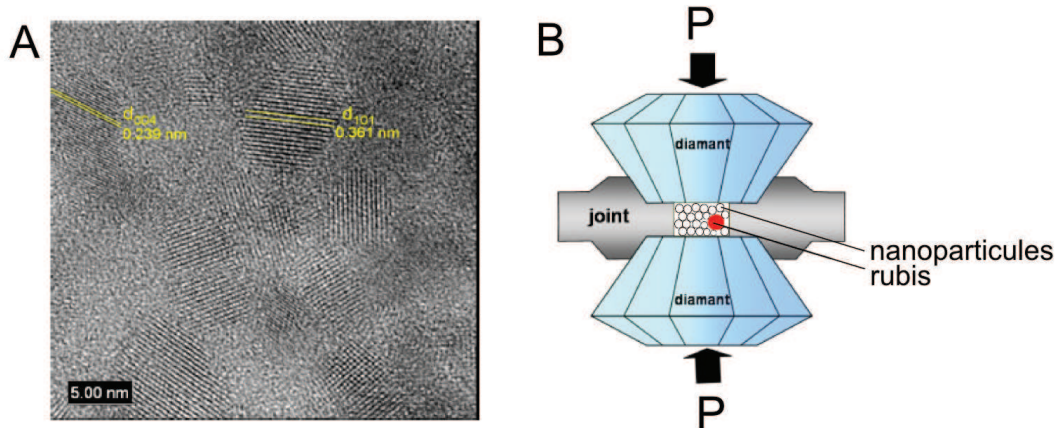
FIGURE 6.3 – A. Image MET haute résolution de la poudre HT7 montrant des nanoparticules de TiO 2 de diamètre moyen D=3.6 \text{ nm} [100]. B. Représentation schématique d'un chargement de poudres en CED (pas à l'échelle)
