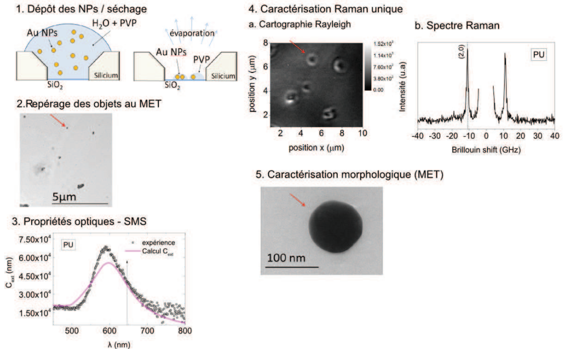
FIGURE 5.2 – Résumé de l'ensemble des cinq étapes du protocole expérimental pour la caractérisation Raman - SMS d'un nano-objet unique (ici une nanoparticule d'or unique marquée par une flèche rouge).
