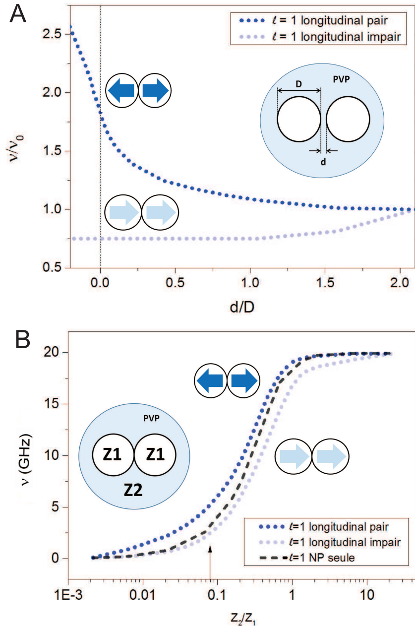
FIGURE 5.7 – A. Calcul des fréquences des modes dipolaires longitudinaux symétriques et anti-symétriques d'un dimère en matrice (PVP) de nanoparticules d'or de diamètre D en fonction de la séparation normalisée d/D . Les fréquences sont normalisées à la fréquence \nu_0 du mode dipolaire d'une sphère seule en matrice. B. Calcul des fréquences des modes dipolaires longitudinaux symétriques et anti-symétriques d'un dimère d'or en matrice de PVP ( D_1 = D_2 = 100 nm, d = 0 nm) en fonction du rapport des impédances acoustiques Z_2/Z_1 ( Z_2 = matrice, Z_1 = NP). La fréquence du mode dipolaire d'une sphère seule ( D = 100 nm) est également représentée (noir). La valeur de Z_2/Z_1 correspondant aux conditions expérimentales des dimères mesurés est représentée par une flèche verticale.
