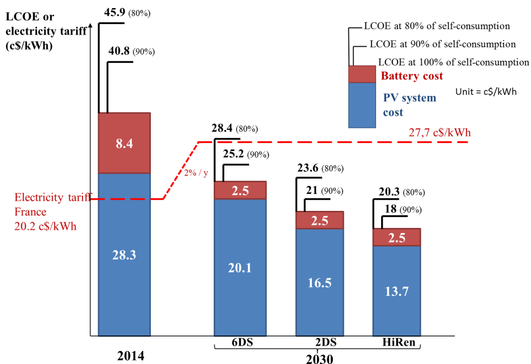
Figure 6 : Attrait économique de l'autoconsommation PV avec batterie dans le résidentiel en 2030
