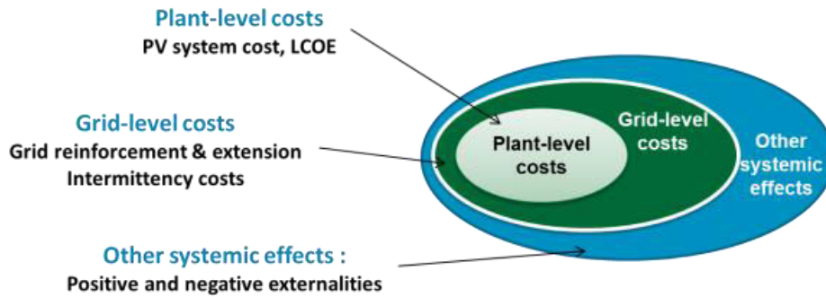
Figure 1: Coût total du système PV (OECD/NEA)
