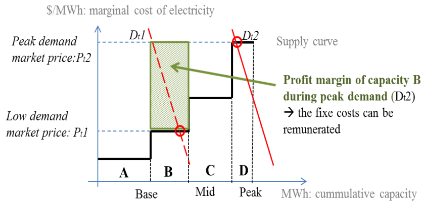
Figure 27: Merit order and electricity price formation (Haas, et al., 2013; Commissariat Général à la Stratégie et la Prospective (CGSP), 2014)
