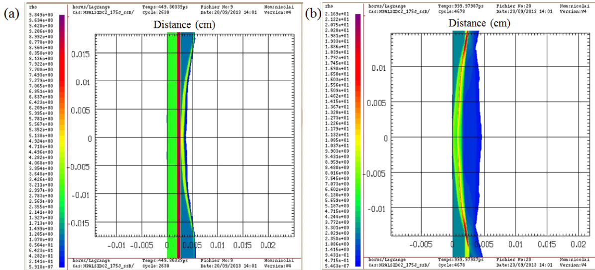
FIGURE 4.30 – Exemple de résultat d’une simulation CHIC réalisée sur une cible constituée de 25\mu\text{m} de parylène-C, 5\mu\text{m} de cuivre et 25\mu\text{m} d’aluminium avec un faisceau à 3\omega ( \lambda=0,438\text{nm} ), une énergie de 200\text{J} et une tache focale gaussienne de 100\mu\text{m} de largeur à mi-hauteur. Carte des densités à t=450\text{ps} (a) lorsque le choc arrive dans le cuivre et à t=1\text{ns} (b) lorsque le choc débouche dans le vide et que l’on commence à collecter l’émission propre du choc.
