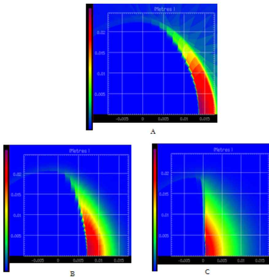
FIGURE 4.11 – Cartes des pressions dans le cas d'un tir sur une demi-sphère obtenues à l'aide de simulations 2D réalisées avec le code CHIC avec une intensité de 10^{14}\text{W}/\text{cm}^2 et une tache focale gaussienne de 400\mu\text{m} de diamètre à 1/e aux temps A :2ns, B :3,5ns et C :4,75ns. Les distances sont en centimètres et le maximum de pression vaut 23Mbar. On voit bien que dans ce cas, le choc devient plan et c'est cela que l'on veut voir expérimentalement.
