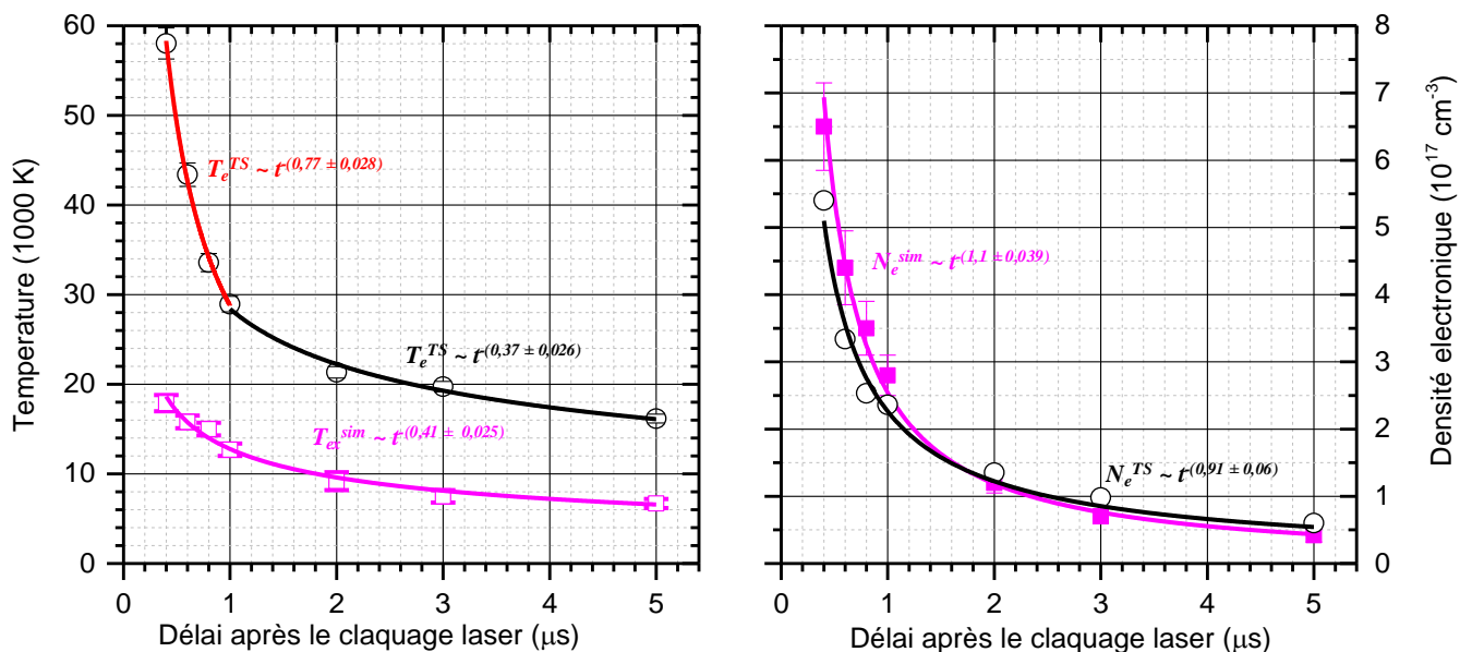
Fig. 4-24 : Evolution temporelle des densités électroniques et des températures sur l'axe du plasma ( Z = 0, Y = 0, r = 0 ) [Fluence laser plasma : 1,8 \text{kJ}/\text{cm}^2 - Fluence laser Thomson : 10 \text{J}/\text{cm}^2 ]
