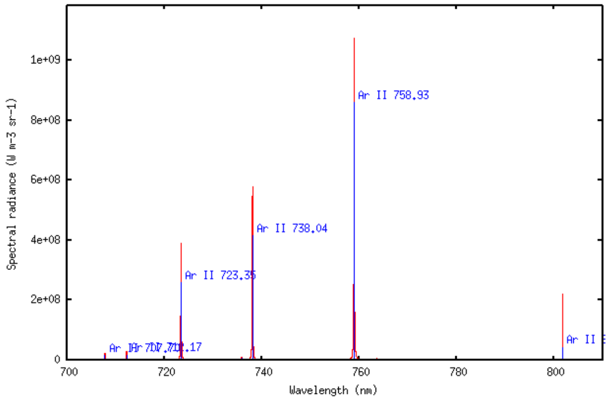
4) Spectre d'émission simulé pour T_e^{TS} = 68000 K et N_e^{TS} = 5,4 \times 10^{17} \text{ cm}^{-3}
