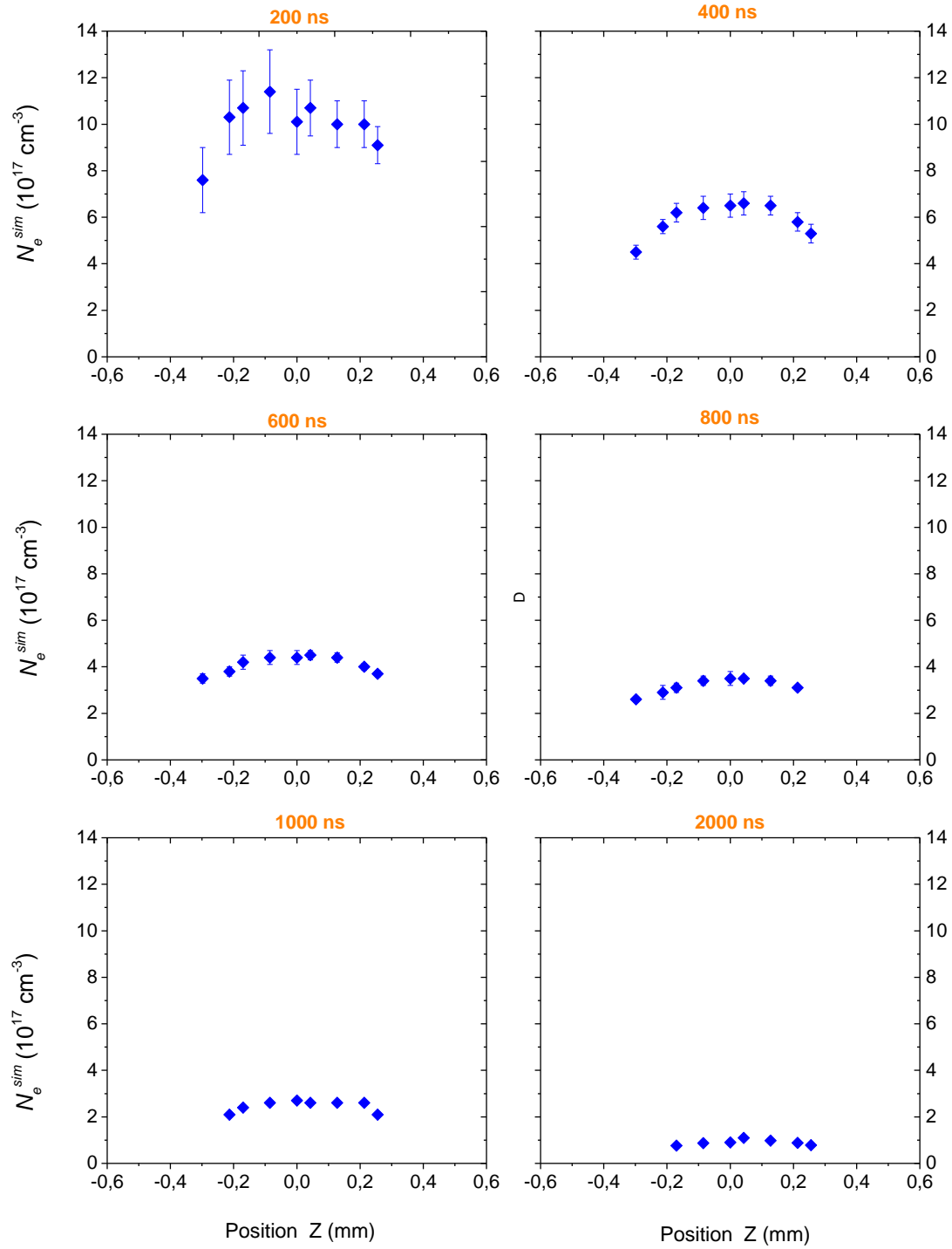
Fig. 4-18 : Distribution spatiale de N_e^{sim} à différents instants après le claquage laser ( Y = 0 ) [Fluence laser plasma : 1,8 \text{kJ}/\text{cm}^2 ]
