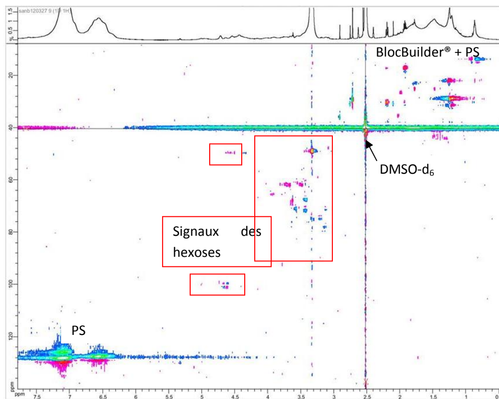
Figure 3.VII.2. Spectres RMN HSQC 2D, dans DMSO- d_6 à température ambiante, du polymère tri-bio-fonctionnalisé P_3 montrant la présence des principaux pics des hexoses
