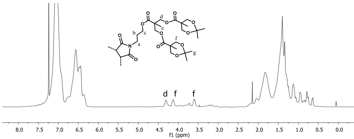
Figure 2.VIII.D.2. Spectre RMN ^1\text{H} du copolymère P(Sty-co-D2) enregistré à température ambiante dans \text{CDCl}_3 .
