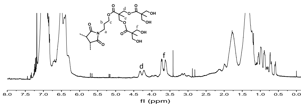
Figure 2.VIII.D.5. Spectre RMN 1 H du copolymère P(Sty-co-D5) enregistré à température ambiante dans CDCl 3 .
