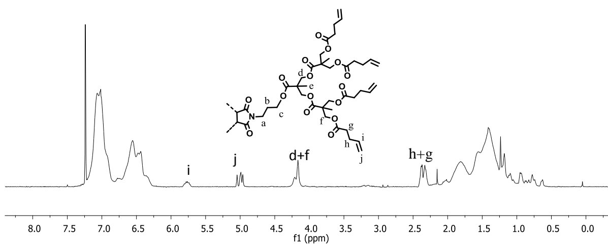
Figure 2.VIII.D.6. Spectre RMN 1 H du copolymère P(Sty-co-D6) enregistré à température ambiante dans CDCl 3 .
